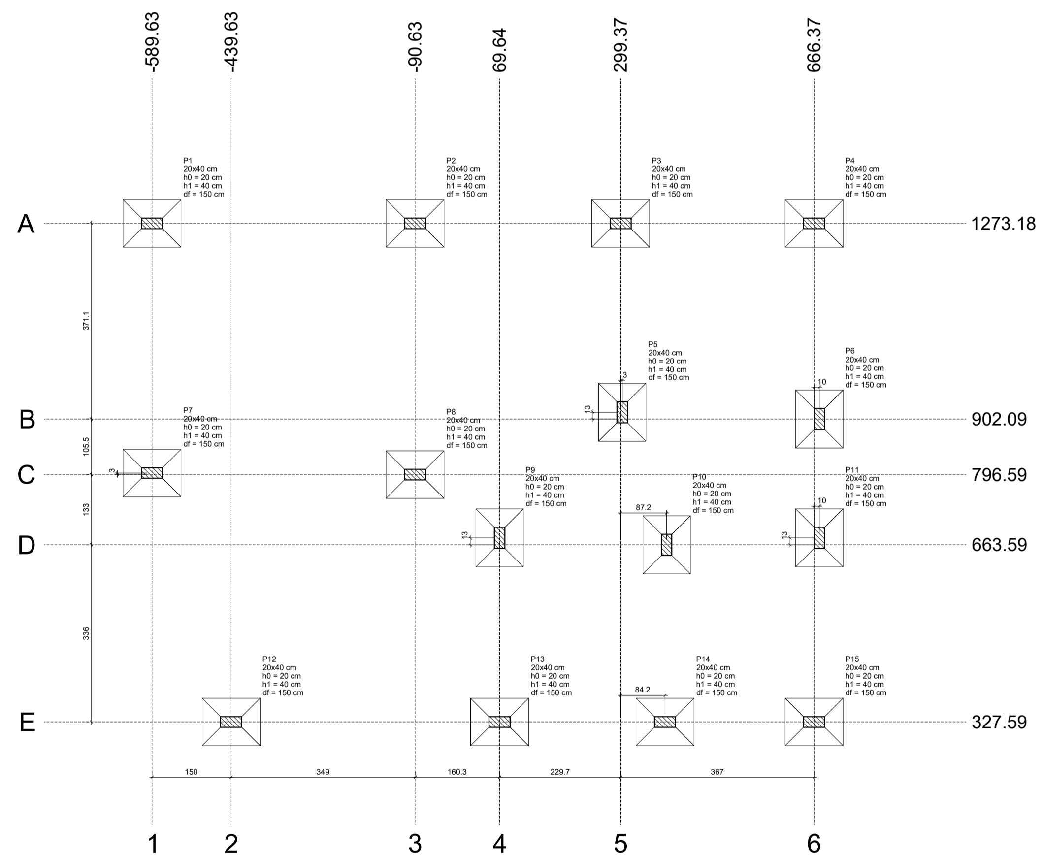
PLANTA DE LOCAÇÃO Escala 1:50
