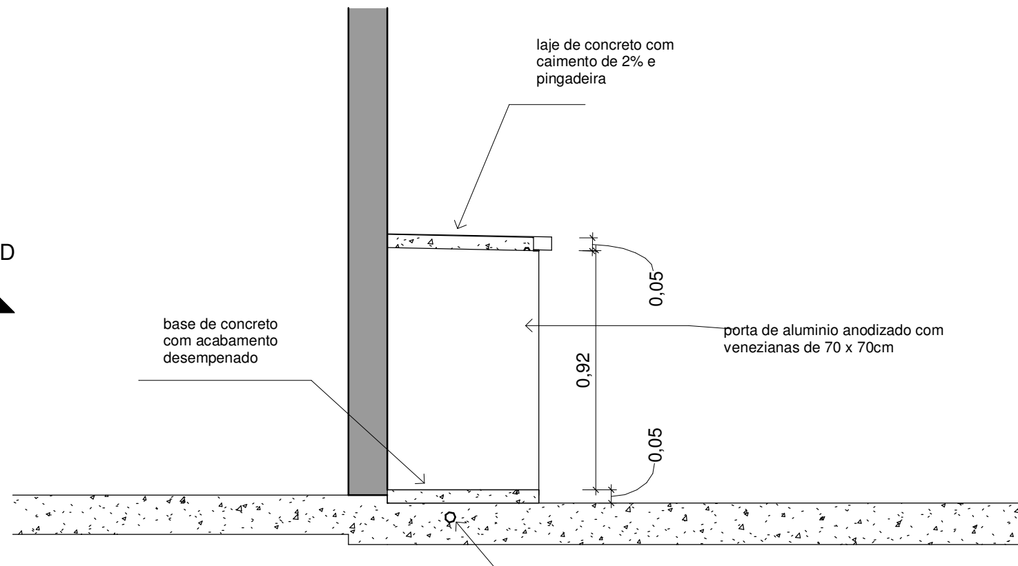
CORTE D-D - ABRIGO DE GÁS ESC:1/20
