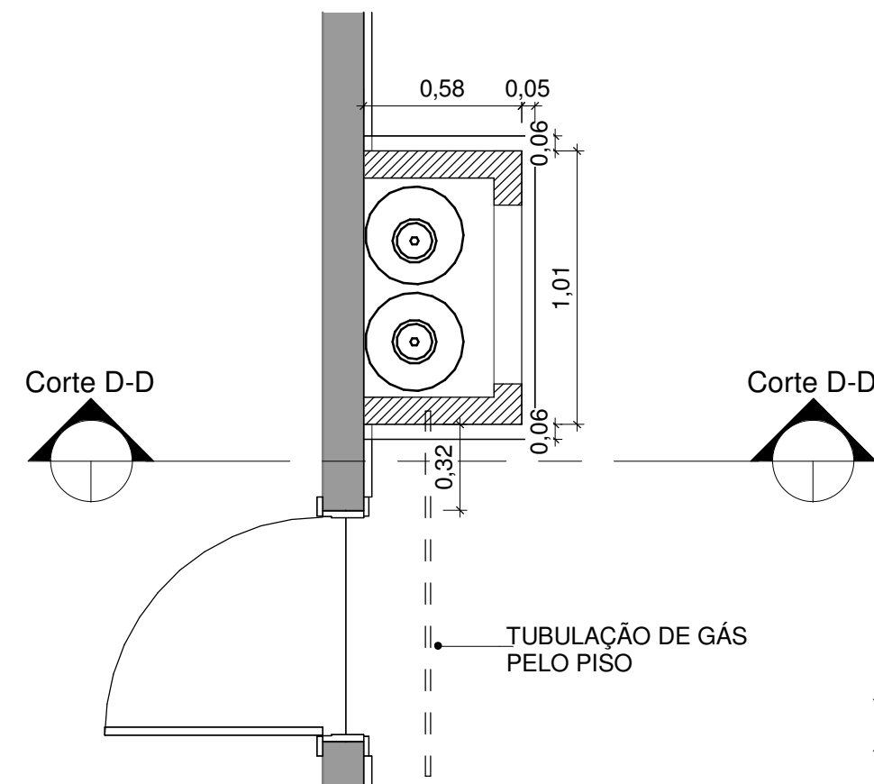
DETALHE 04 - PLANTA BAIXA ABRIGO DO GÁS ESC:1/25
