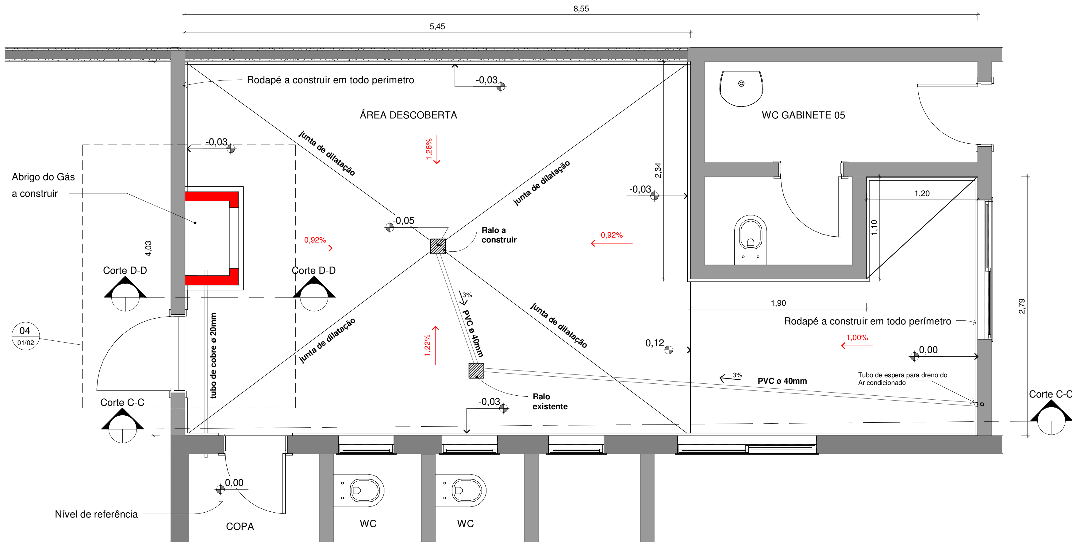
DETALHE 01 - PLANTA BAIXA DETALHE PISO DA ÁREA DESCOBERTA ESC:1/25
