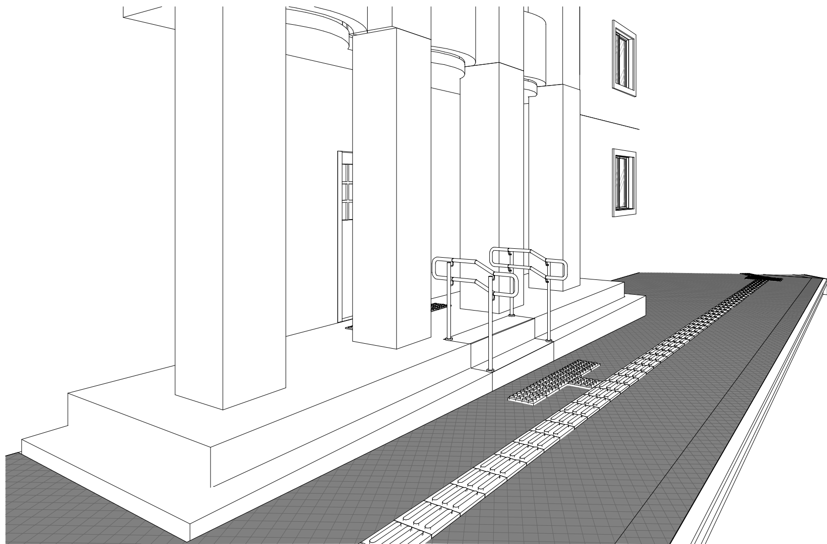
VISTA DETALHE DO CORRIMÃO ACESSÍVEL S/ESC.
