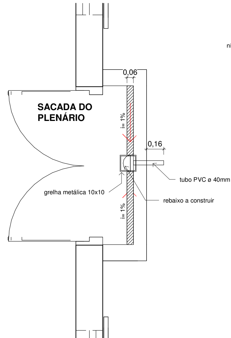
DETALHE 02 - SACADA DO PLENÁRIO ESC:1/20
