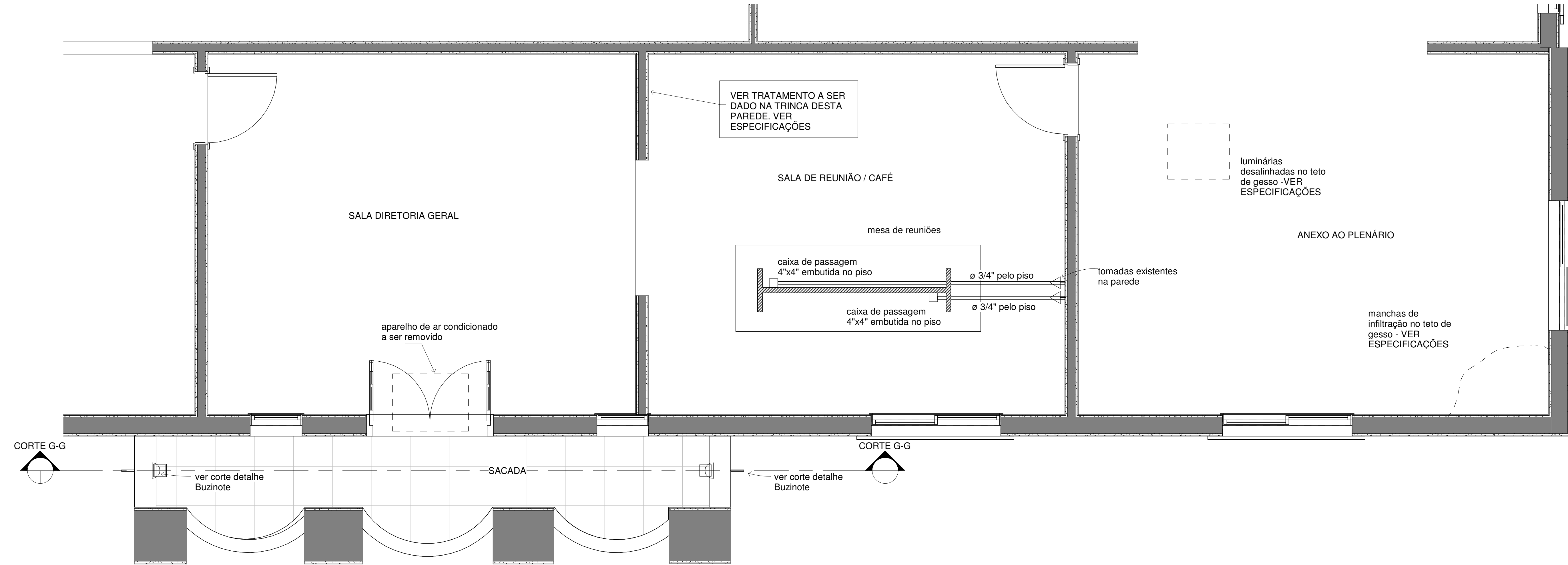
DETALHE 03 - PLANTA DETALHE SACADA DIRETORIA GERAL ESC:1/25
