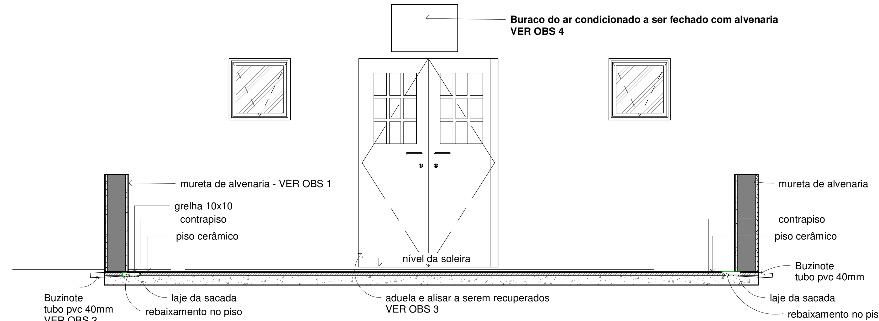
CORTE G-G - PISO DA SACADA DA SALA DIRETORIA GERAL ESC: 1/25
