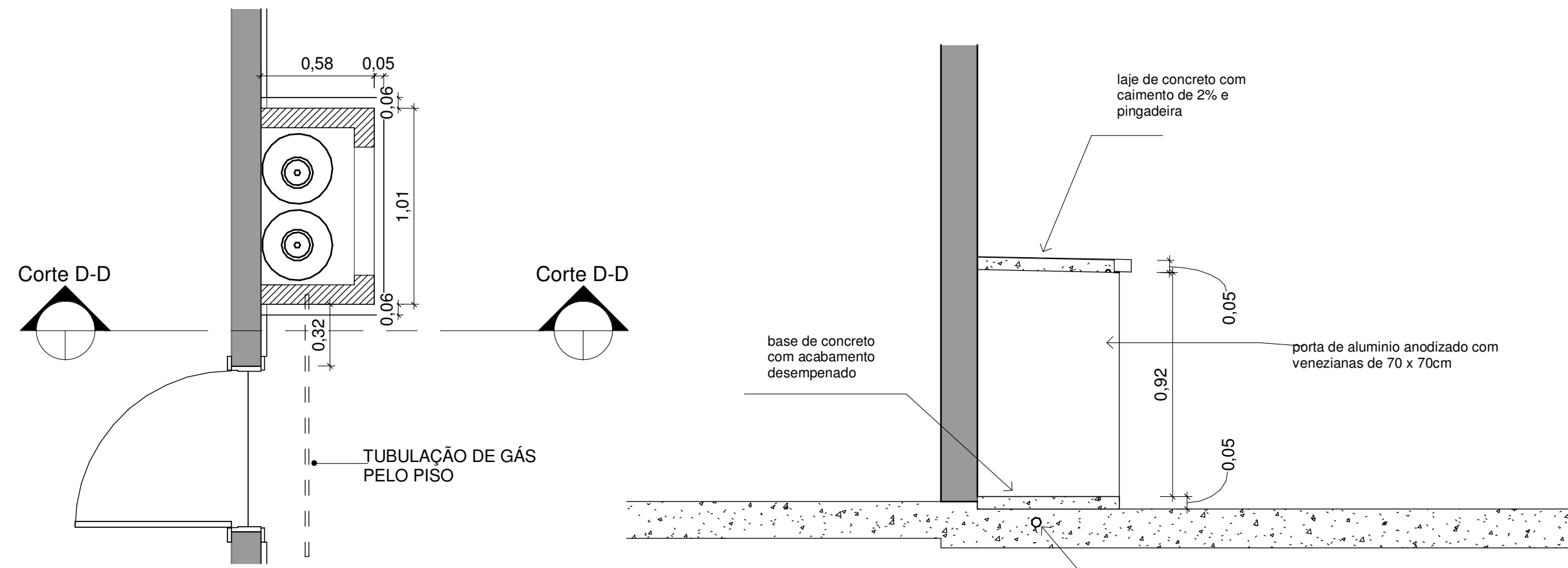
DETALHE 04 - PLANTA BAIXA ABRIGO DO GÁS ESC:1/25
