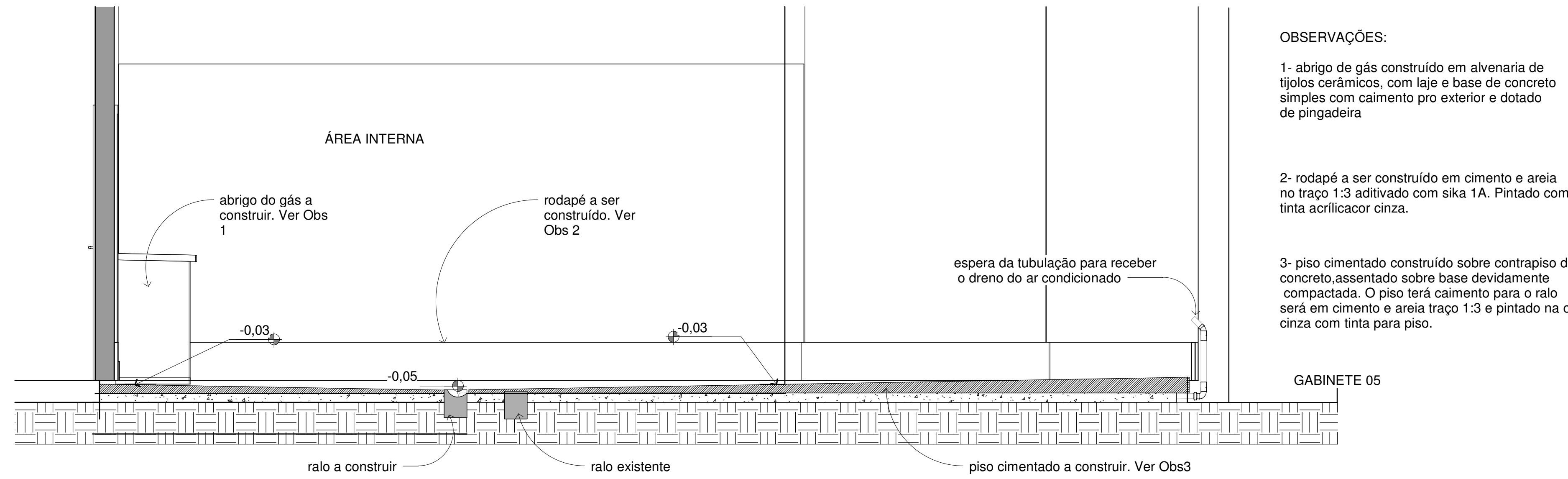
CORTE C-C - PISO DA ÁREA DESCOBERTA ESC:1/25
