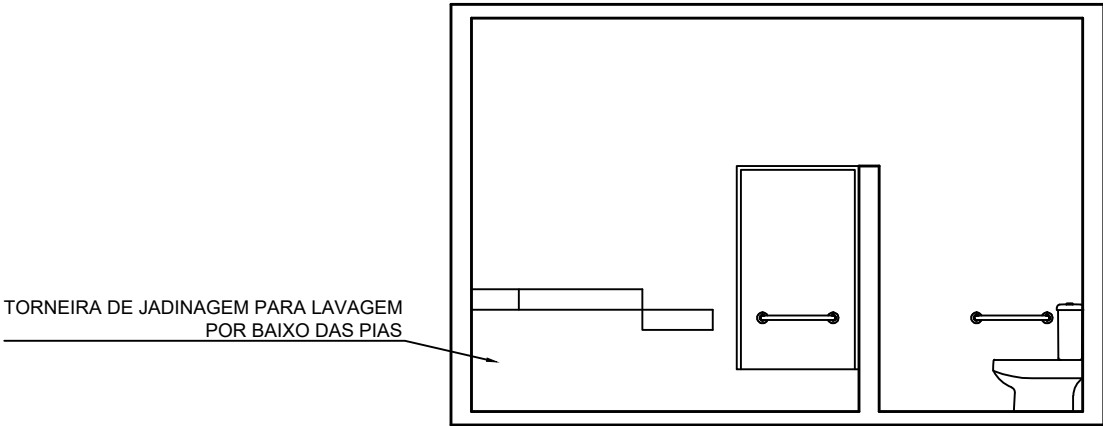
CORTE BB
