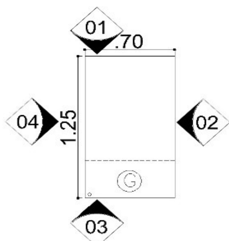
PLANTA - MESA "G" – 01 UNIDADE
