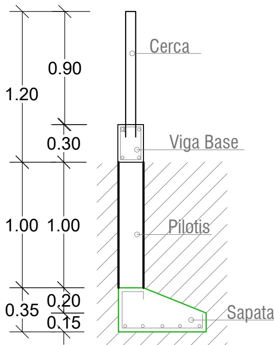
Corte AA' Escala: 1 : 30
