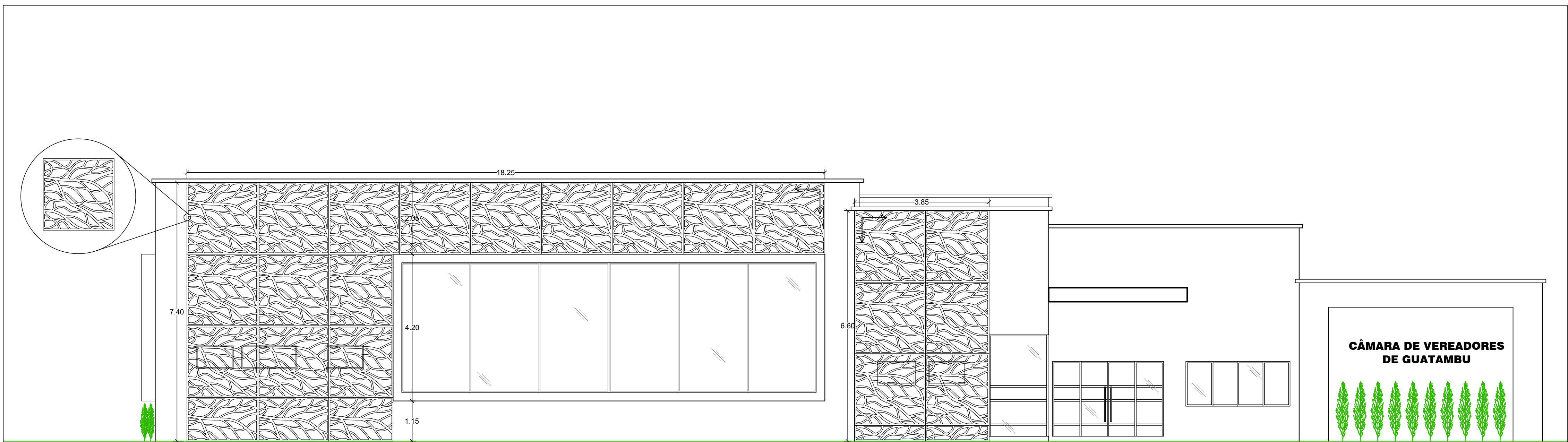
Elevação Frontal Sul
