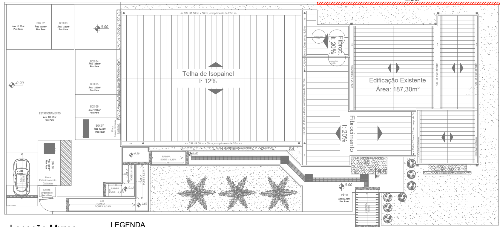
Locação Muros Escala: S/E
