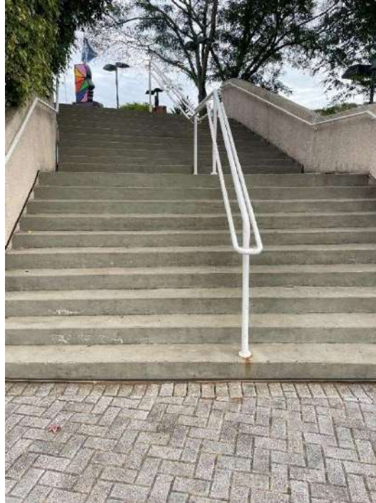
Fotografia 120 - Fissuração contrapiso escada Classificação: vício, congênito, endógeno.
