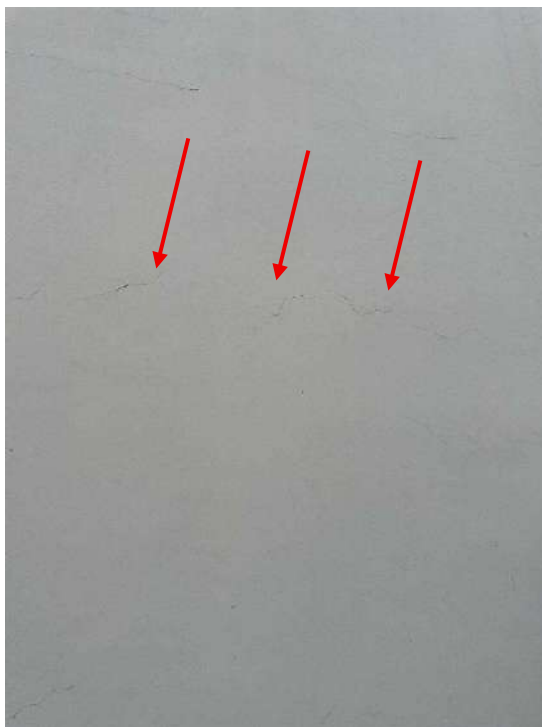
Fotografia 67 - Fissura por provável retração de argamassa
