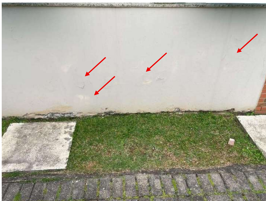
Fotografia 15 - Fissura por provável retração de argamassa / Infiltração Classificação: Vício, congênito / adquirido, endógeno.
