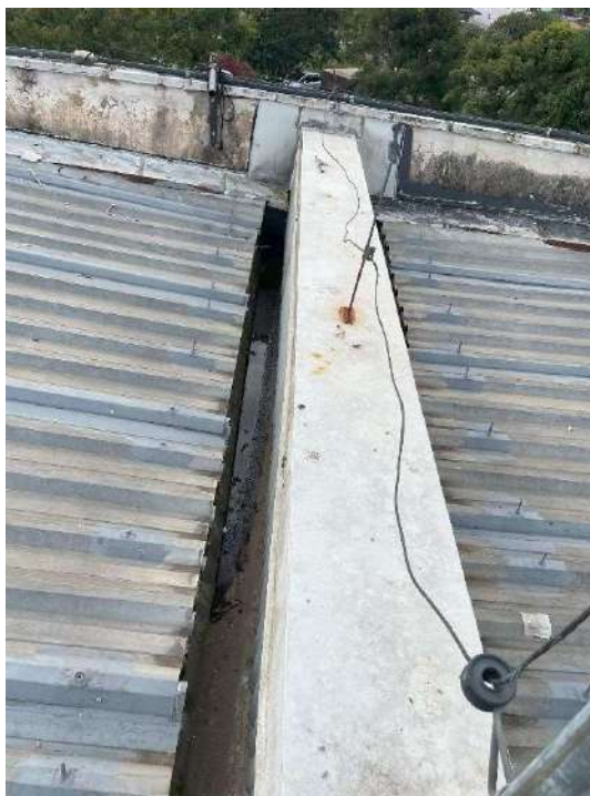
Fotografia 102 - Cabos do SPDA soltos
