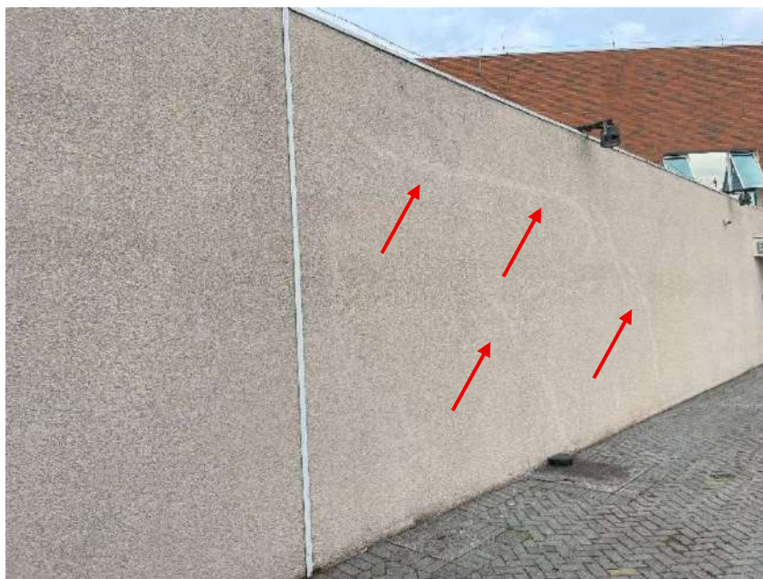
Fotografia 49 - Fissura por provável retração de argamassa
