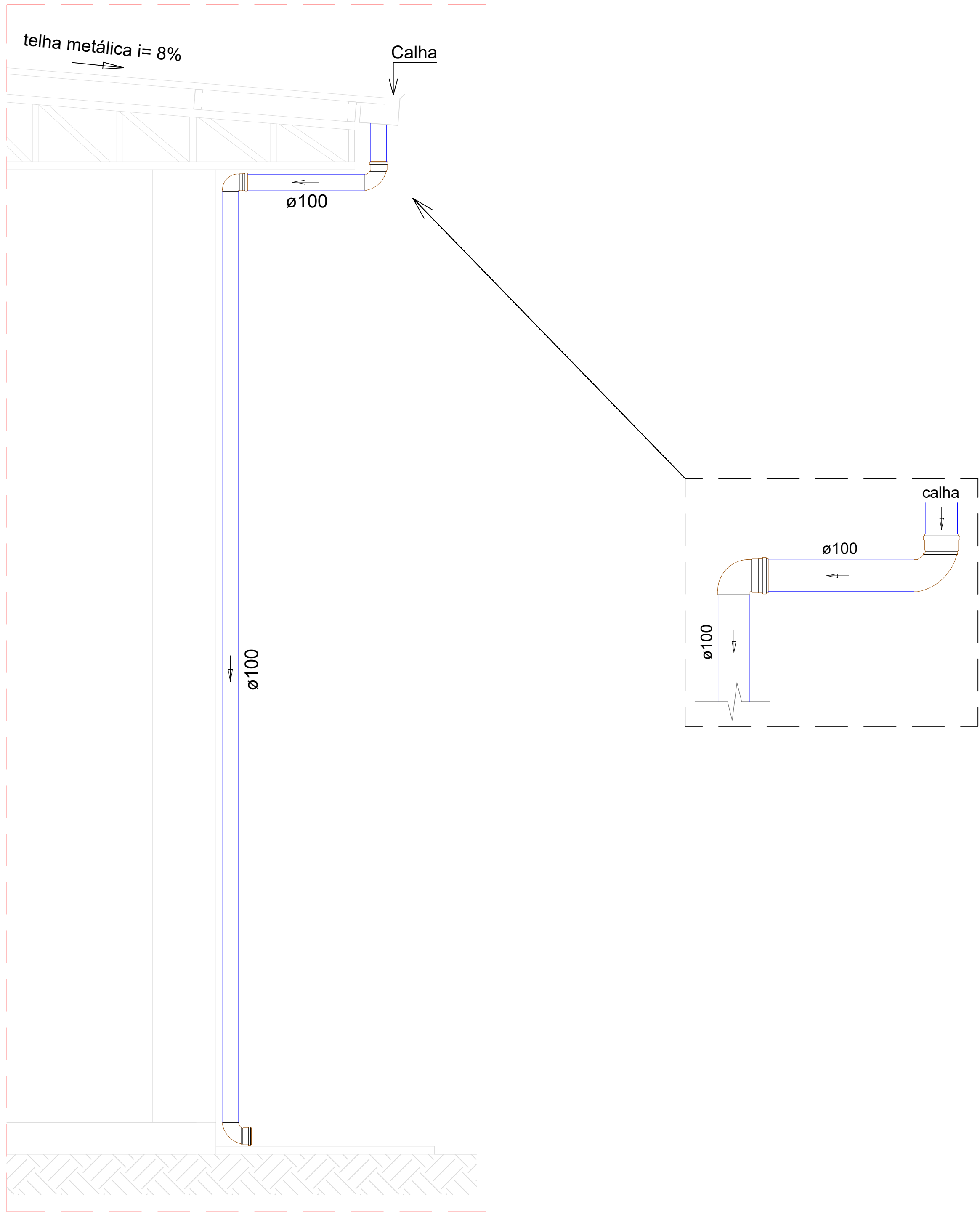
Detalhe descida calha - Det. 1 esc. 1:20
