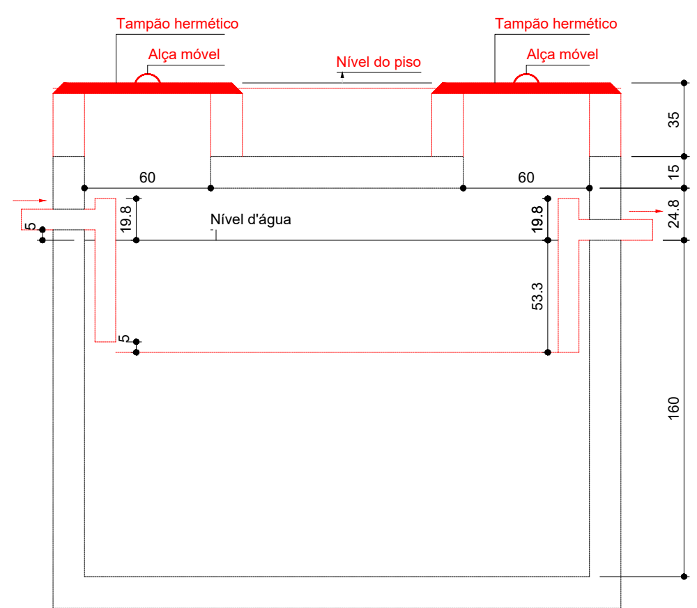
Tanque séptico - Térreo Corte 1 - ESC. 1:25
