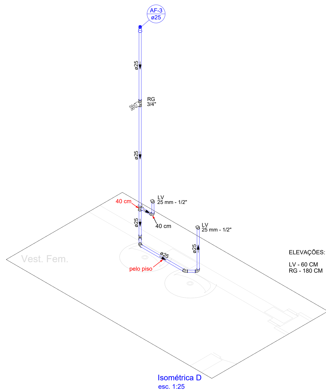
Isométrica D esc. 1:25
