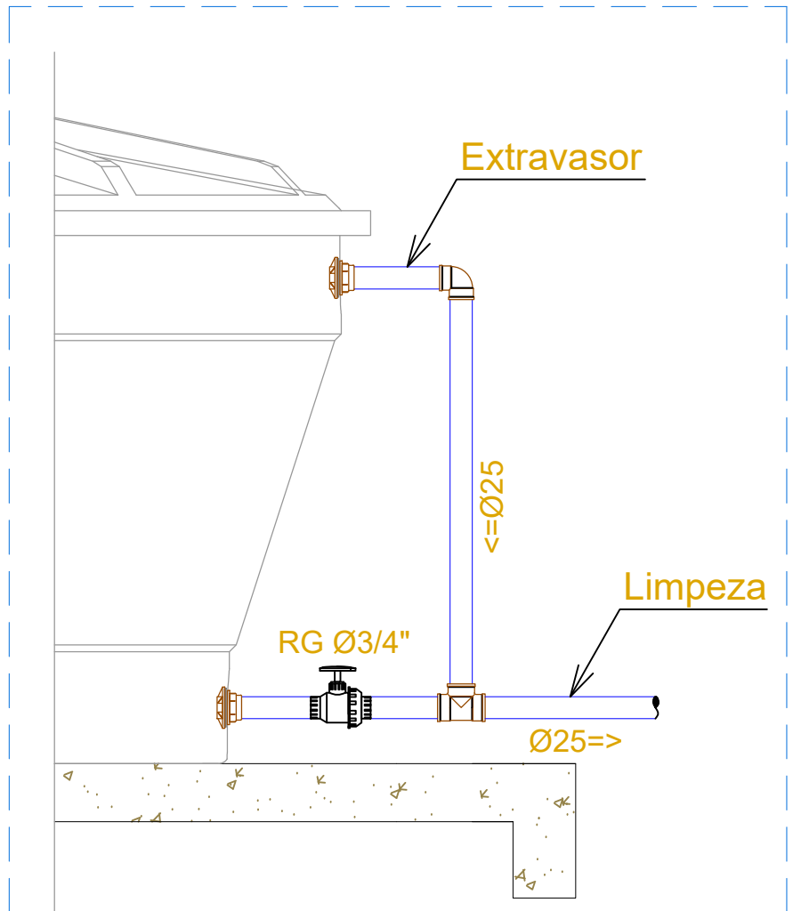
Detalhe extravasor e limpeza caixa d'água esc. 1:15
