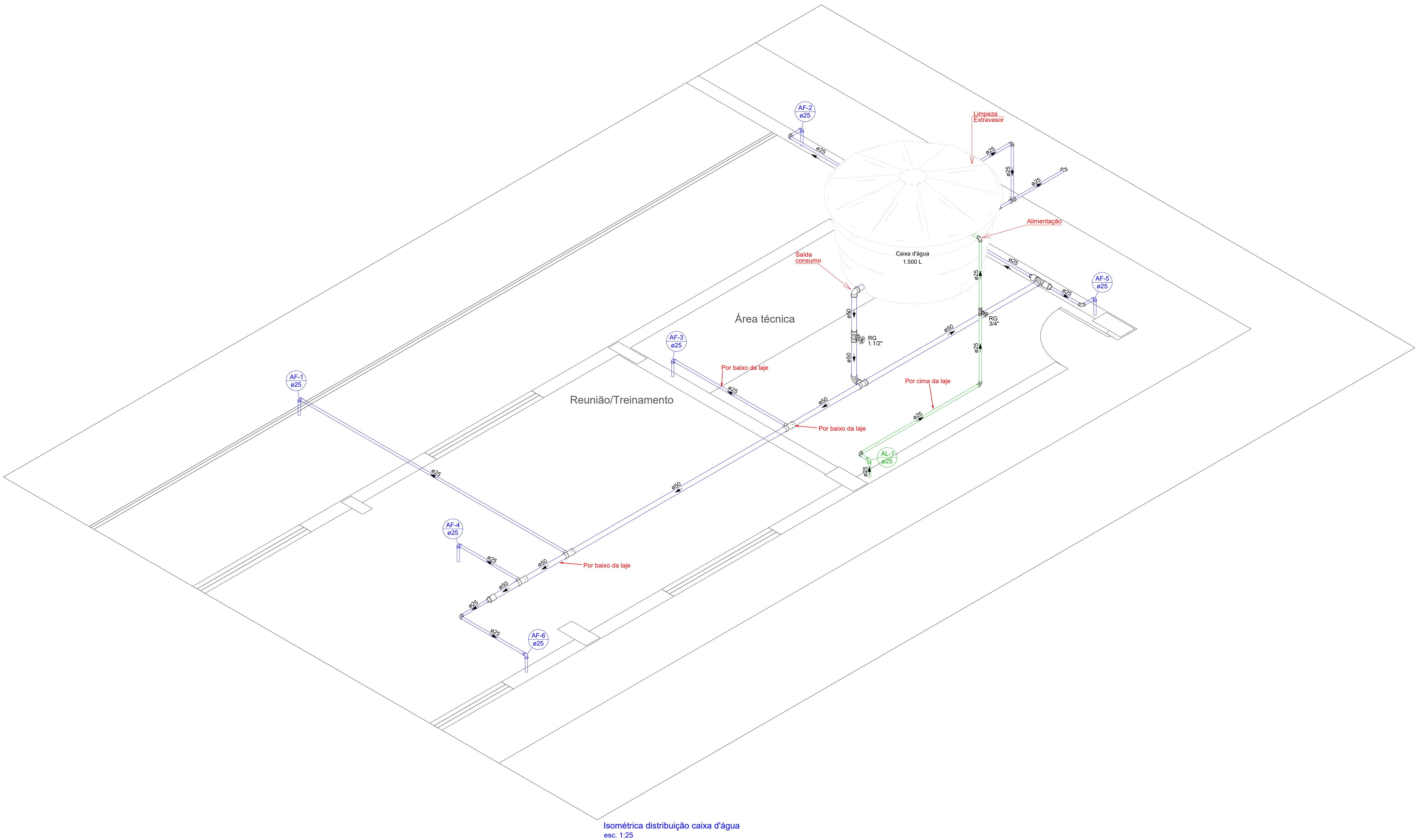
Isométrica distribuição caixa d'água esc. 1:25
