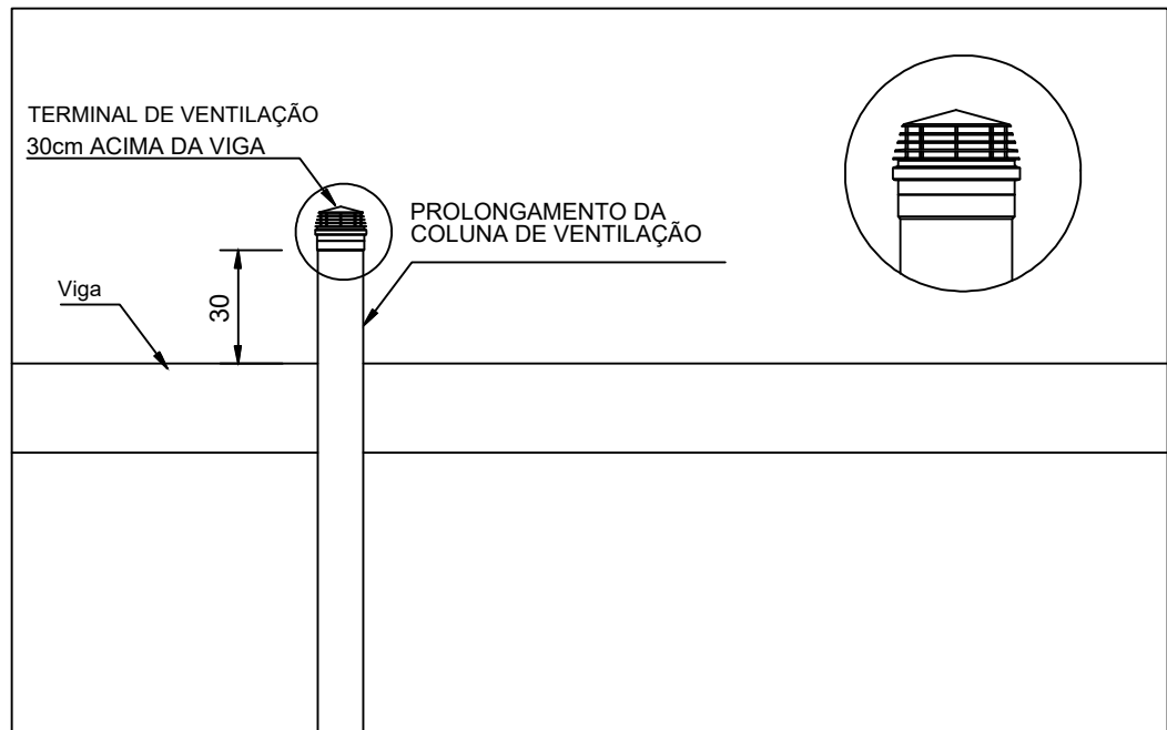
DETALHE - GENÉRICO - TERMINAIS DE VENTILAÇÃO SEM ESCALA
