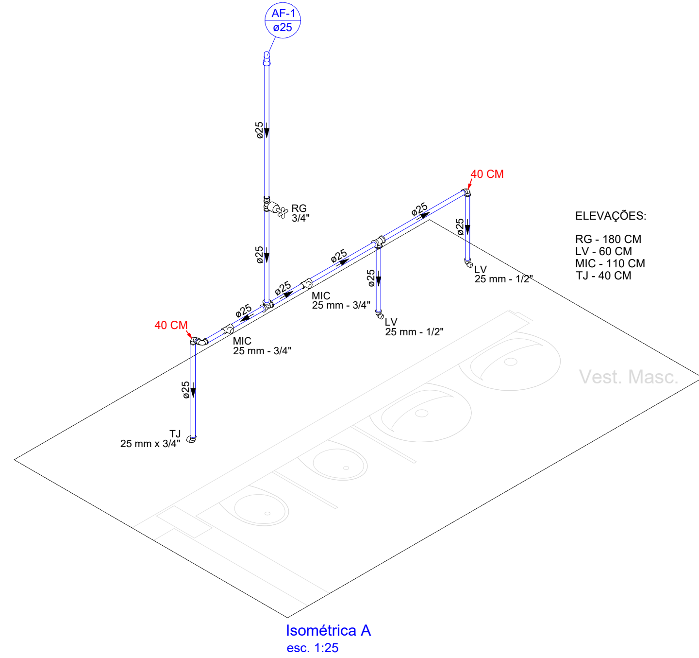
Isométrica A esc. 1:25
