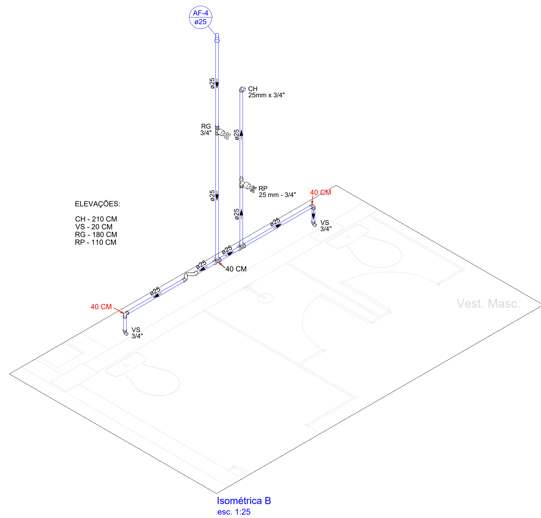
Isométrica B esc. 1:25
