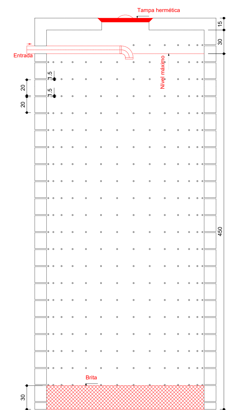
Sumidouro - Térreo Corte 1 - ESC. 1:25
