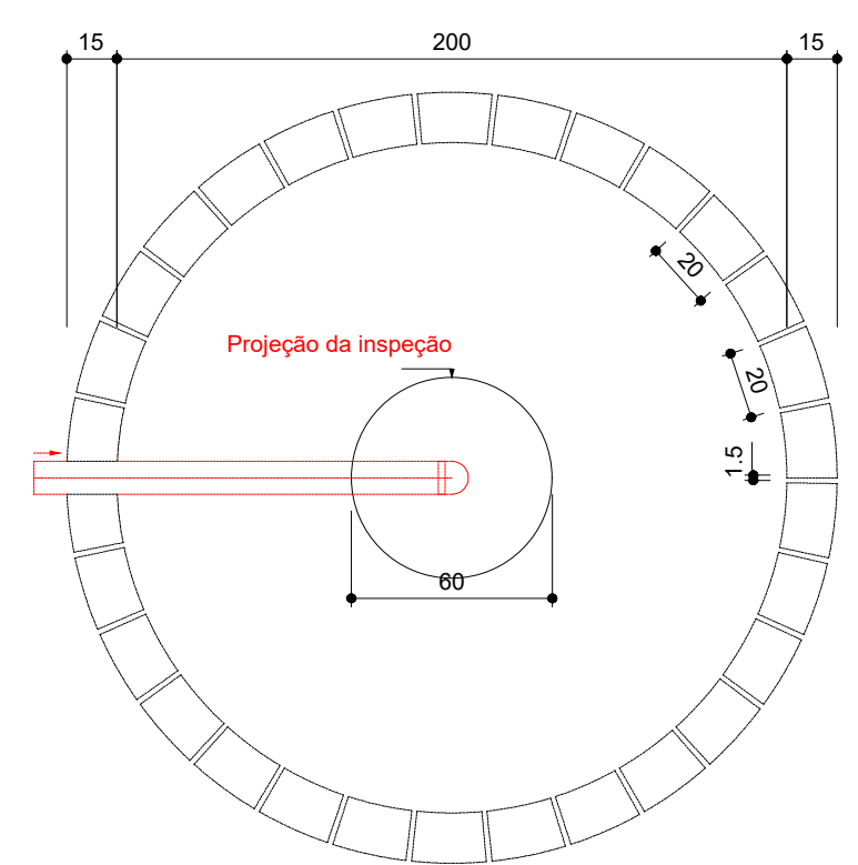
Sumidouro - Térreo Planta baixa - ESC. 1:25
