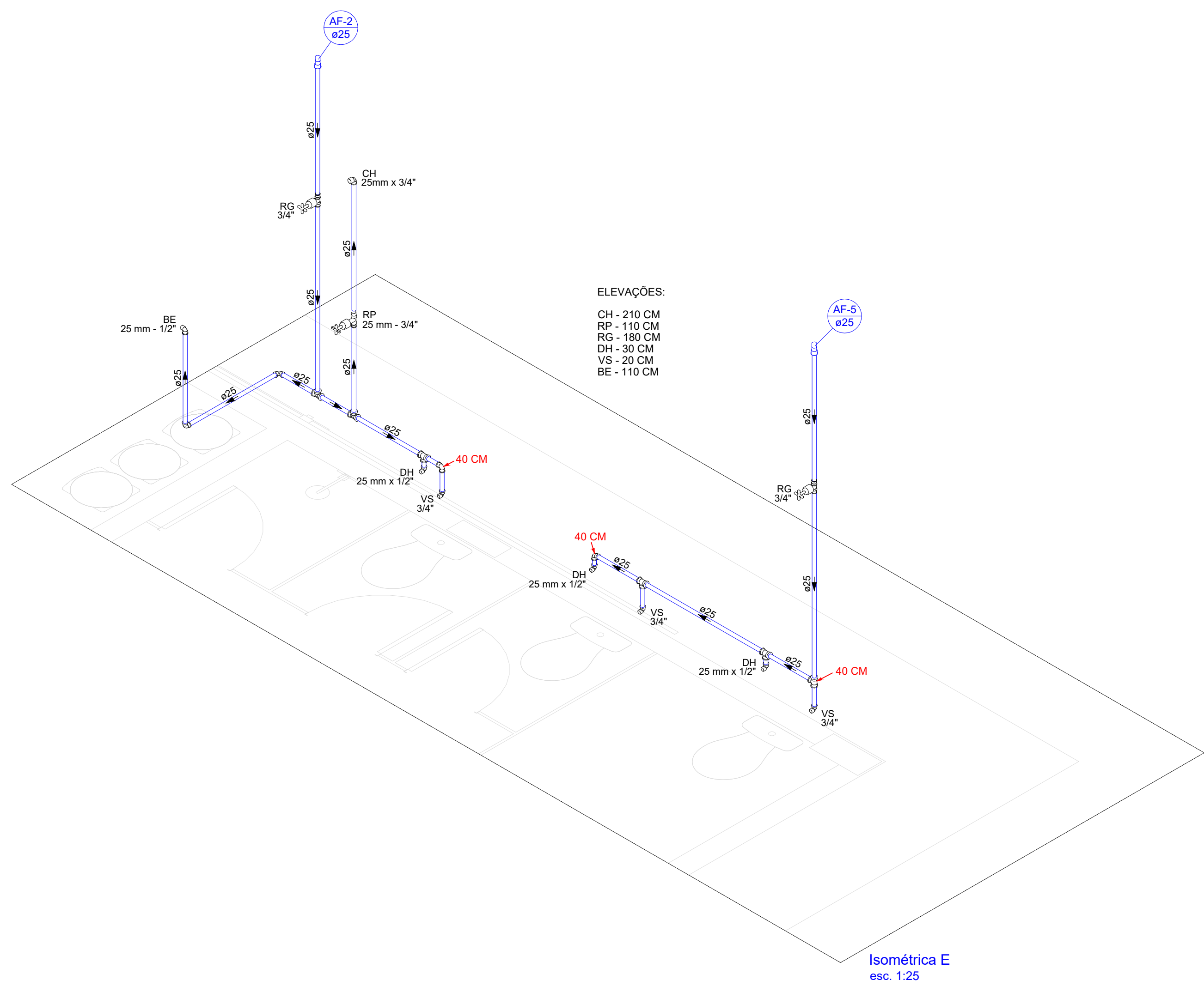
Isométrica E esc. 1:25
