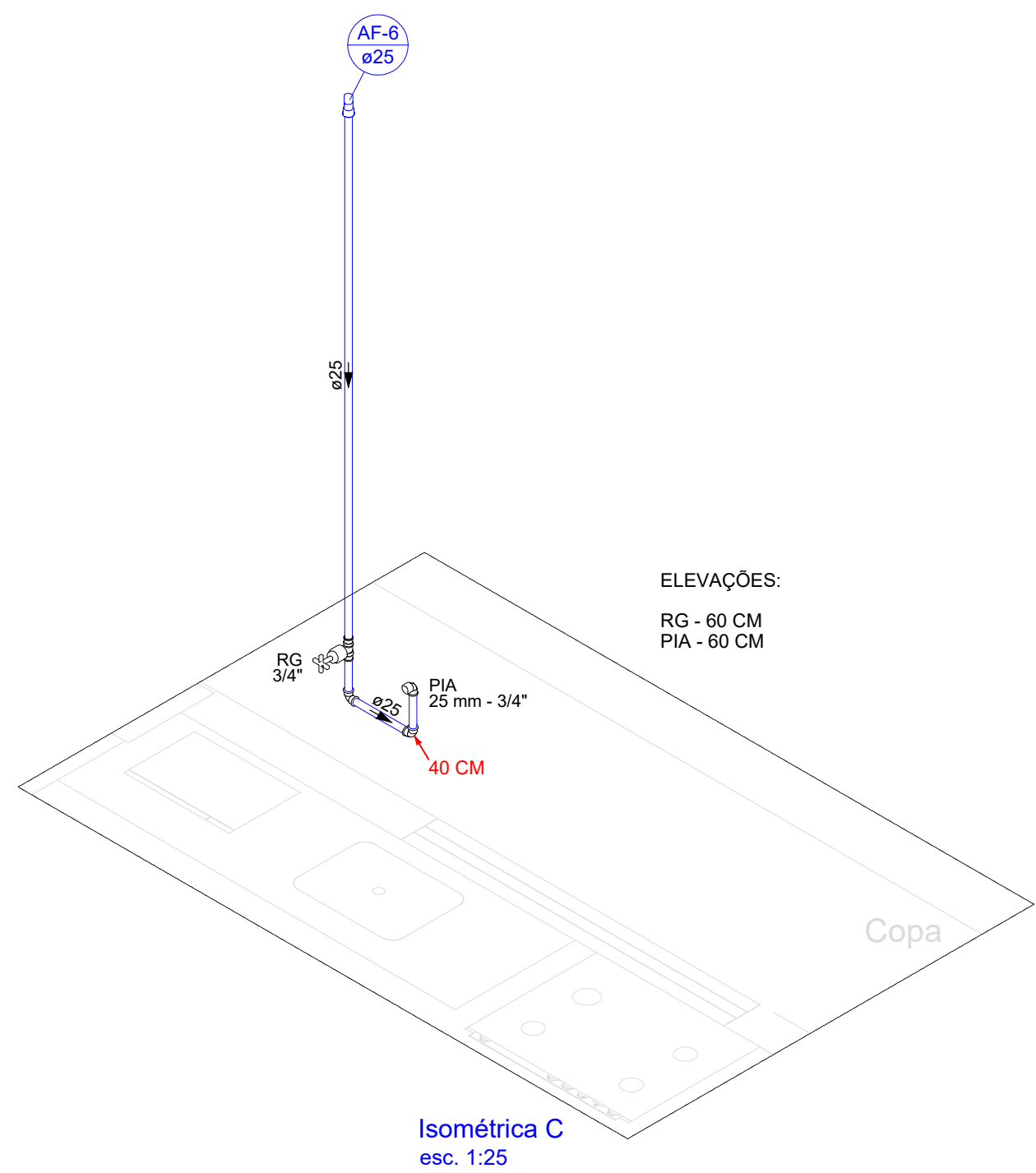
Isométrica C esc. 1:25
