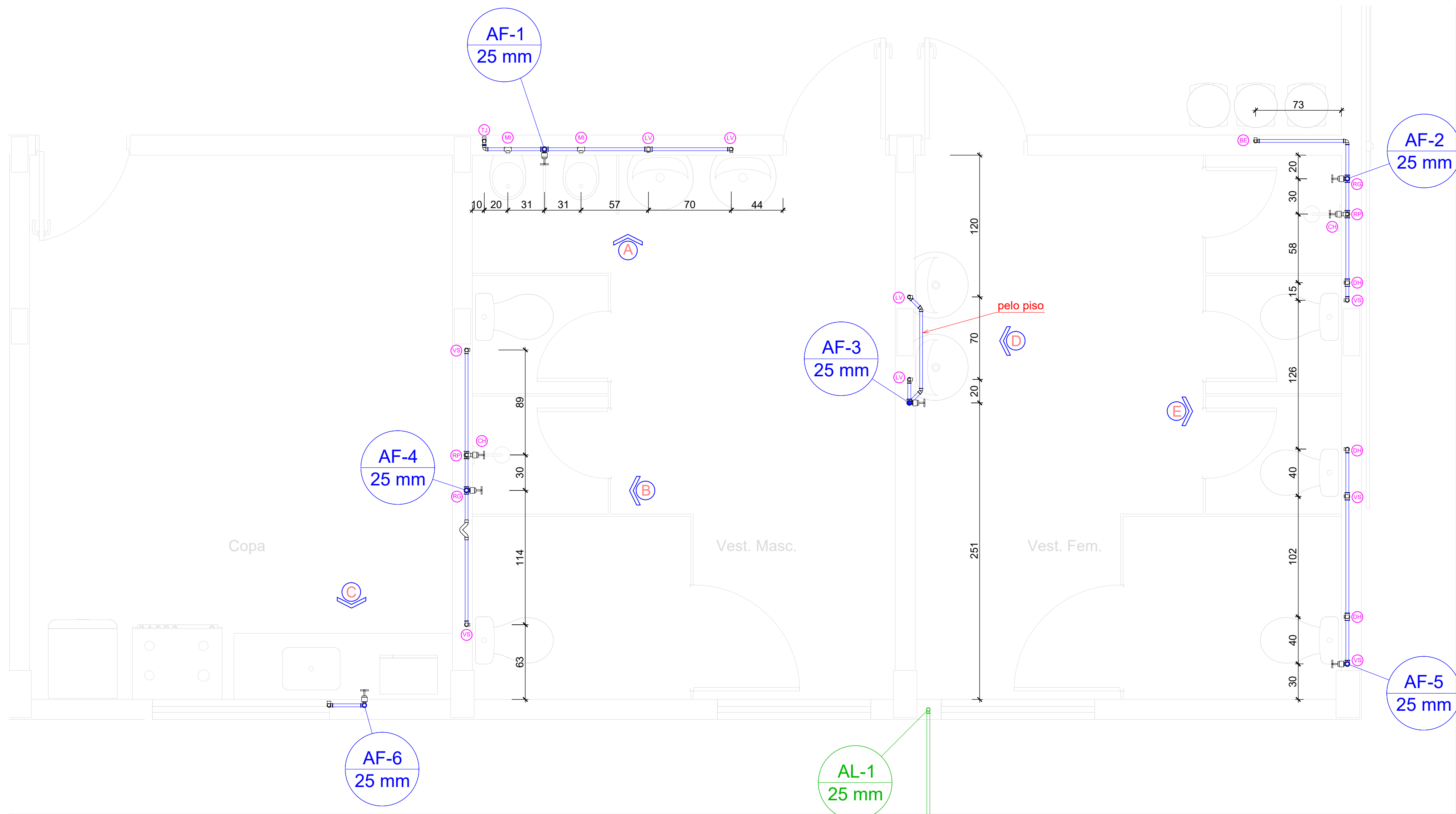
Planta hidráulica - área molhada esc. 1:25
