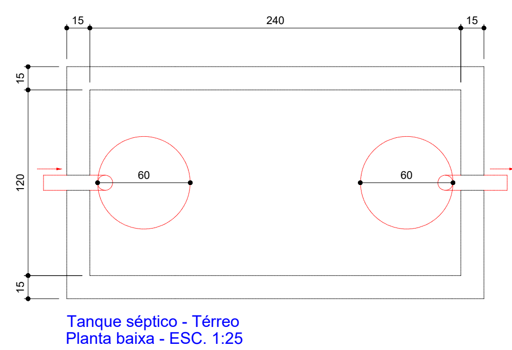
Tanque séptico - Térreo Planta baixa - ESC. 1:25
