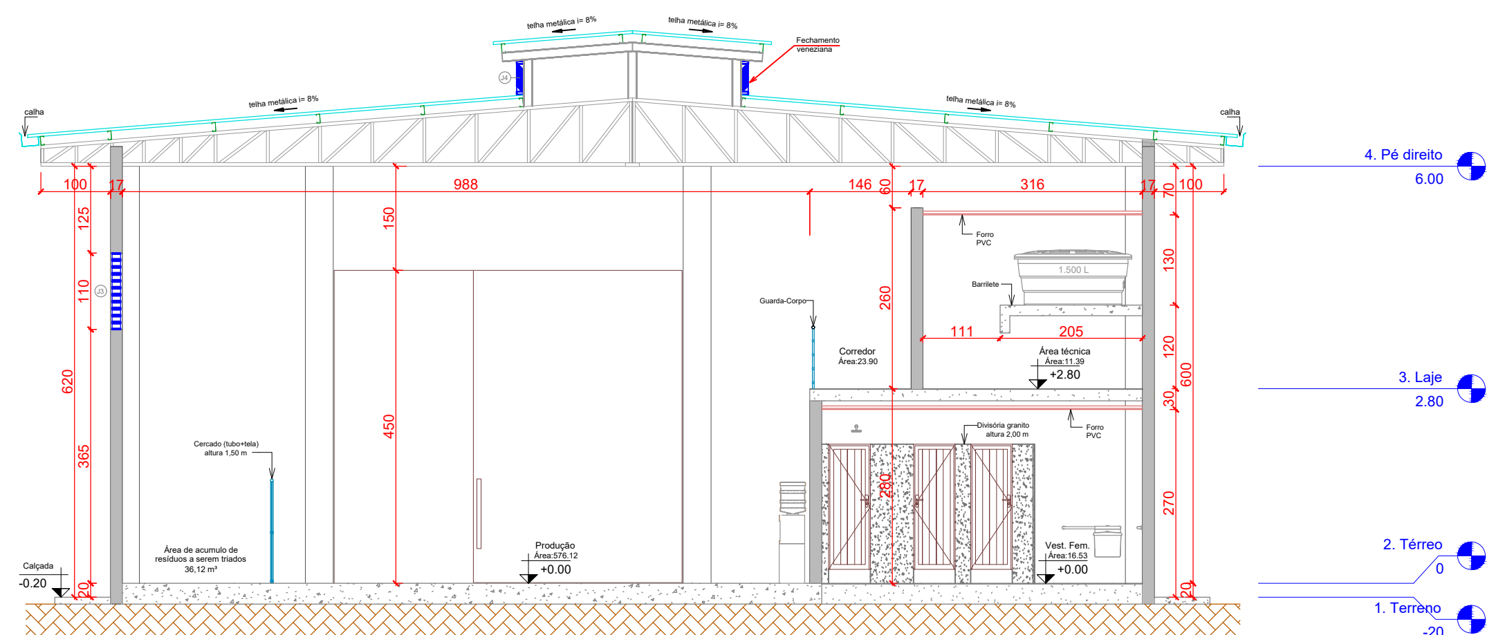
Corte D-D esc. 1:50
