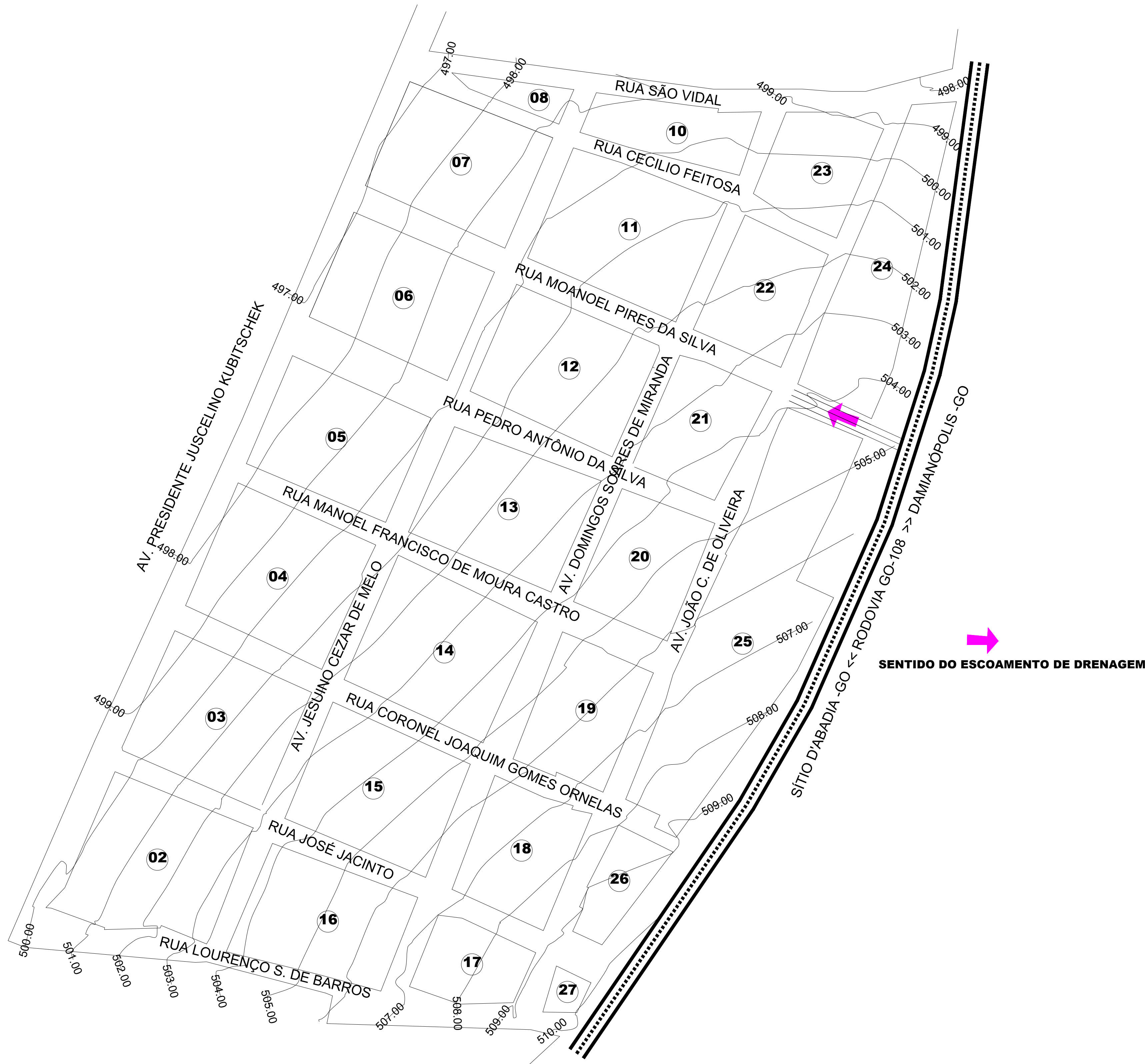
DRENAGEM - DISTRITO DE SÃO VIDAL ESC: 1:1250
