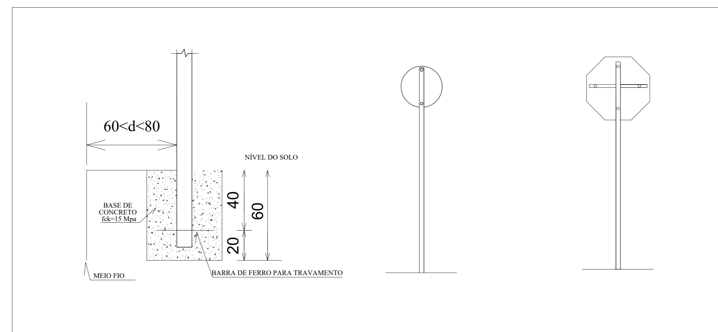
DETALHE FIXAÇÃO E CHUMBAMENTO PLACAS SEM ESCALA
