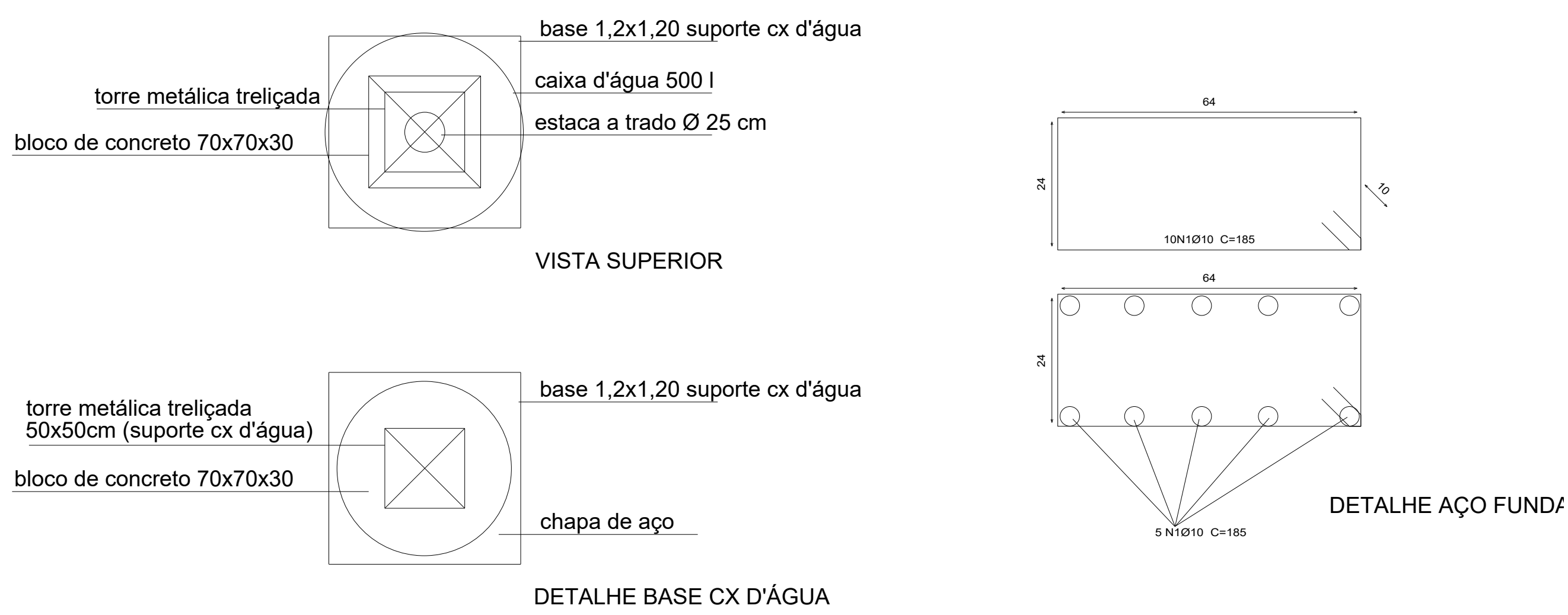
DETALHES FUNDAÇÃO ESC.:S/ESC.
