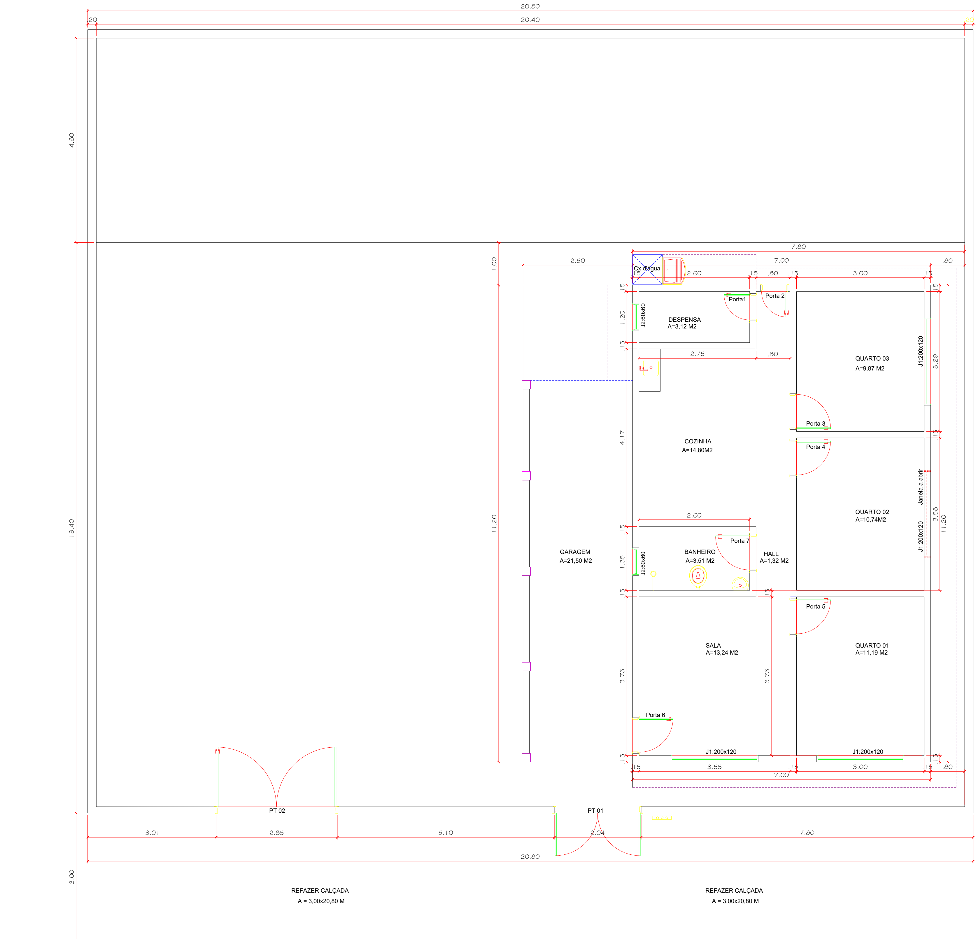
PLANTA BAIXA ESC.:1/100
