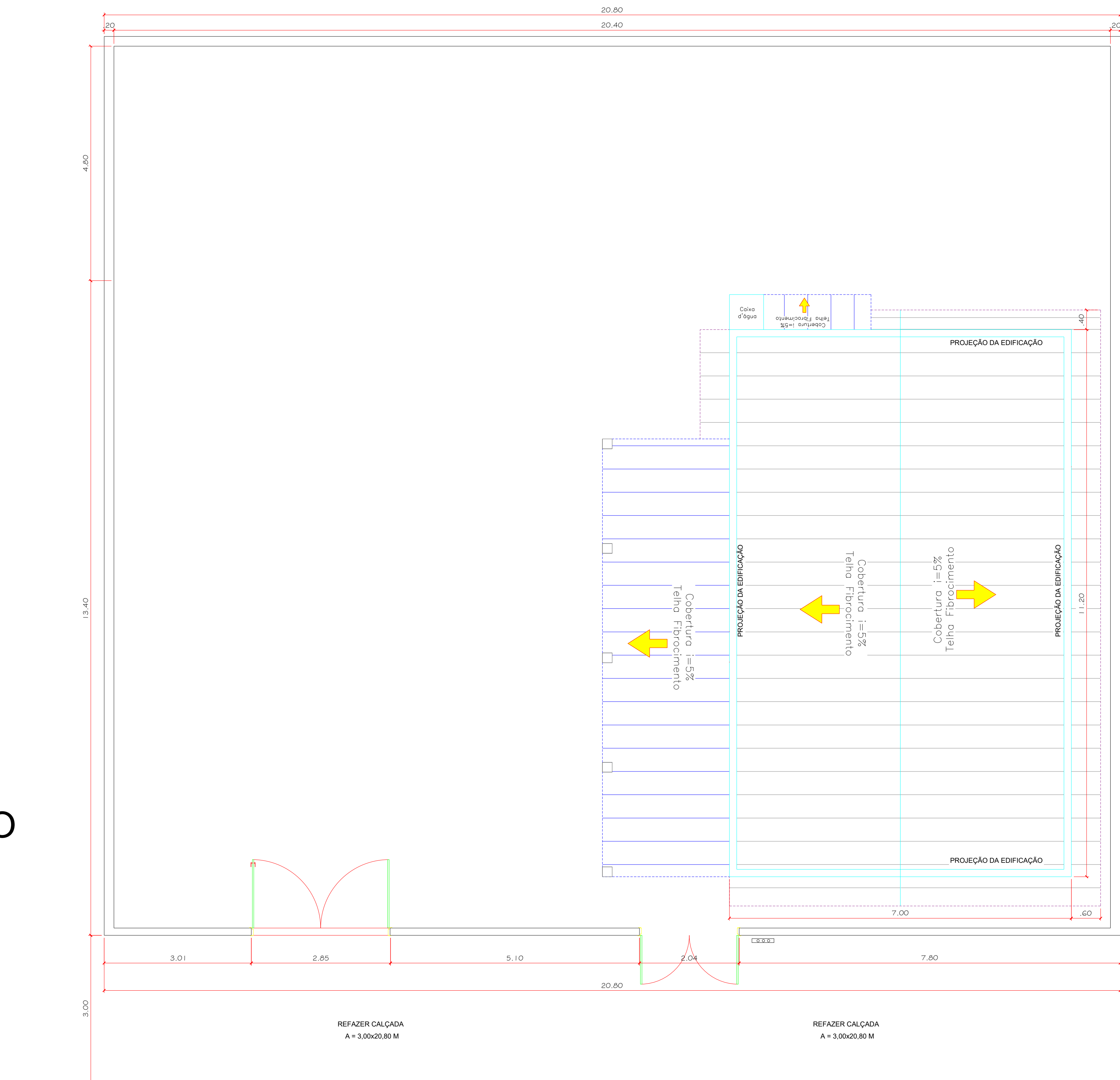
PLANTA COBERTURA ESC.:1/100
