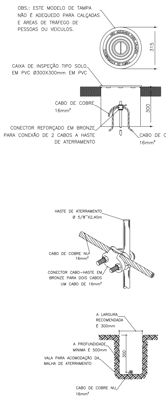
DETALHES ATERRAMENTO sem esc.
