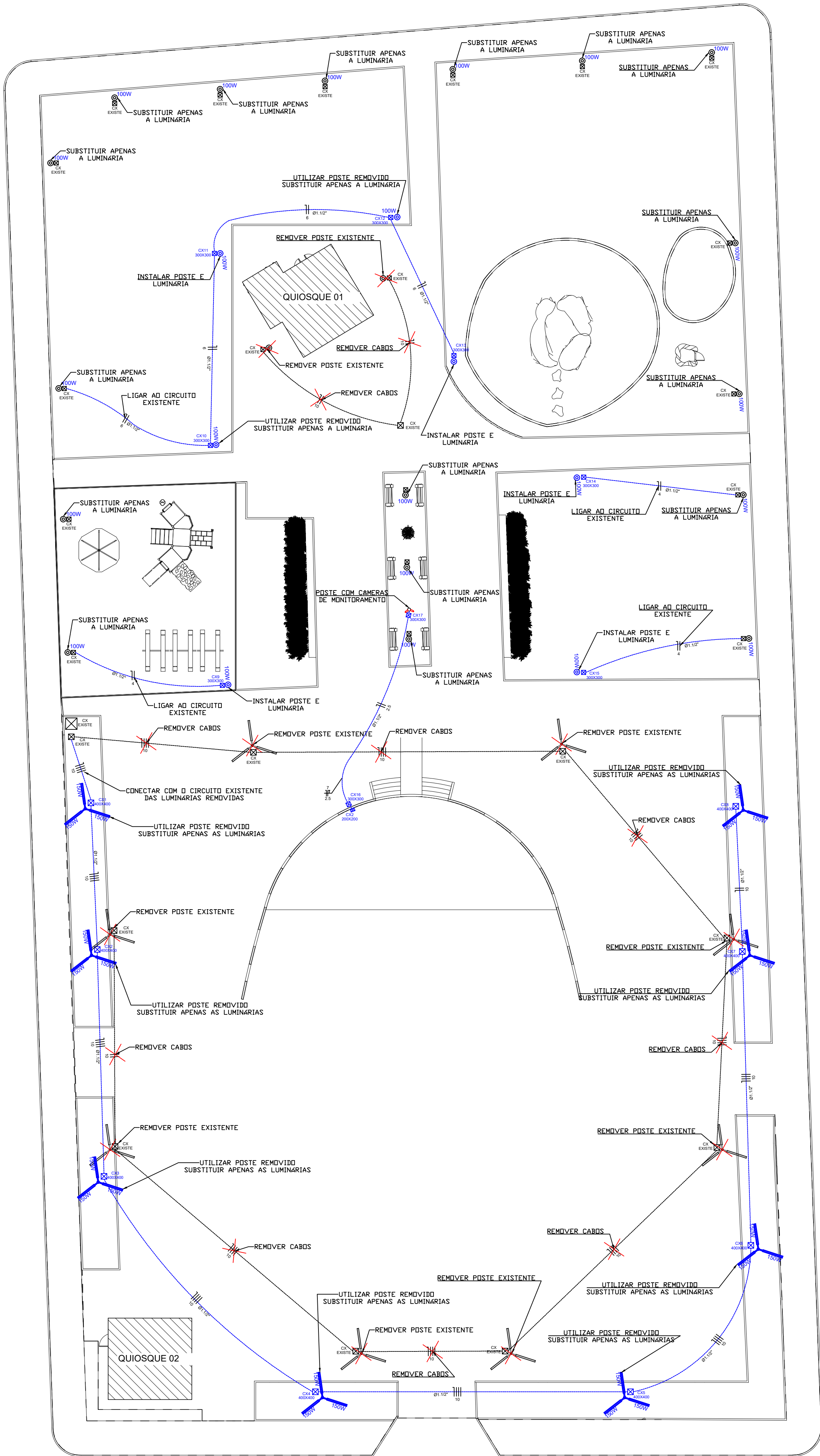
INSTALAÇÕES ELÉTRICAS PRAÇA SEM ESCALA
