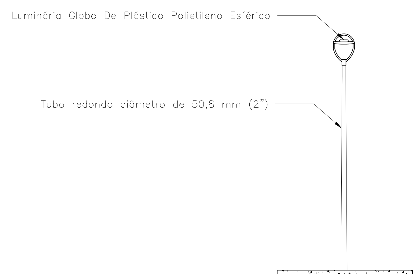
DETALHES SUBSTITUIÇÃO DAS LUMINÁRIAS sem esc.
