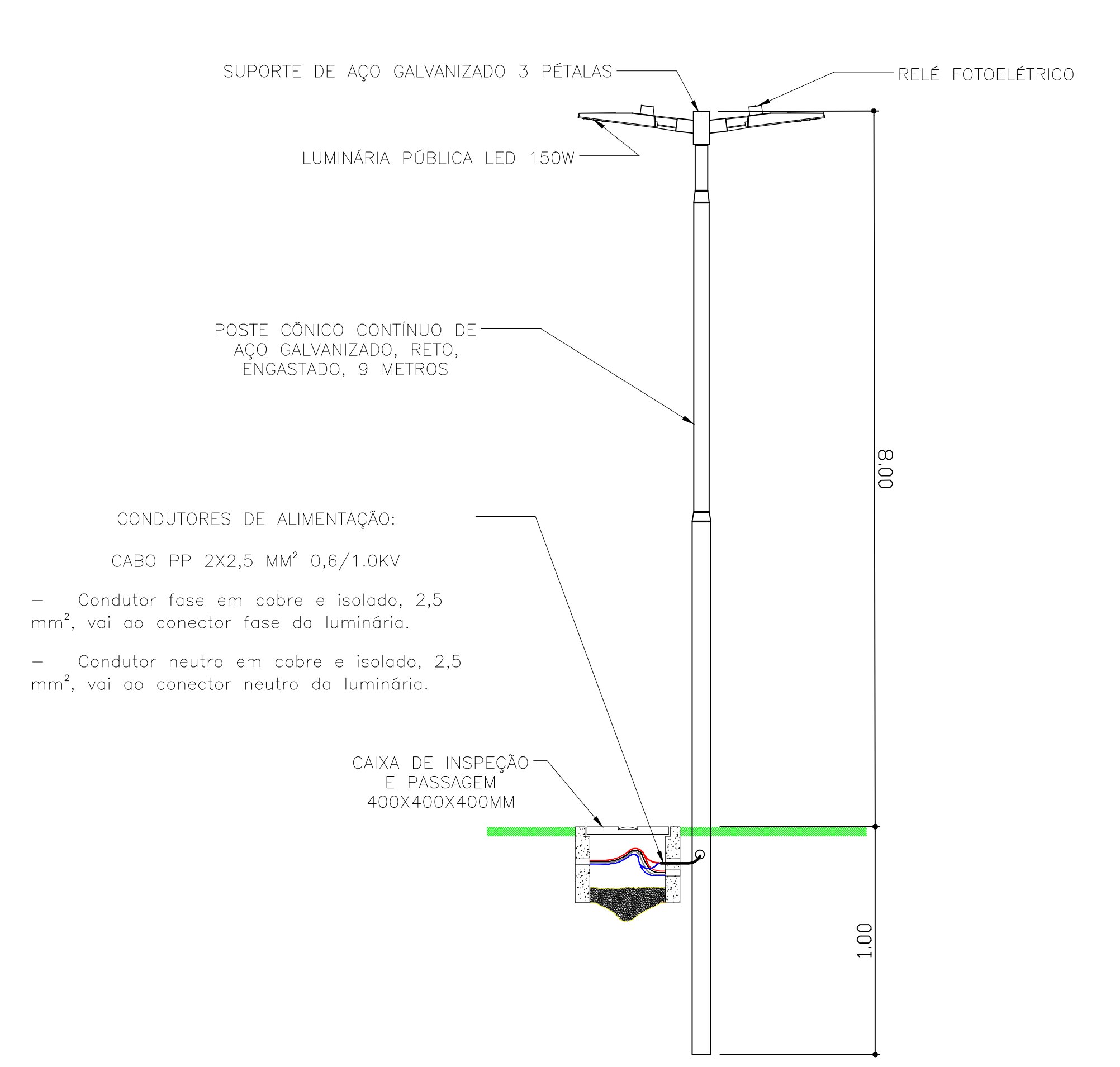
DETALHES POSTE sem esc.
