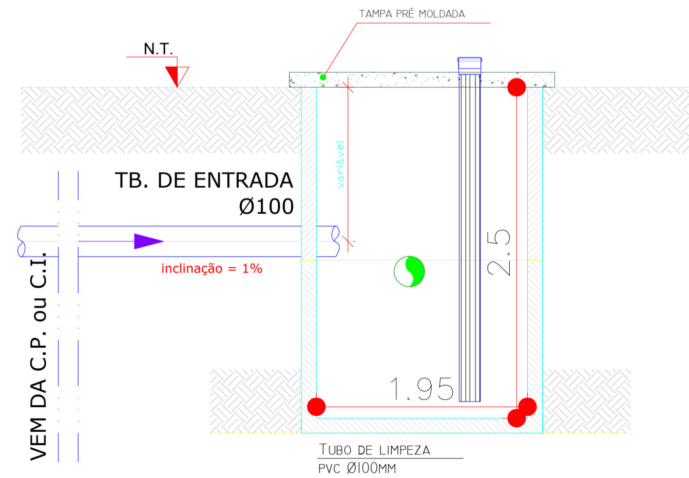
CORTE B - FOSSA SÉPTICA
