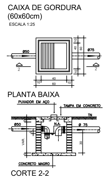
CORTE 2-2
