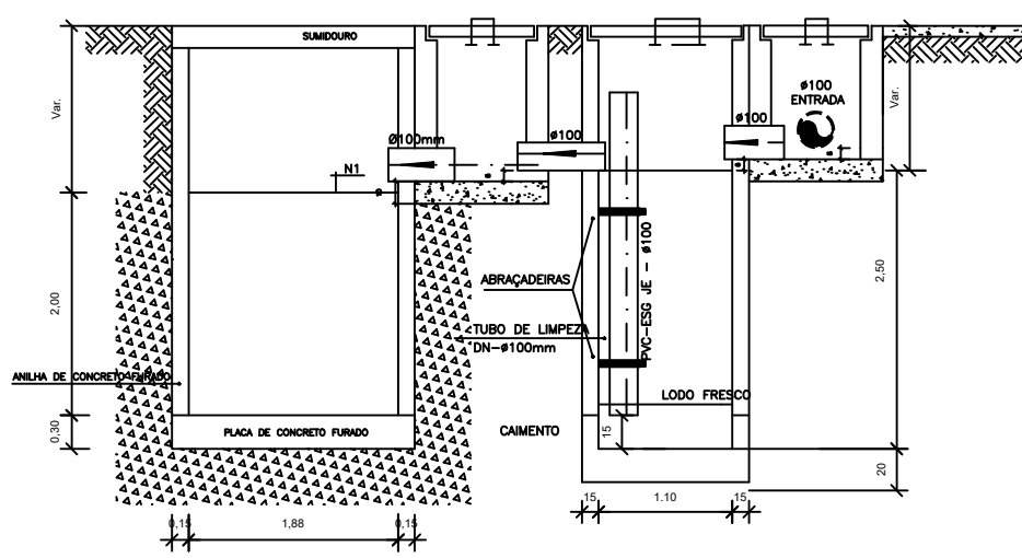
CORTE A-A - FOSSA SÉPTICA E SUMIDOURO ESCALA 1:50
