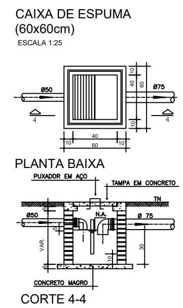
CORTE 4-4
