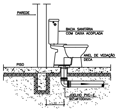
DETALHE GENÉRICO DO VASO SANITÁRIO ESCALA 1:25
