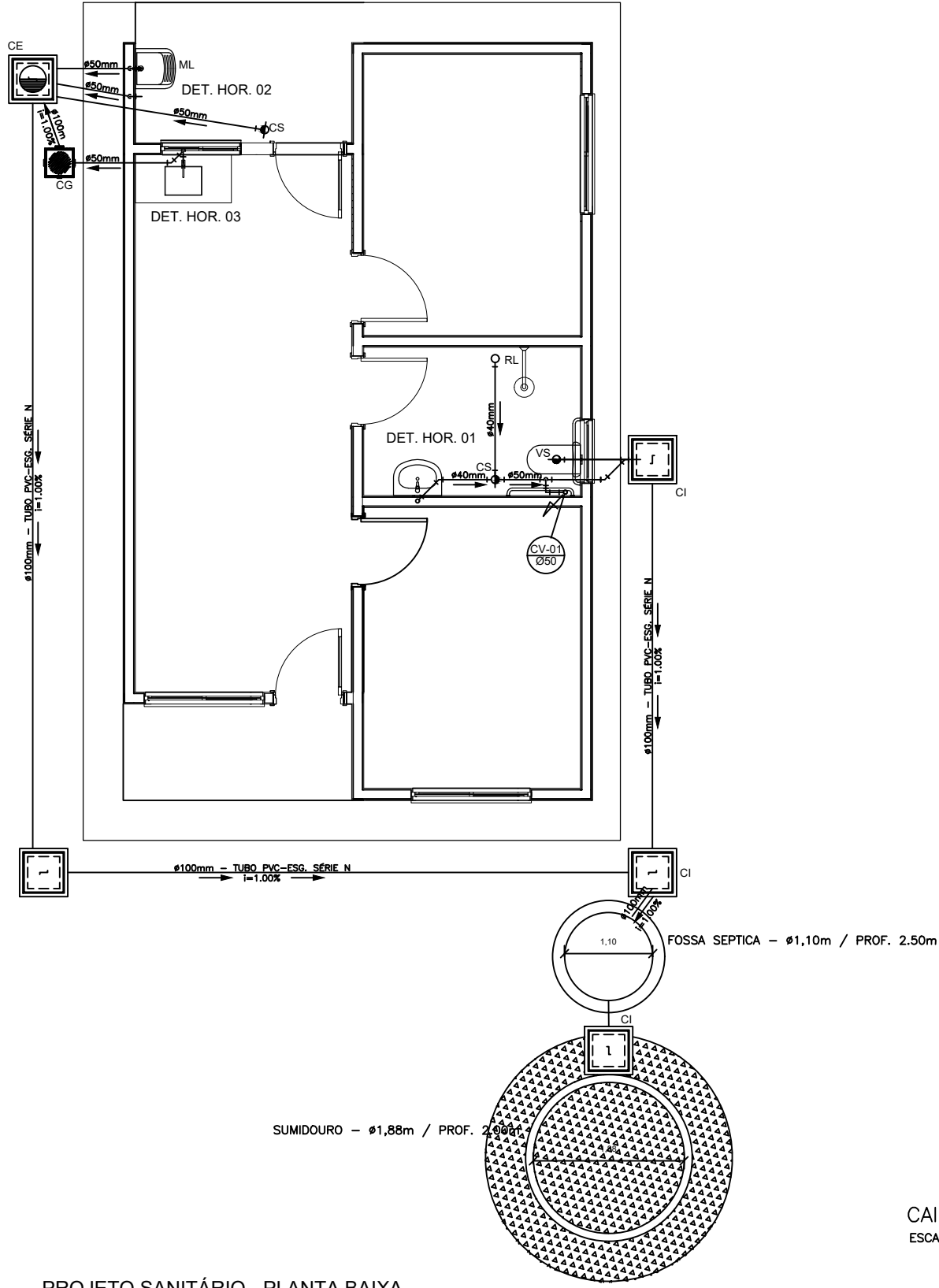
PROJETO SANITÁRIO - PLANTA BAIXA ESCALA 1:50
