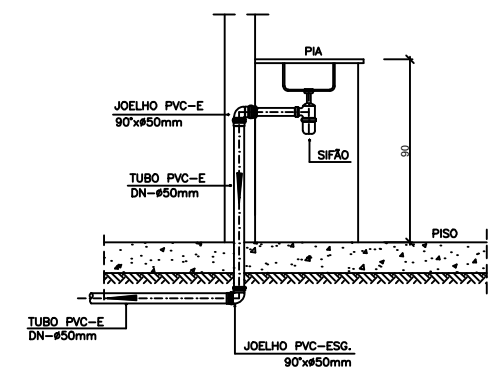
DETALHE DA PIA ESCALA 1:25
