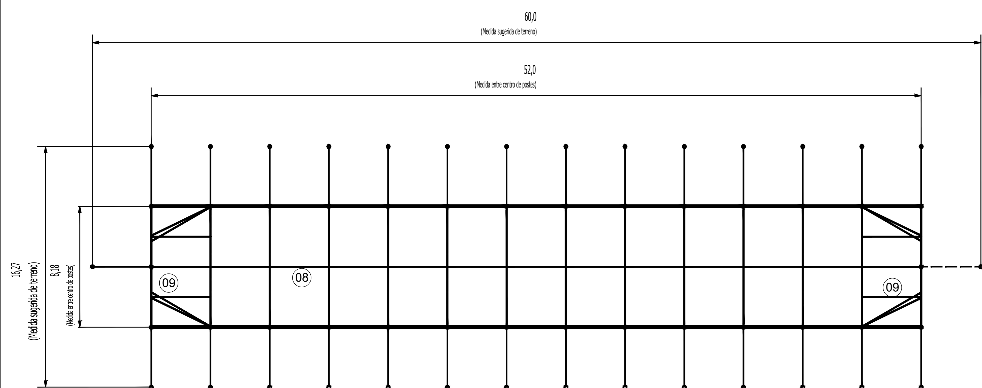
PLANTA BAIXA:
