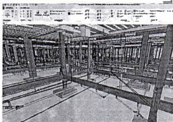
Vista 3D de instalações Hidrossanitárias e sua interferência no projeto estrutural
