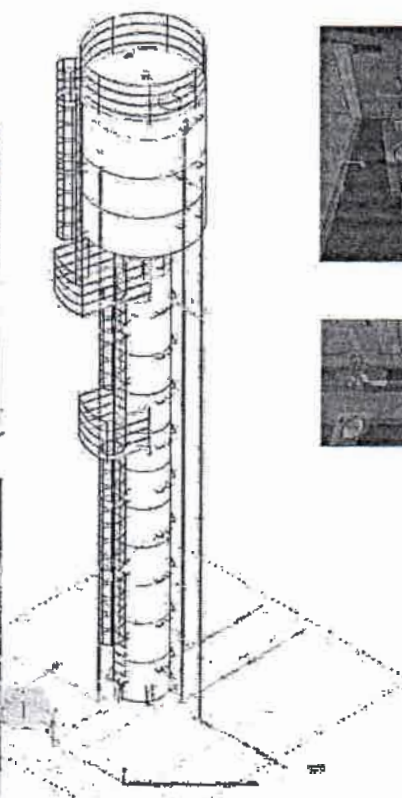
Vista 3D de reservatórios externos e de prumadas das instalações hidrossanitárias
