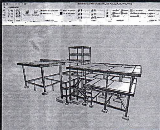
Vista 3D de um projeto de fundação e estrutural compatibilizados
