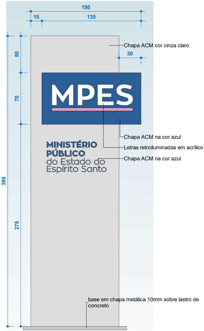
2 Elevação 1 1 : 30
