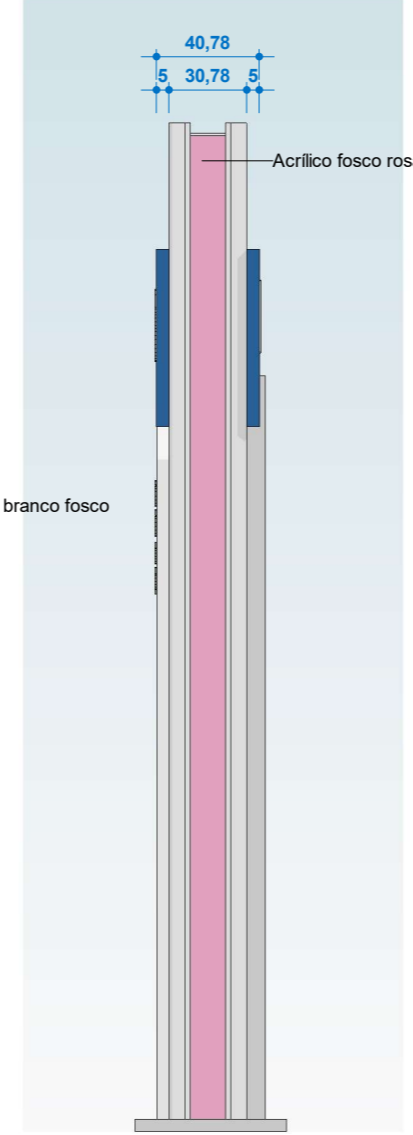
3 Elevação 2 1 : 30
