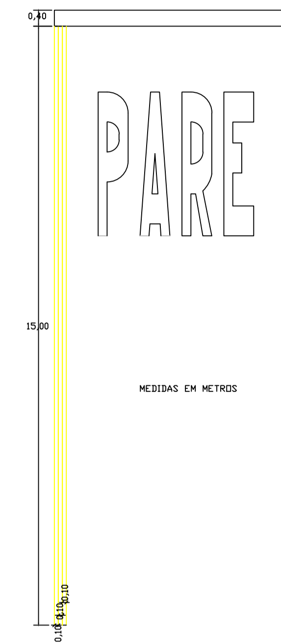
DETALHE DA SINALIZAÇÃO HORIZONTAL DE PARADA OBRIGATÓRIA
