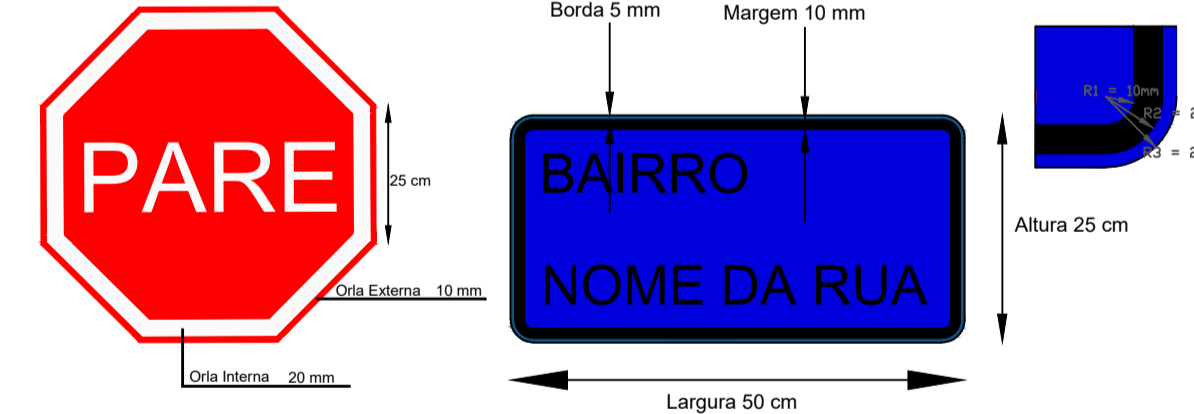
DIMENSÕES PADRÃO DAS PLACAS
