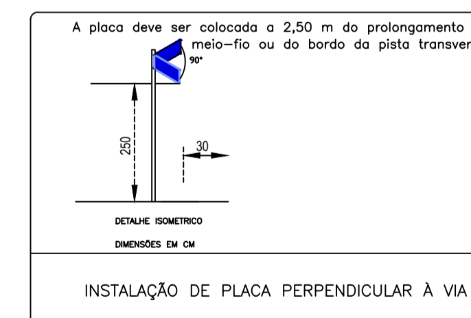
DETALHE DA PLACA DE IDENTIFICAÇÃO DE RUAS
