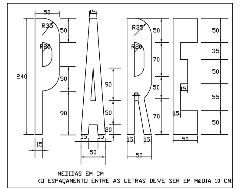
DIAGRAMAÇÃO DA LEGENDA "PARE"
