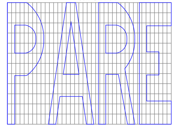
DIAGRAMAÇÃO DA LEGENDA "PARE"
