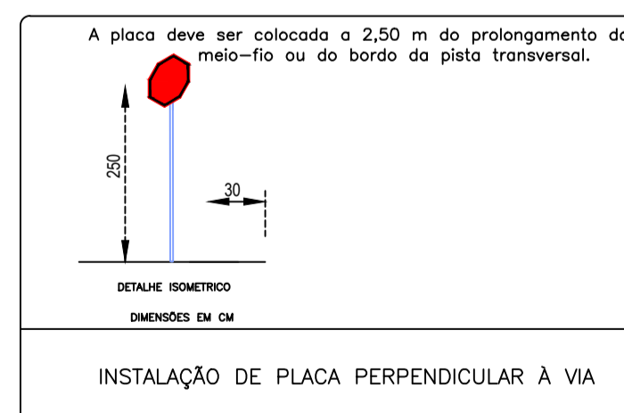
DETALHE DA PLACA DE ADVERTÊNCIA
