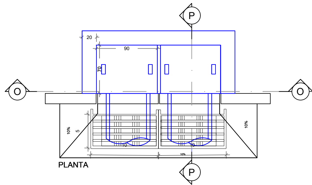
DETALHE BOCA DE LOBO DUPLA COM GRADE E ABERTA NA GUIA
