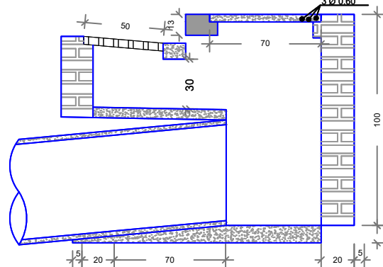
CORTE P-P
