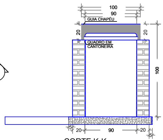
CORTE K-K
