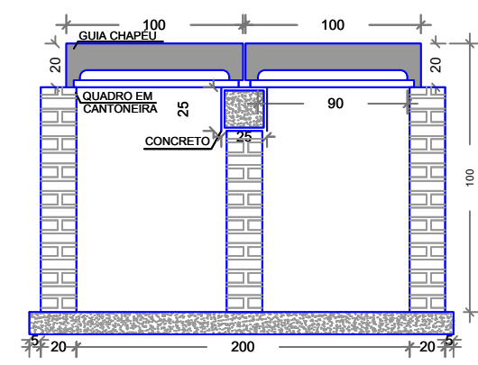
CORTE O-O
