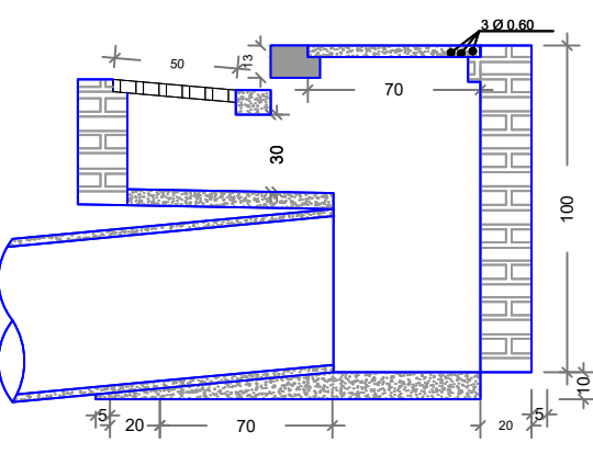
CORTE L-L
