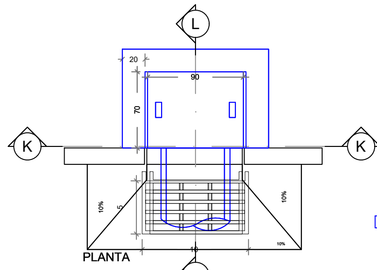
DETALHE BOCA DE LOBO SIMPLES COM GRADE E ABERTA NA GUIA
