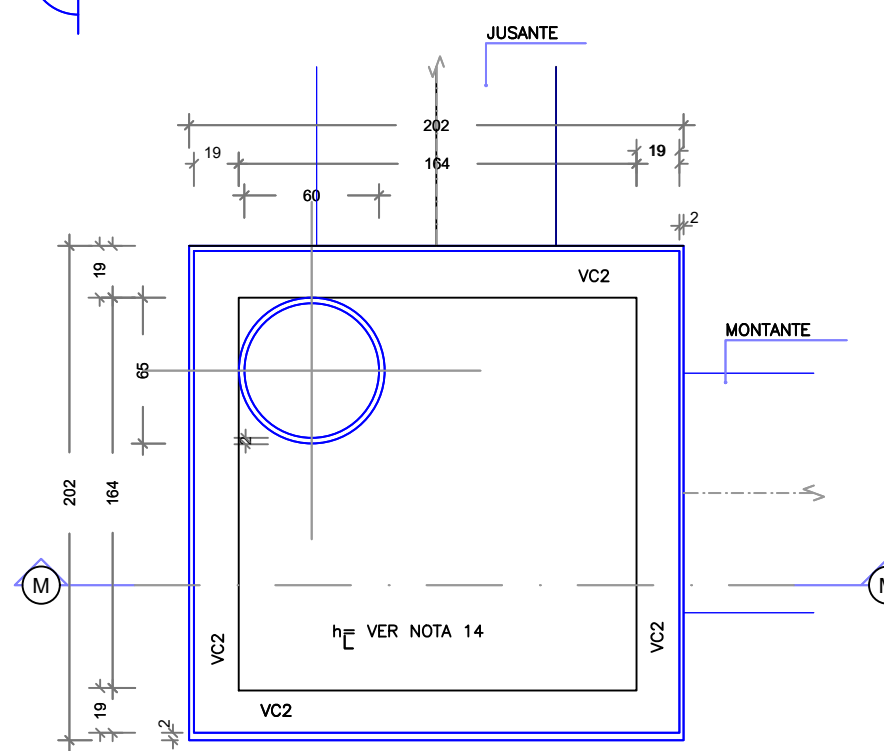
DETALHE TÍPICO DO POÇO DE VISITA
