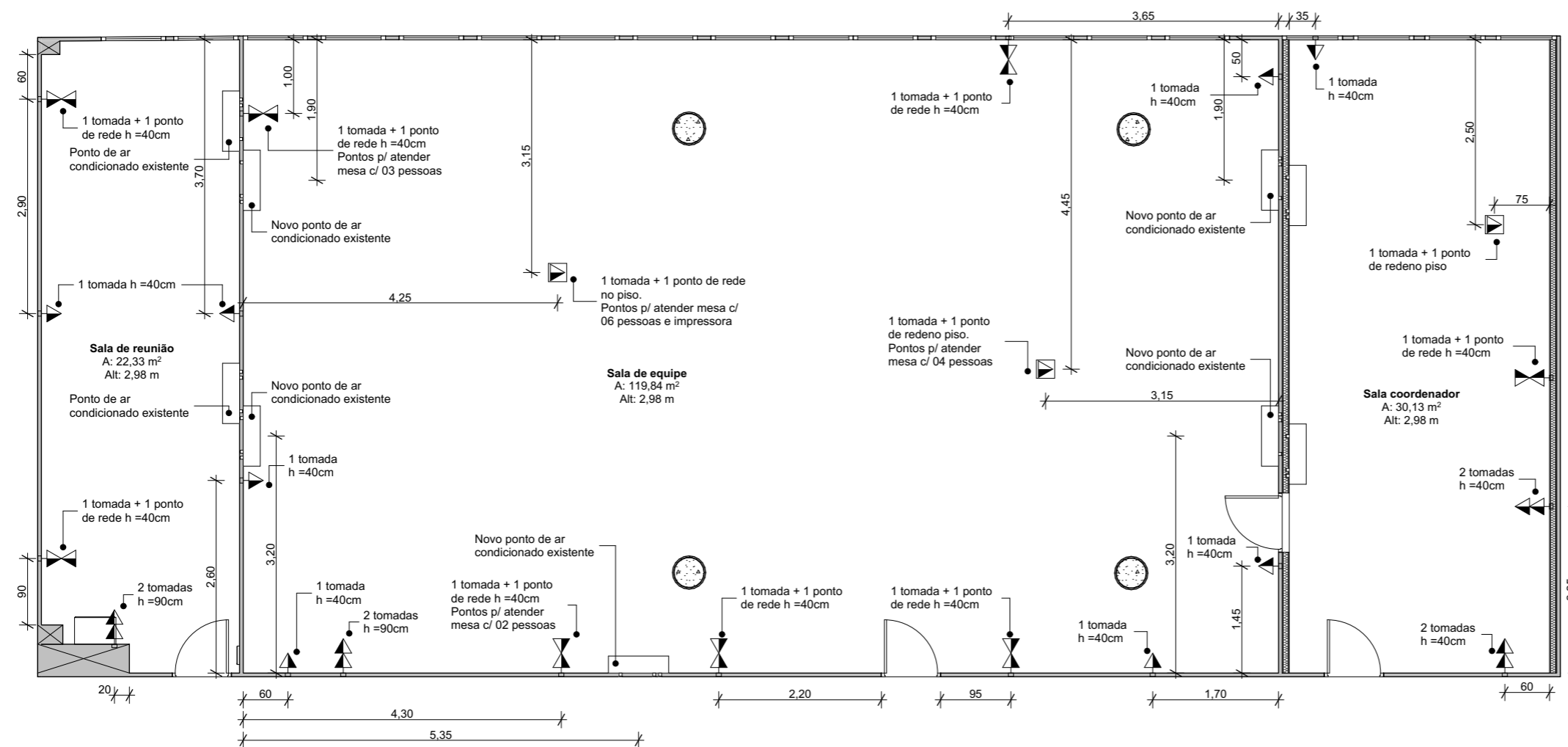
01 Planta de elétrica Escala: 1:75
