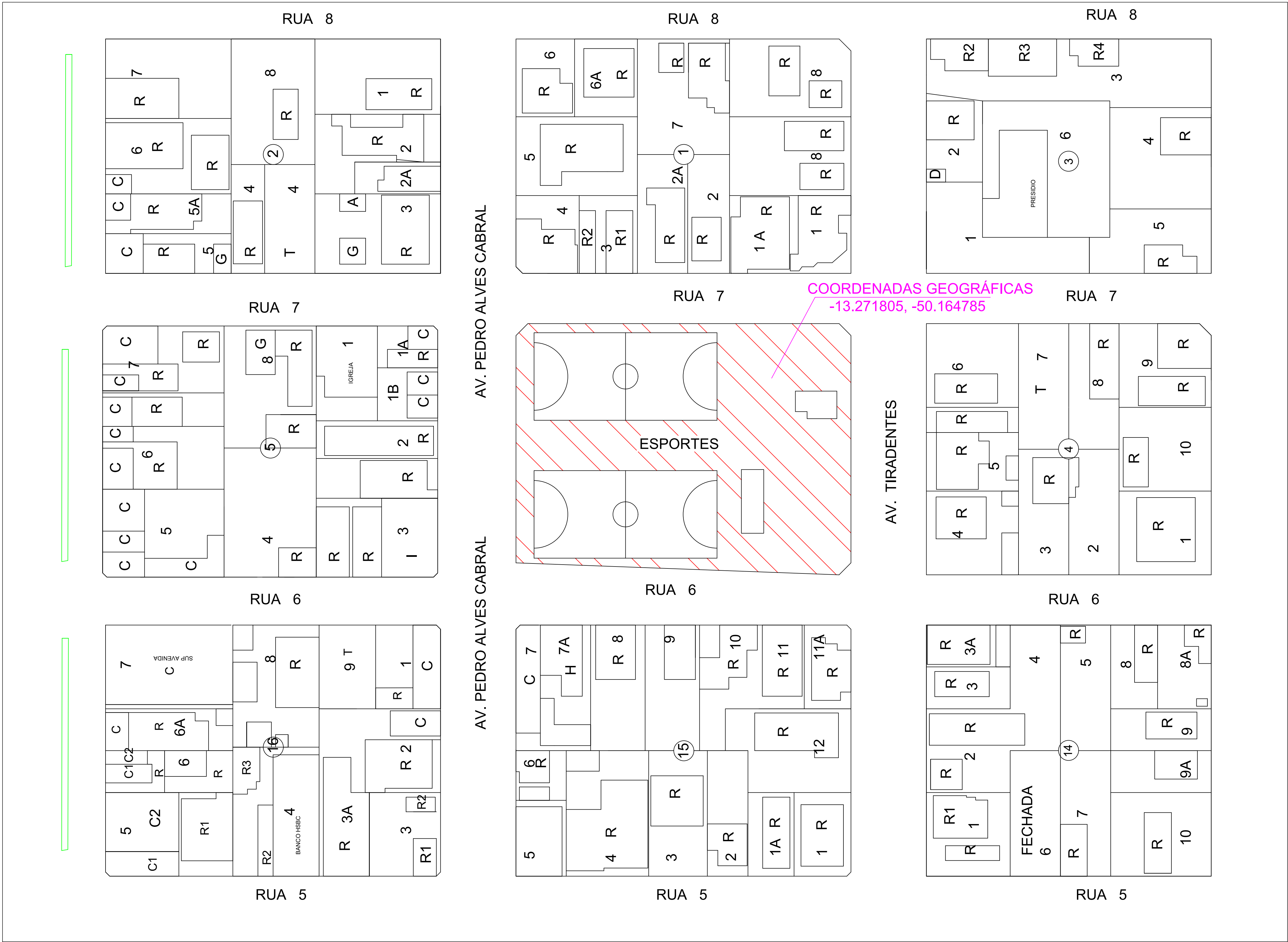
PLANTA DE LOCALIZAÇÃO DA INTERVENÇÃO ESCALA 1/500
