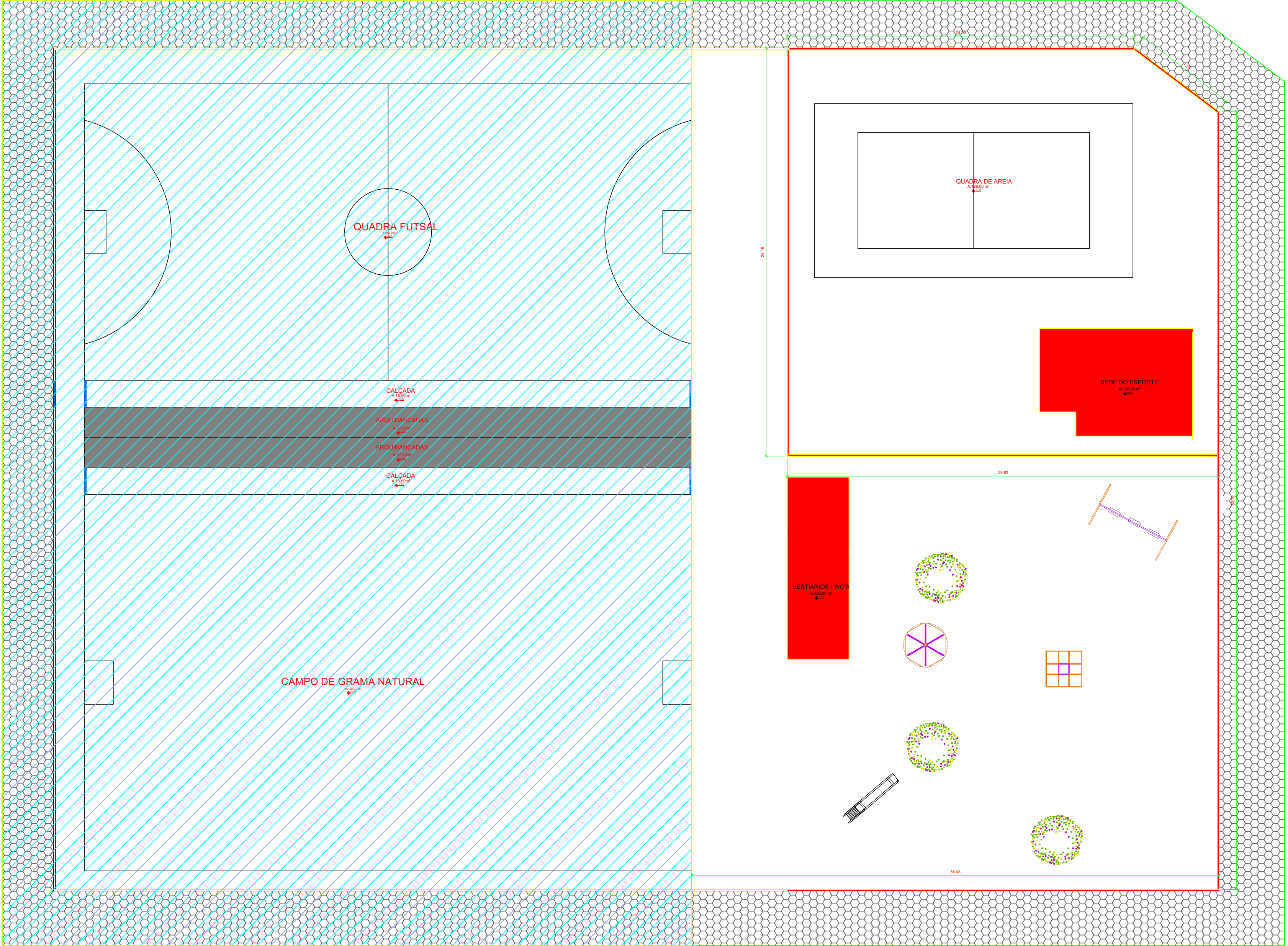
PLANTA DA SITUAÇÃO ATUAL DO COMPLEXO ESPORTIVO COM DEMARCAÇÃO DE DEMOLIÇÃO
