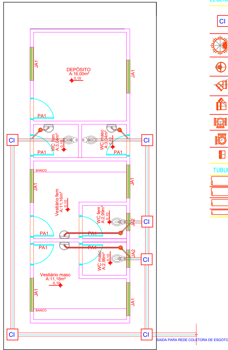
PROJETO SANITÁRIO - VESTIÁRIOS E WC'S ESCALA 1/100
