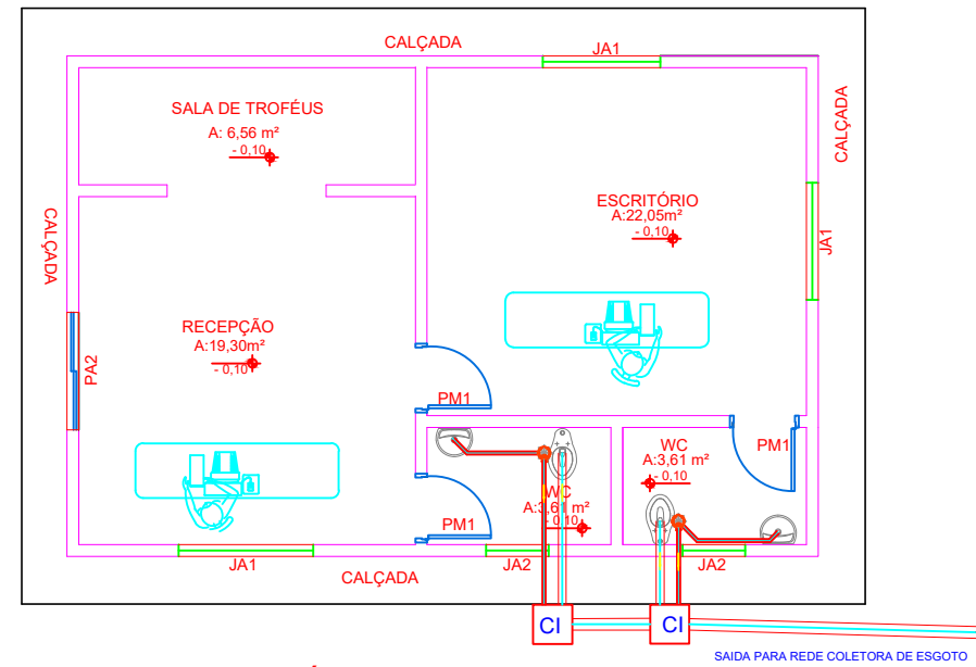
PROJETO SANITÁRIO - SEDE ESPORTE ESCALA 1/100
