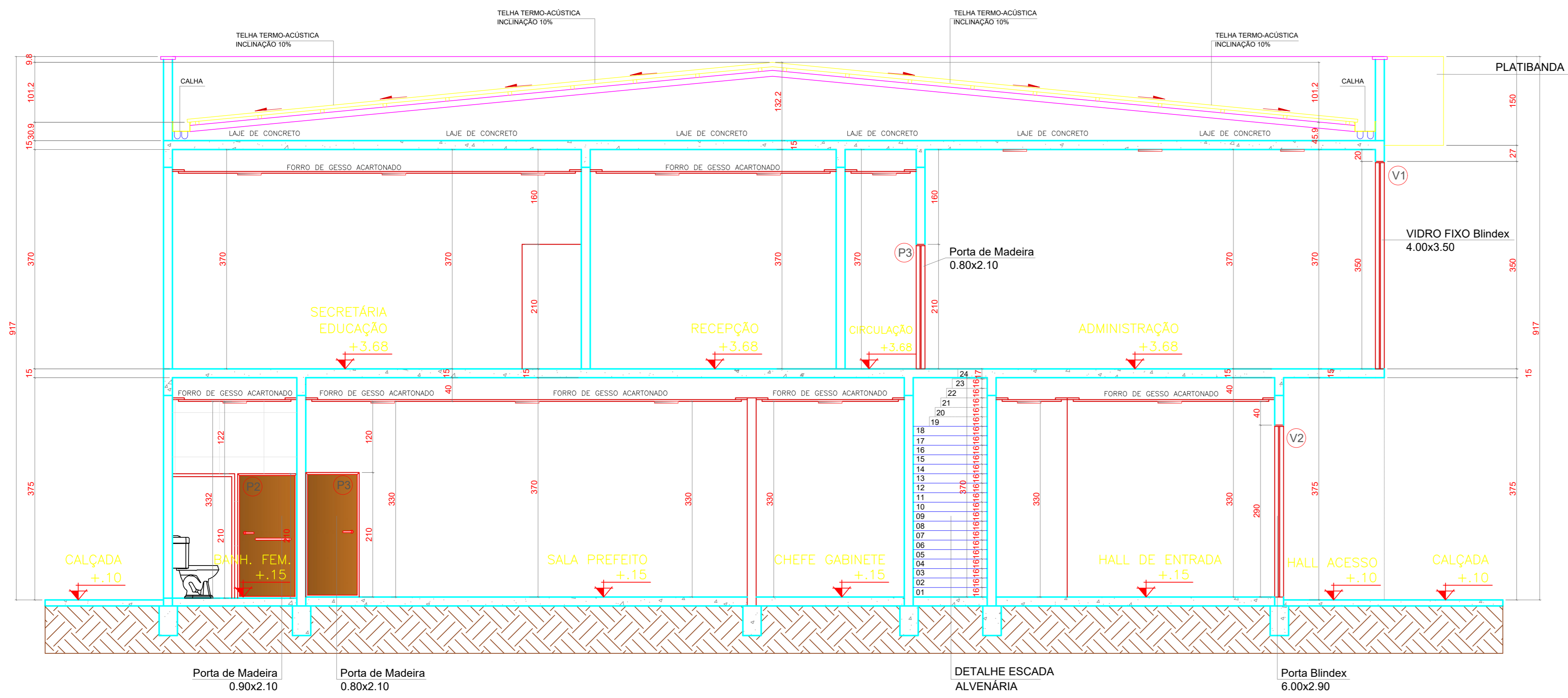
CORTE A-A ESC.: 1:50
