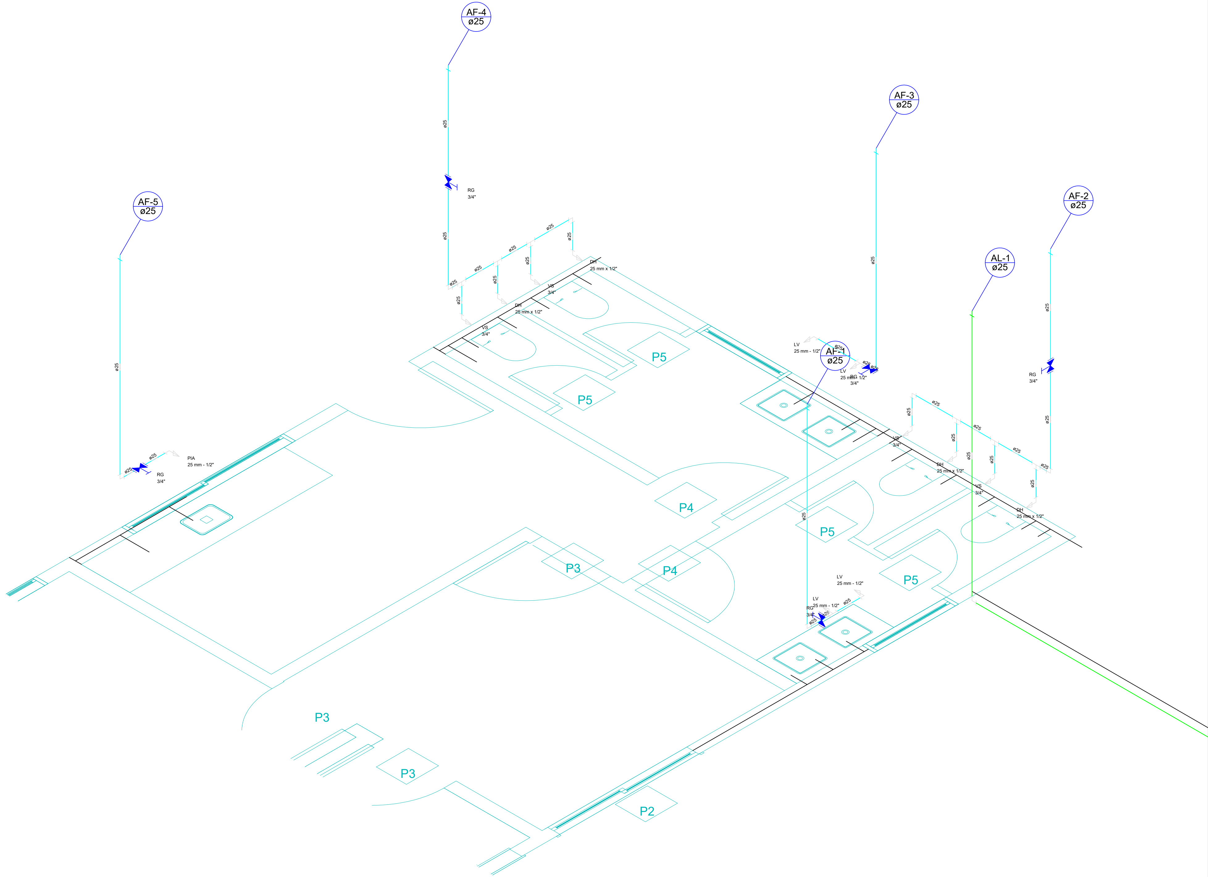
Detalhe H1 escala 1:25
