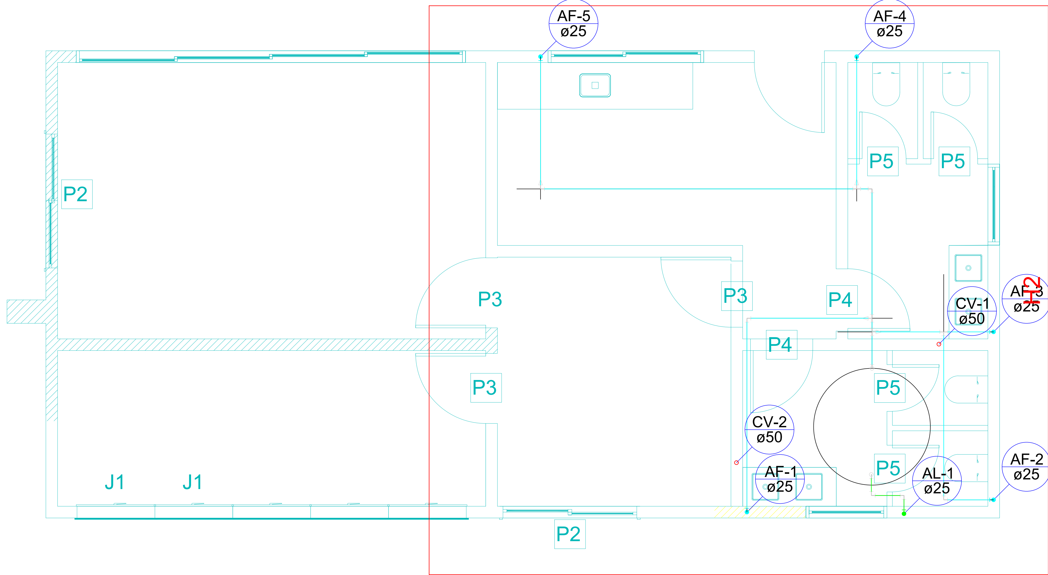
Planta Baixa escala 1:25
