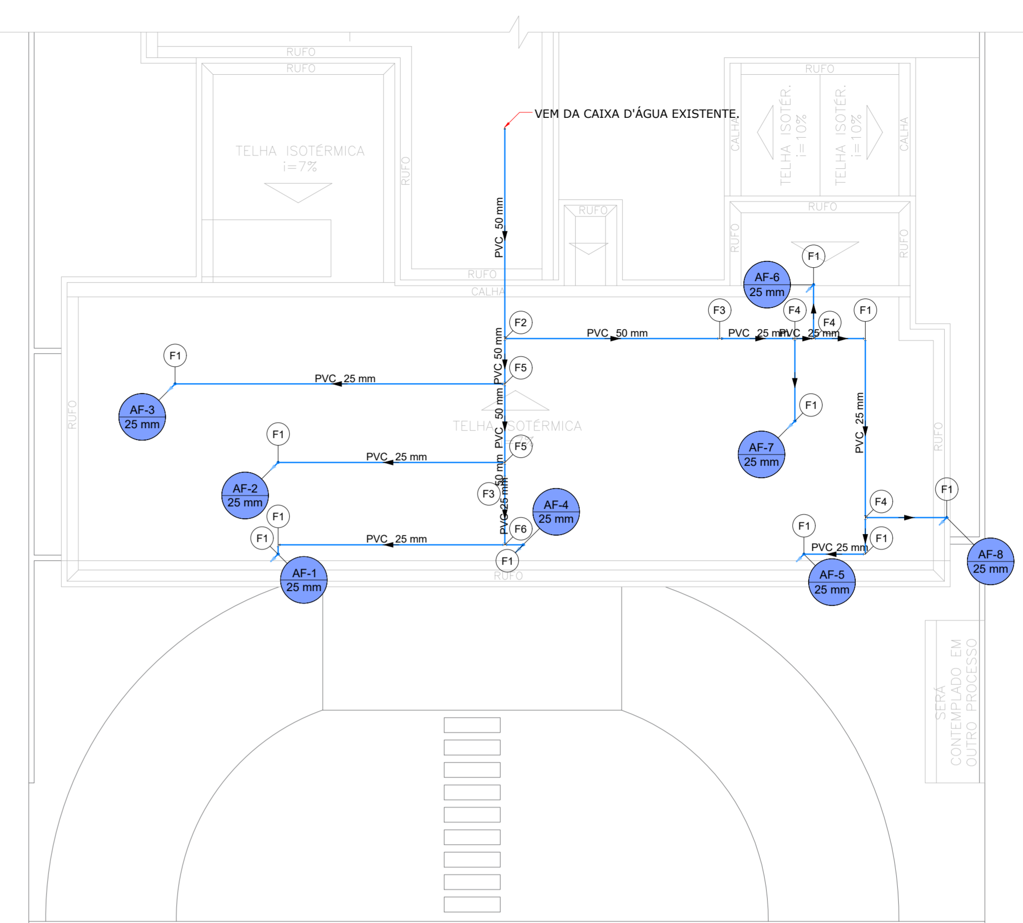
HIDRÁULICO - COBERTURA Escala 1:100
