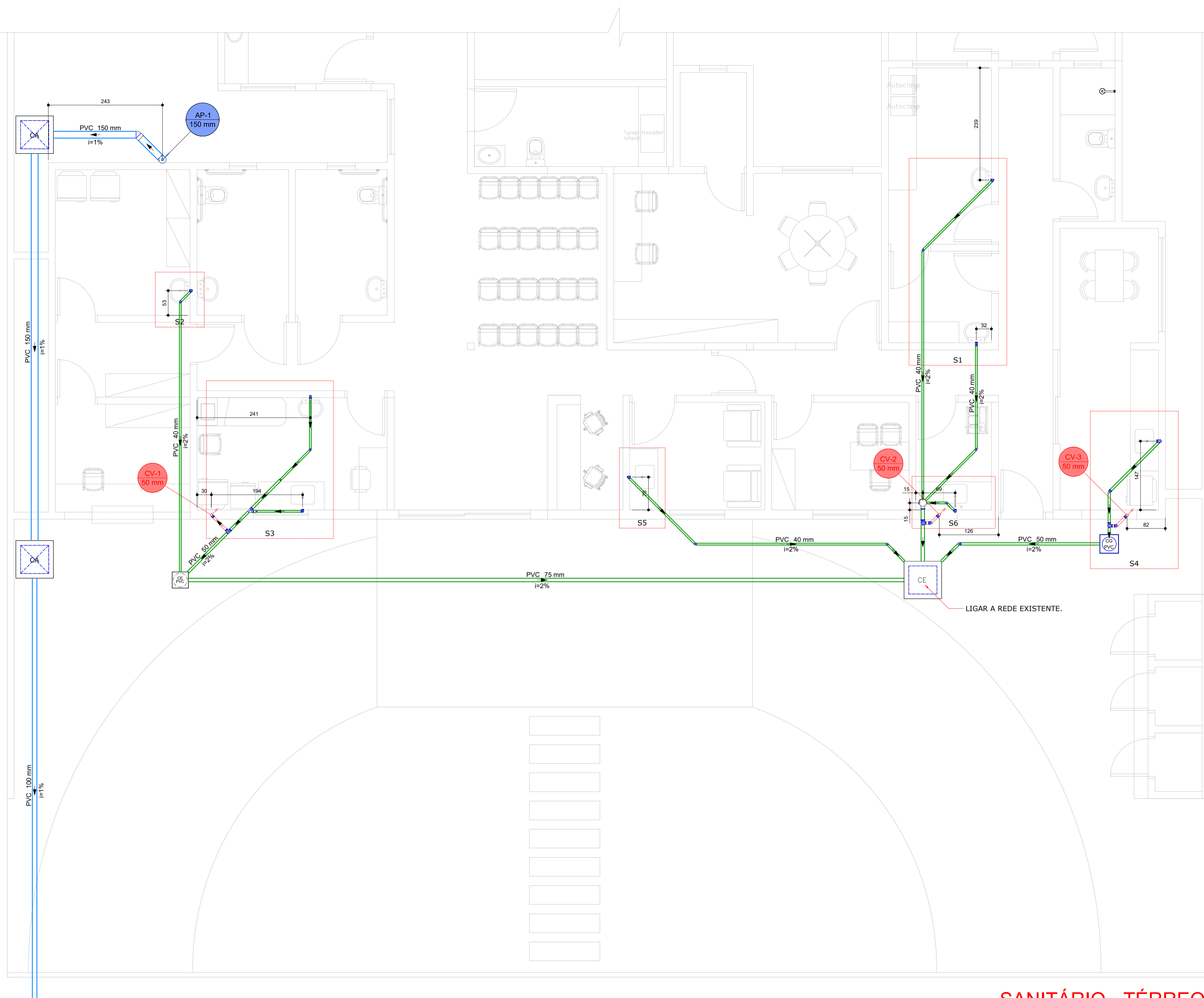
SANITÁRIO - TÉRREO Escala 1:50
