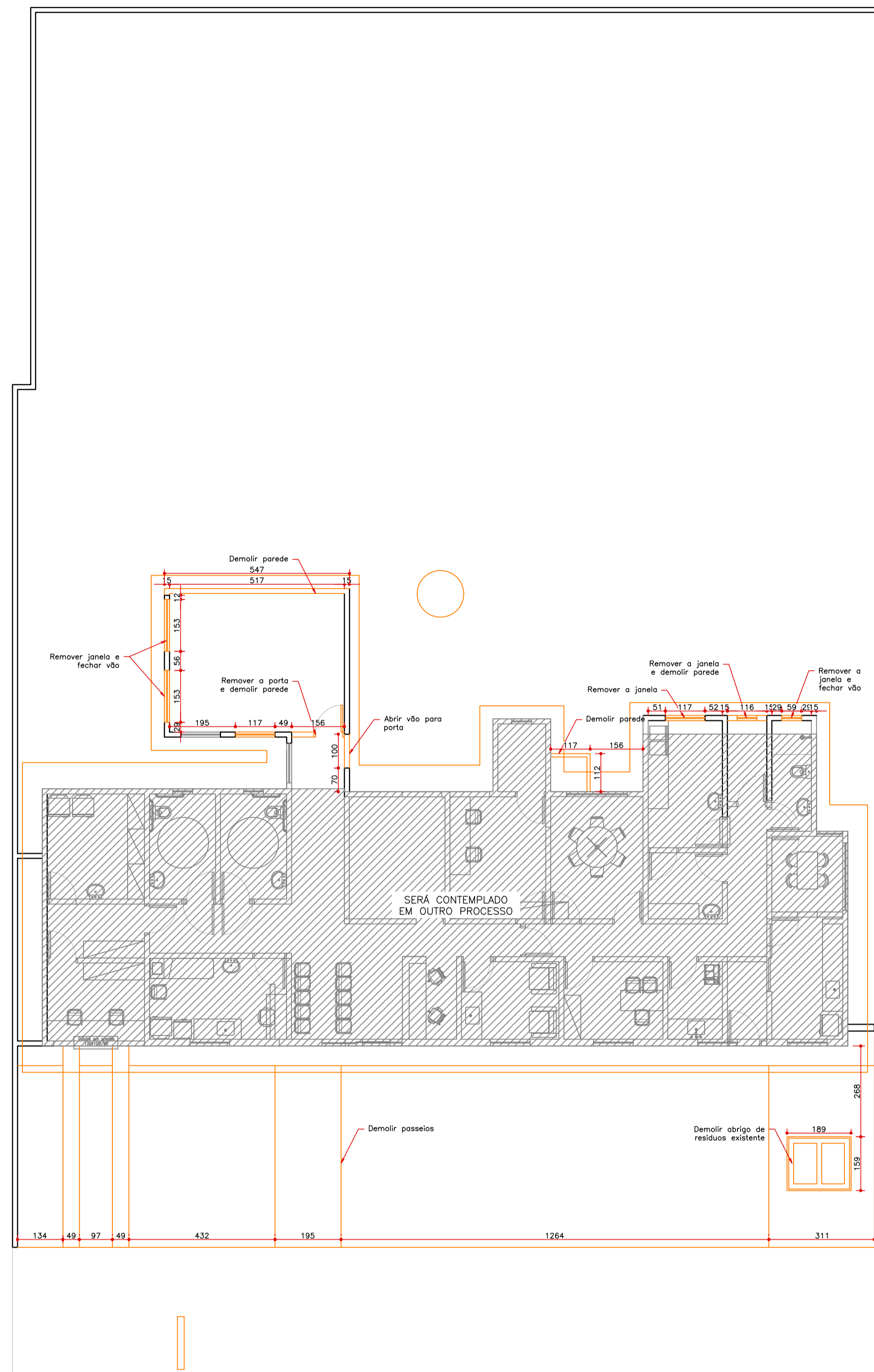
PLANTA BAIXA DEM/CONST 1/75
