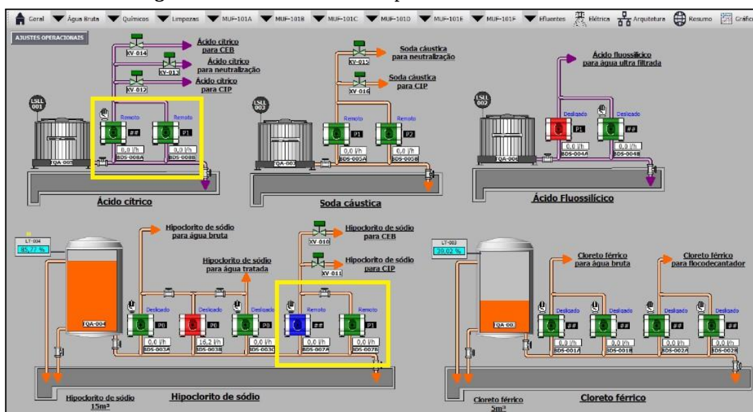
Figura 1 – Bombas vistas no supervisório da ETA Cristo Rei
