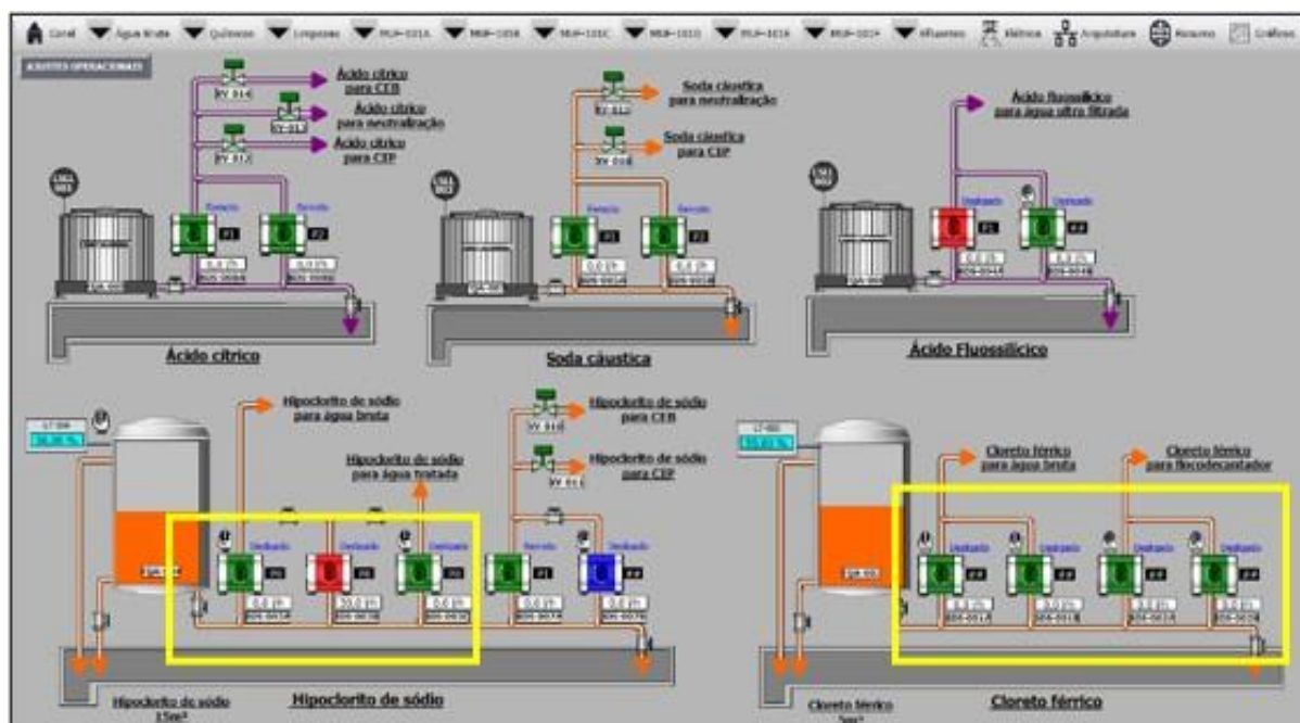
Figura 3 – Bombas dosadoras de diafragma existentes vistas no supervisório da ETA Cristo Rei
