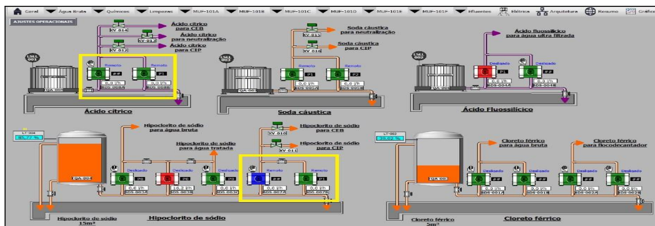
Figura 1 – Bombas vistas no supervisório da ETA Cristo Rei
