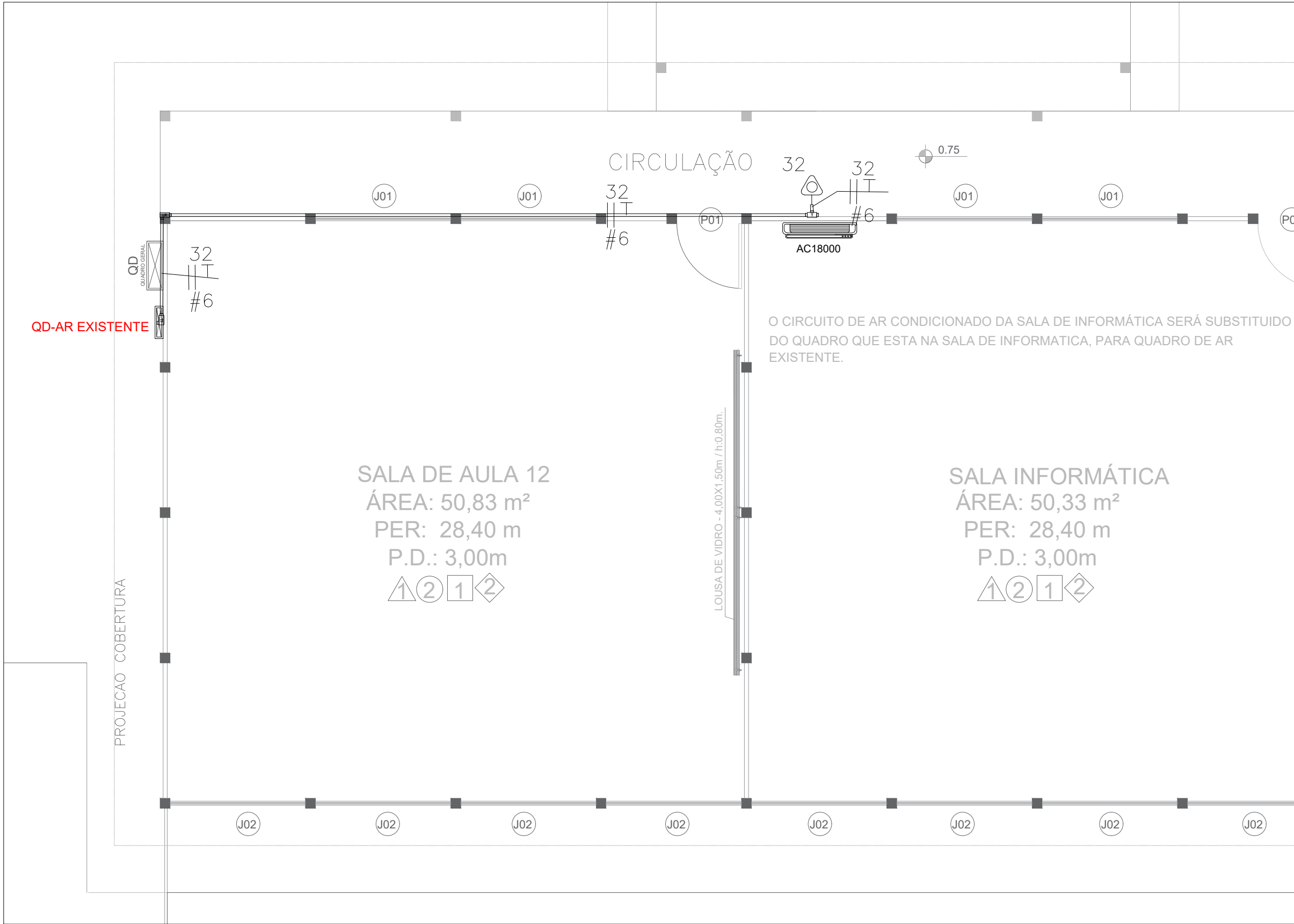
PLANTA AR-CONDICIONADO MUDANÇA DE QUADRO
