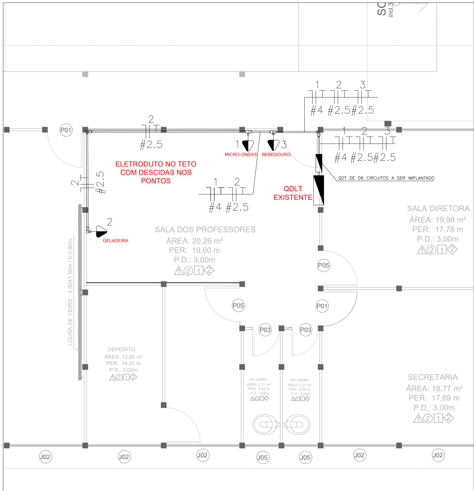
PLANTA SALA DOS PROFESSORES GELADEIRA, BEBEDOURO E MICROONDAS
