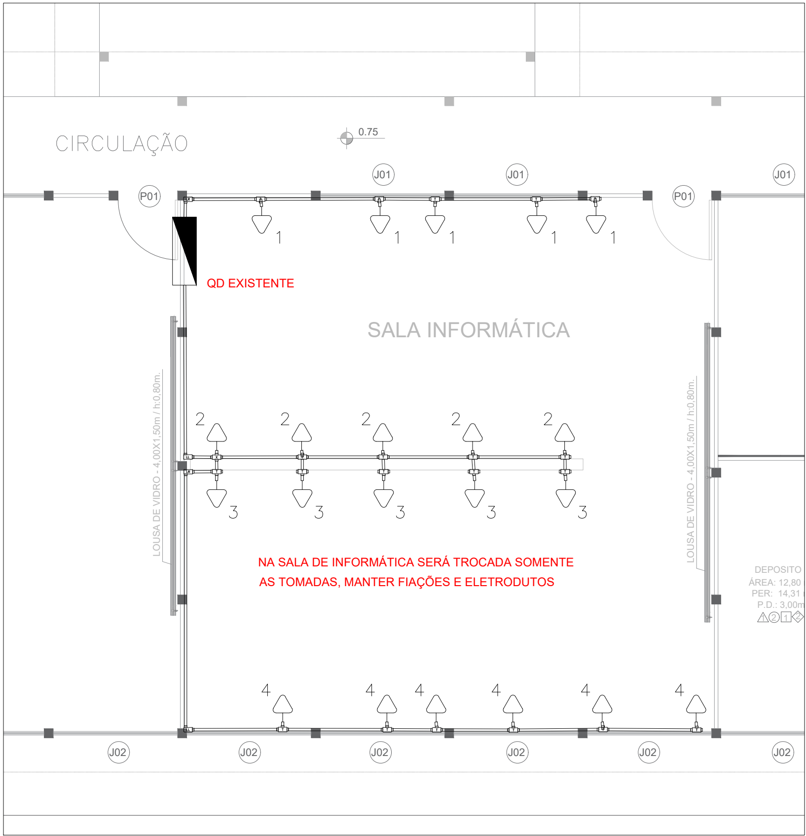
PLANTA TOMADAS MUDANÇA DE CONDULETE
