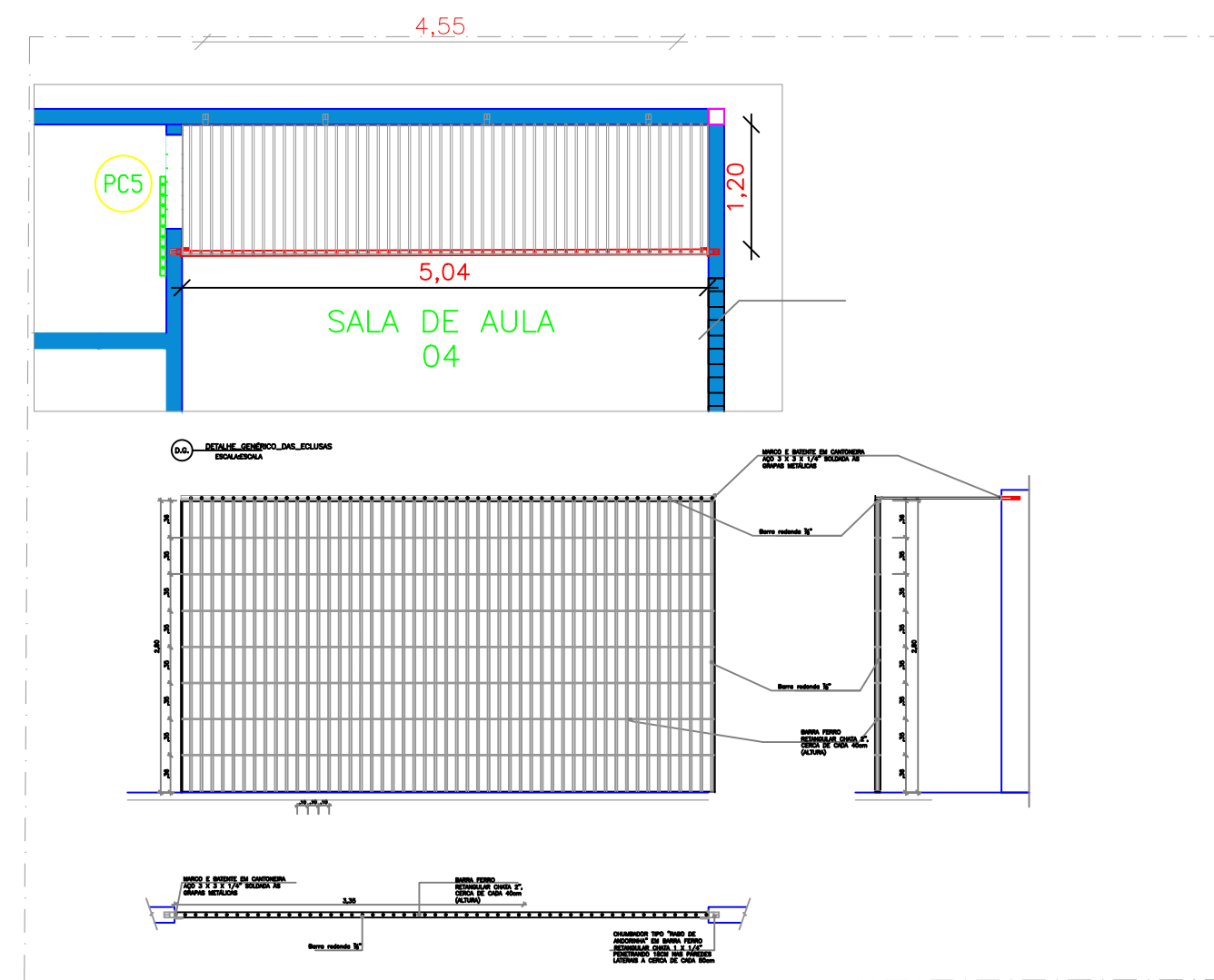
DETALHE 2 - FECHAMENTO SUPERIOR DA ECLUSA ESC.: 1/20
