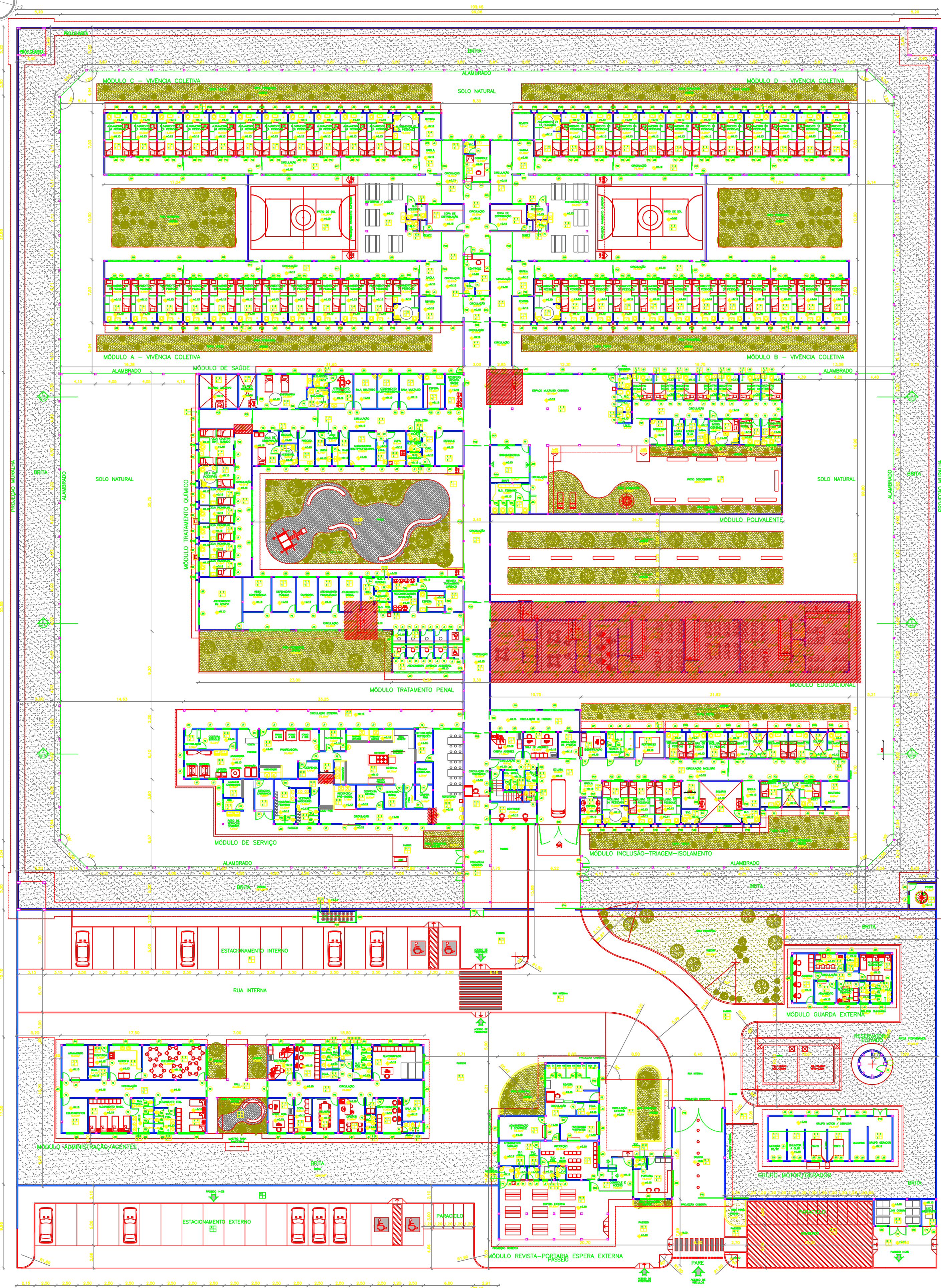
01 PLANTA BAIXA TERREO GERAL - GRADES DE FERRO ESC.: 1/200
