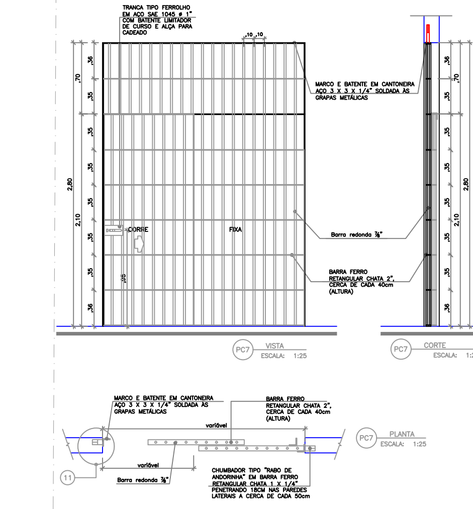
DETALHE DAS GRADES DE FERRO ESC.: 1/20
