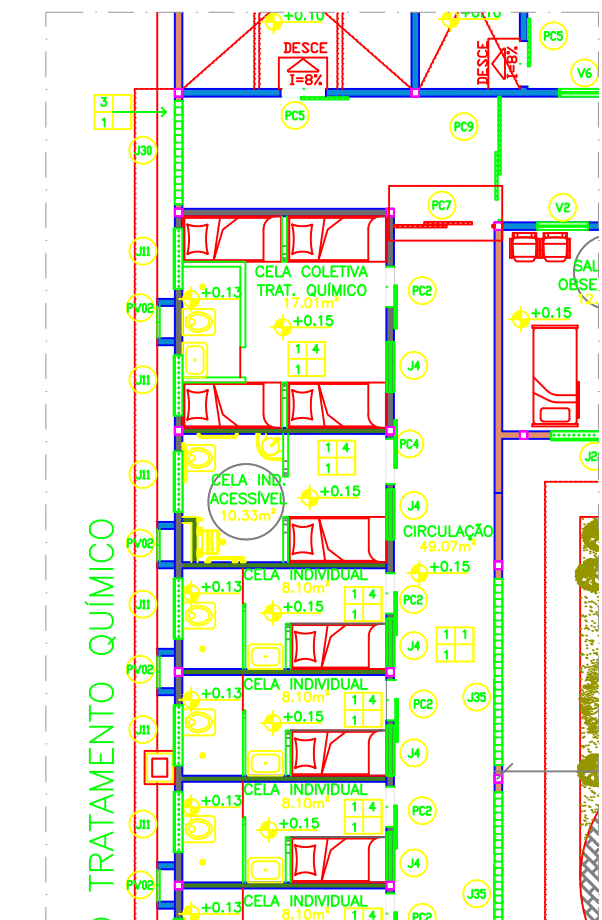
05 PLANTA BAIXA TERREO MÓDULO QUÍMICO - GRADES DE FERRO ESC.: 1/100
