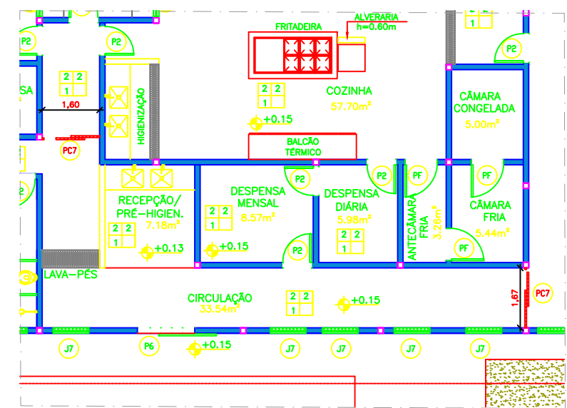
03 PLANTA BAIXA MÓDULO DE SERVIÇOS - GRADES DE FERRO ESC.: 1/100
