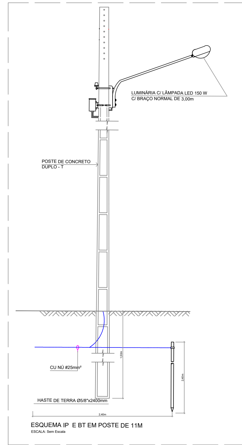
02 POSTE DE ILUMINAÇÃO PÚBLICA S/E
