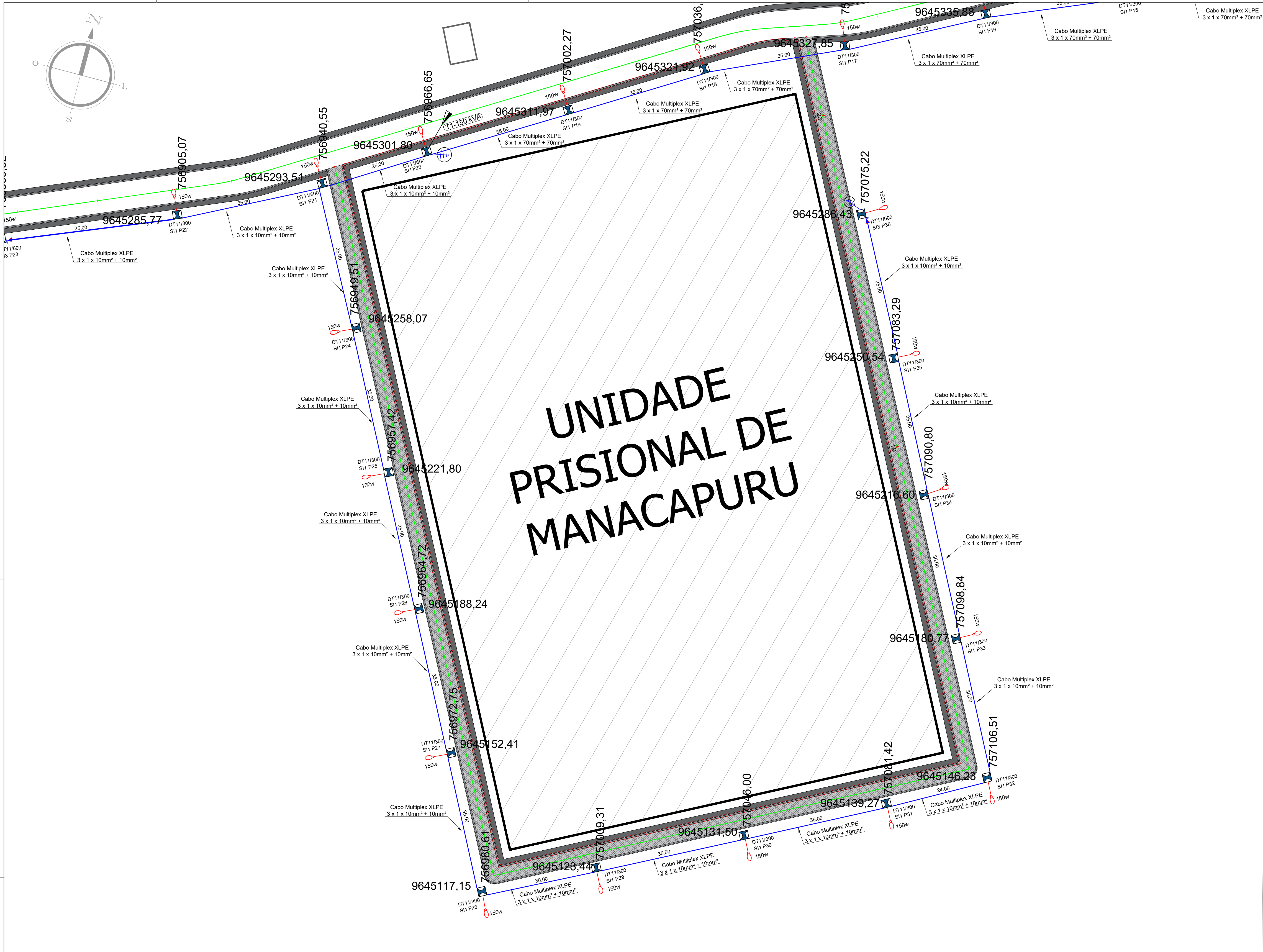
01 IMPLANTAÇÃO ILUMINAÇÃO PÚBLICA VIA DO ENTORNO DO POSTE 24 ESC.: 1/500
