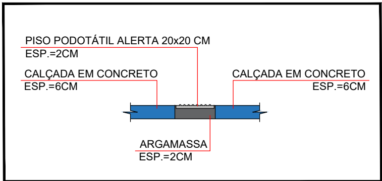
03 DETALHE - FIXAÇÃO DE PISO TÁTIL SEM ESCALA
