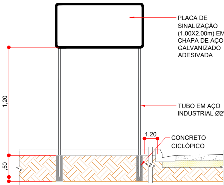
DETALHE - PLACA DE IDENTIFICAÇÃO DE PERÍMETRO E PRÉ-SINALIZAÇÃO SEM ESCALA
