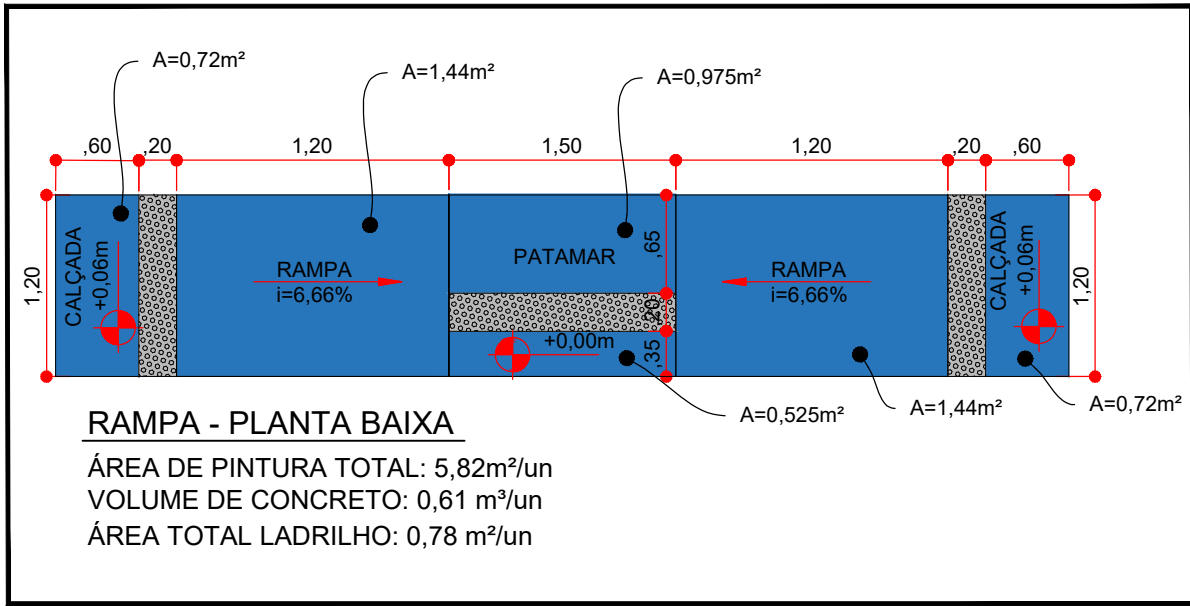
02 DETALHE - RAMPA DE ACESSO ESC.: 1/50
