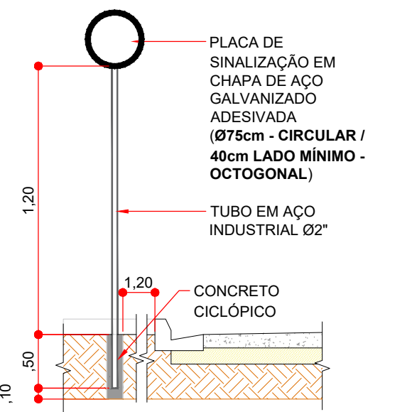
DETALHE - PLACA DE REGULAMENTAÇÃO SEM ESCALA
