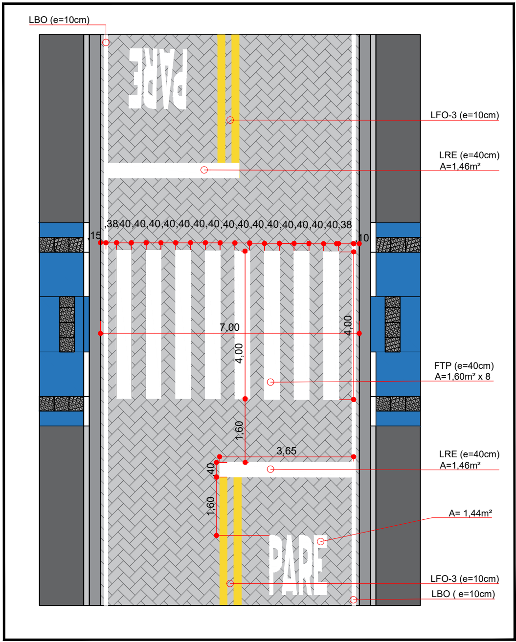
01 DETALHE - Faixa de travessia de pedestre - FTP ESC.: 1/100
