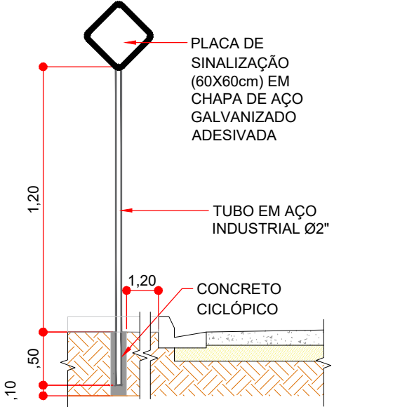
DETALHE - PLACA DE ADVERTÊNCIA SEM ESCALA
