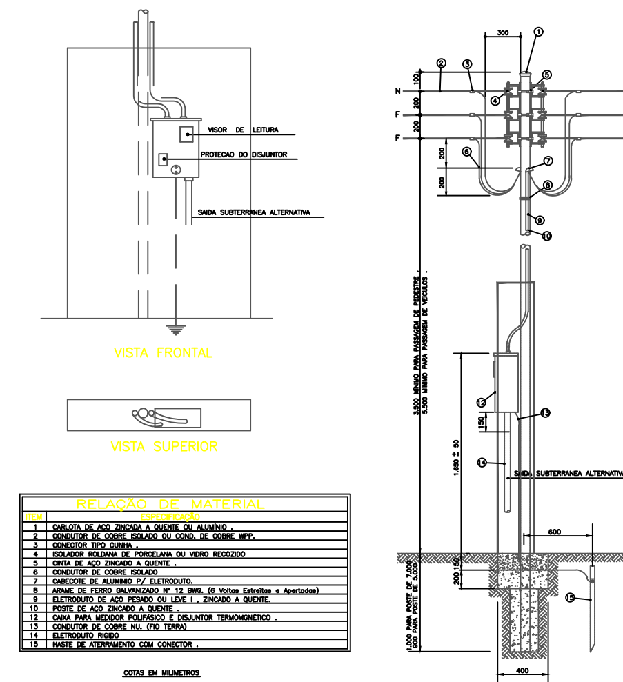
MEDIDOR BIFÁSICO — PADRÃO TIPO CELG INSTALAÇÃO EM MURO OU MURETA SEM ESCALA
