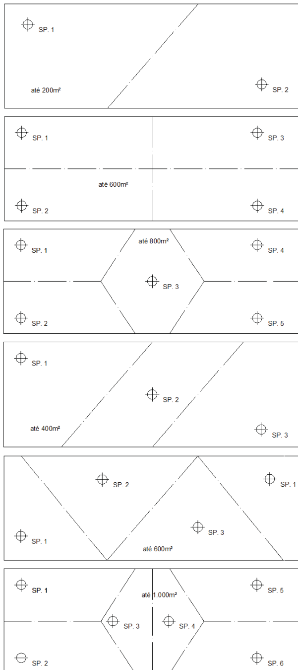
Fig. 02. Disposição recomendada para os furos de sondagem.
