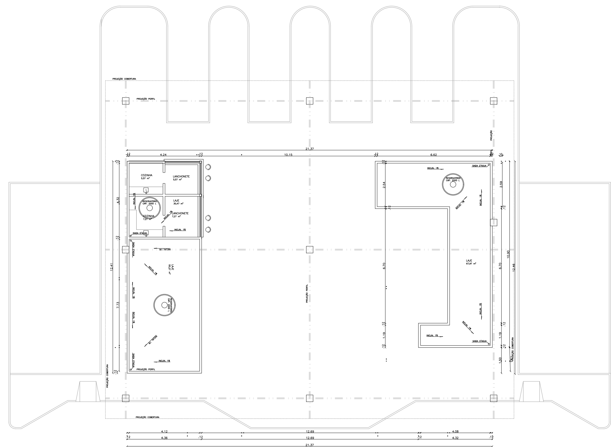
PLANTA BAIXA
