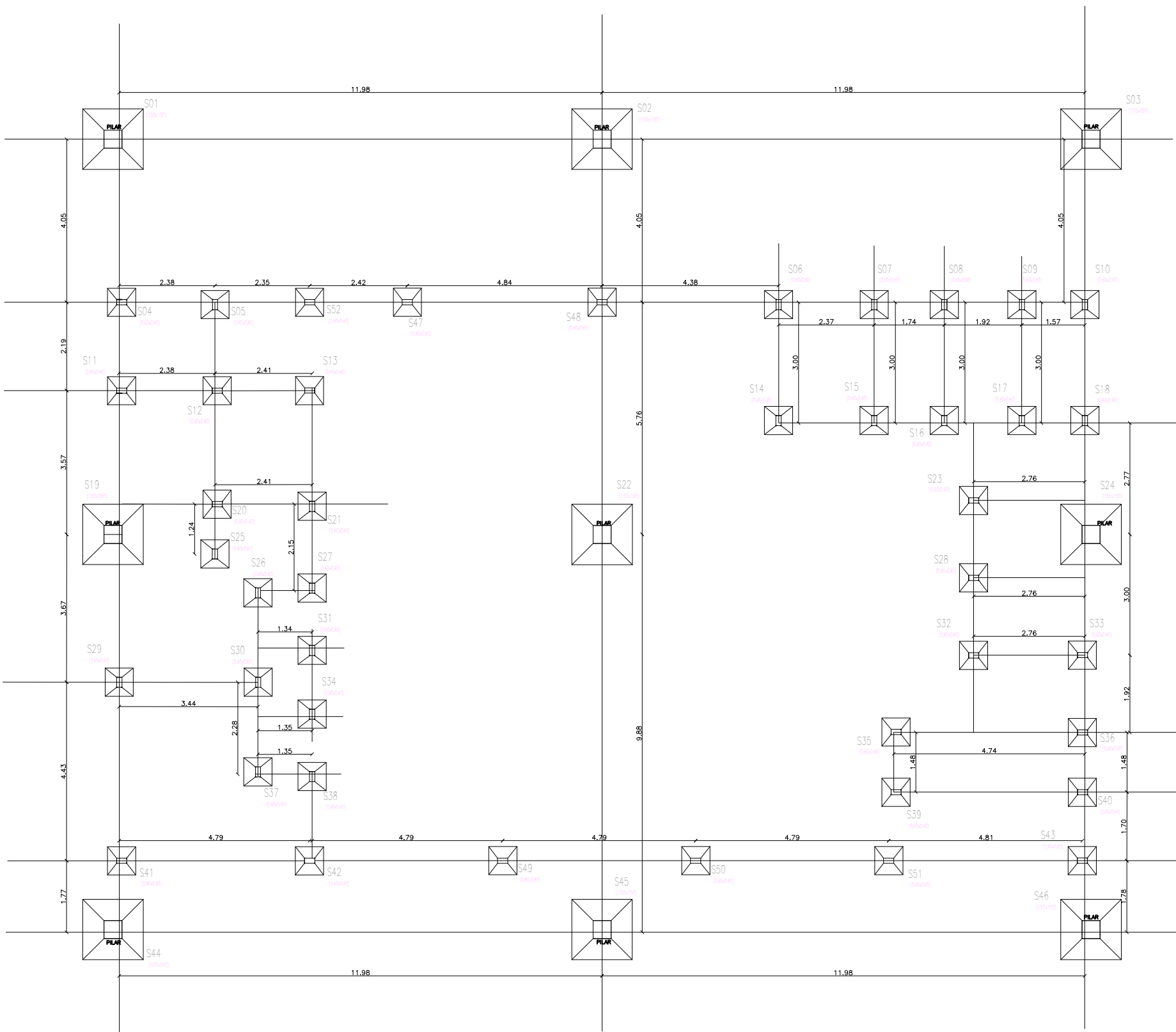
LOCAÇÃO DE SAPATAS E PILARES
