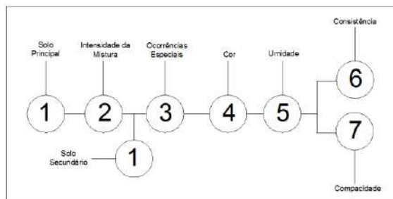
Fig.01 Sequência para Classificação Tátil Visual do Solo.
