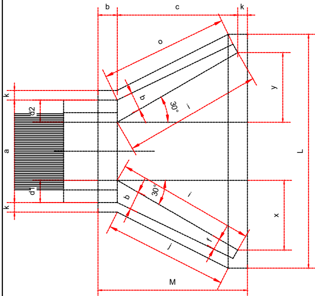
PLANTA NORMAL
