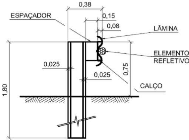
SEÇÃO
