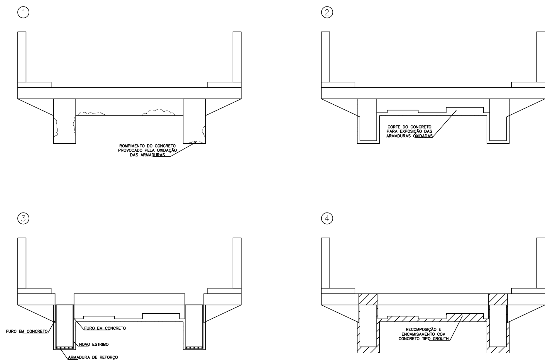
3 DETALHAMENTOS – ESTRUTURAS DE CONCRETO ARMADO SEM ESCALA
