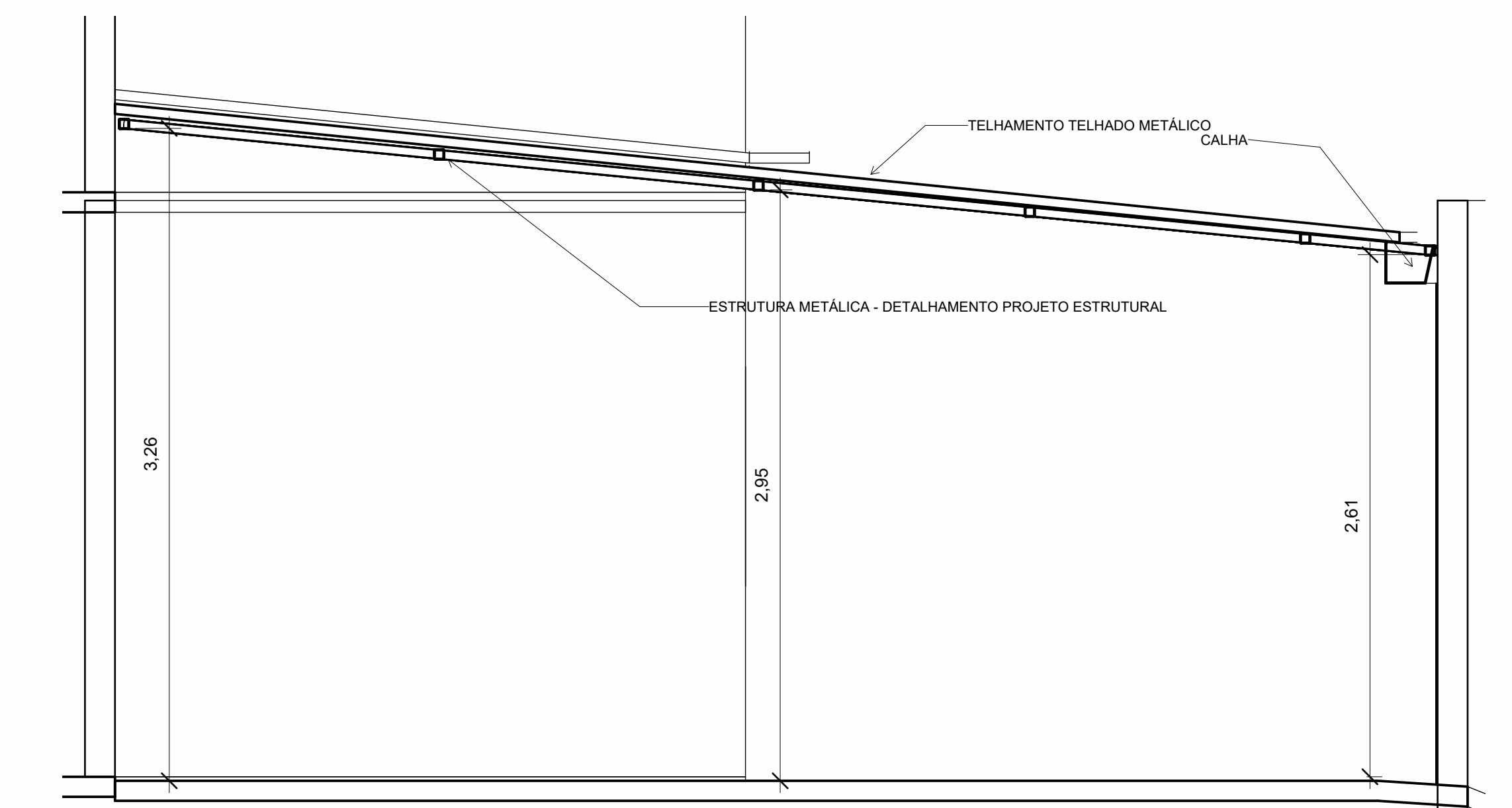
7 CORTE BB 1 : 25
