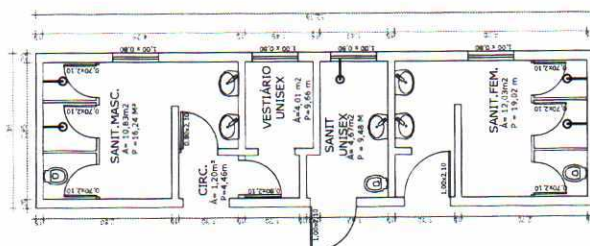
LAYOUT APÓS A REFORMA BANHEIROS QUADRA ESC: 1/75
