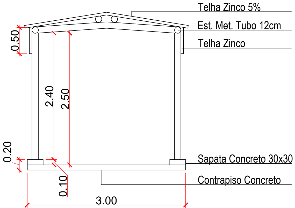
Corte Passarela Acesso Quadra S/ Escala
