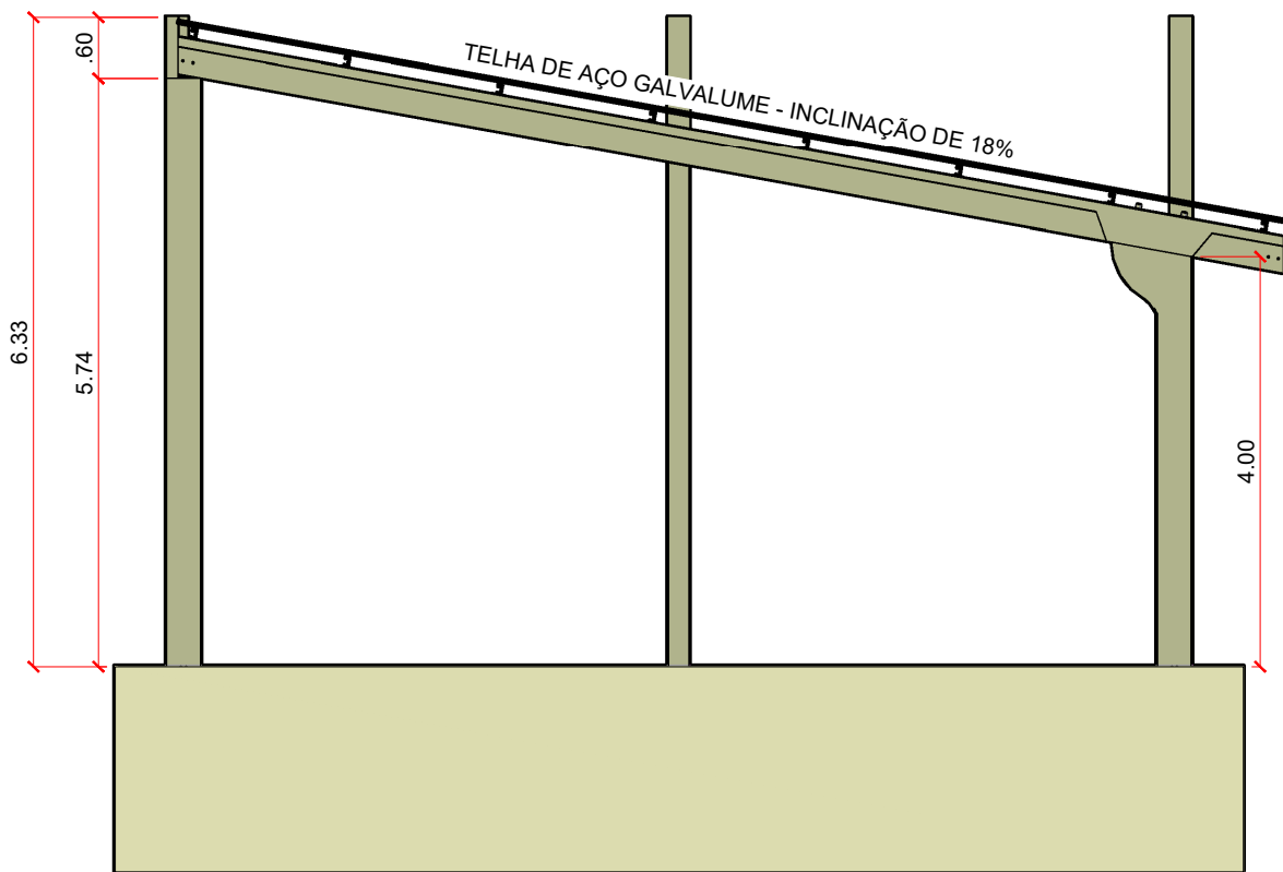
CORTE A-A
