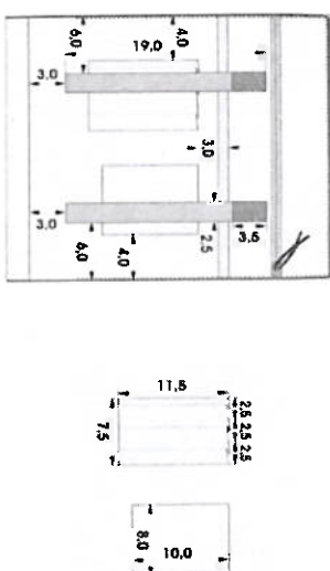
Figura 4 - Medidas e posição das bolsas dentro do bolso grande da frente
