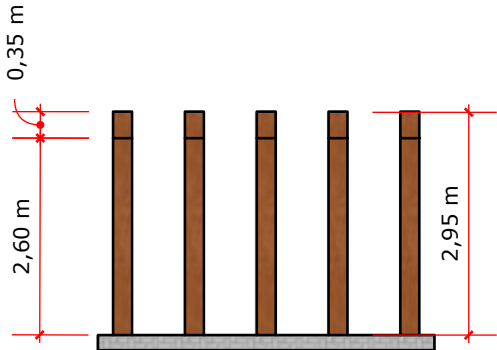
VISTA 3 Escala 1/100
