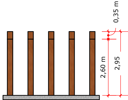
VISTA 2 Escala 1/100
