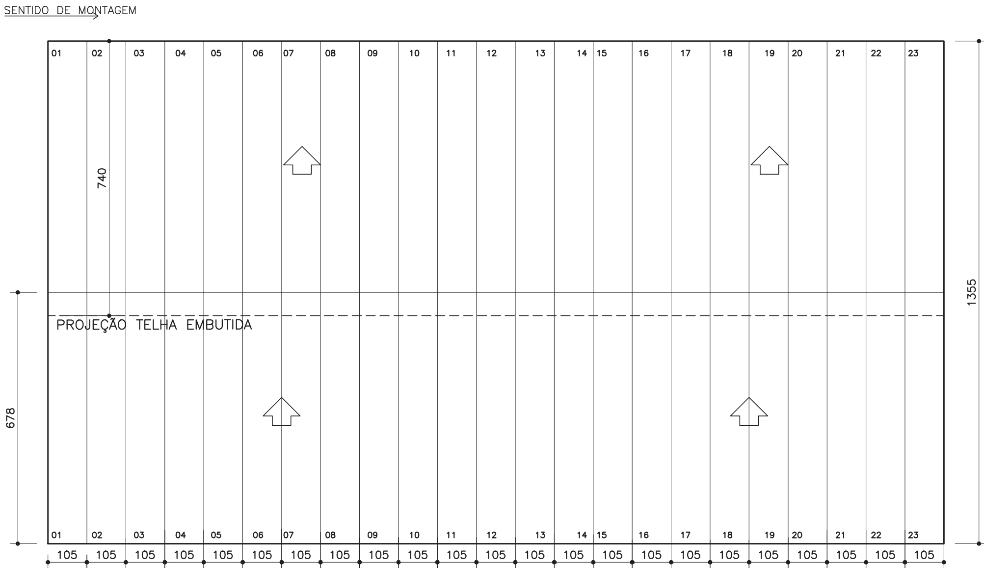
SENTIDO DE MONTAGEM PLANTA AMPLAÇÃO VELÓRIO - NOVA ANDRADINA ESC 1:100
