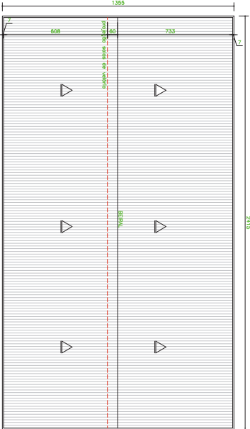
PLANTA COBERTURA – AMPLIAÇÃO VELÓRIO ESC 1/100
