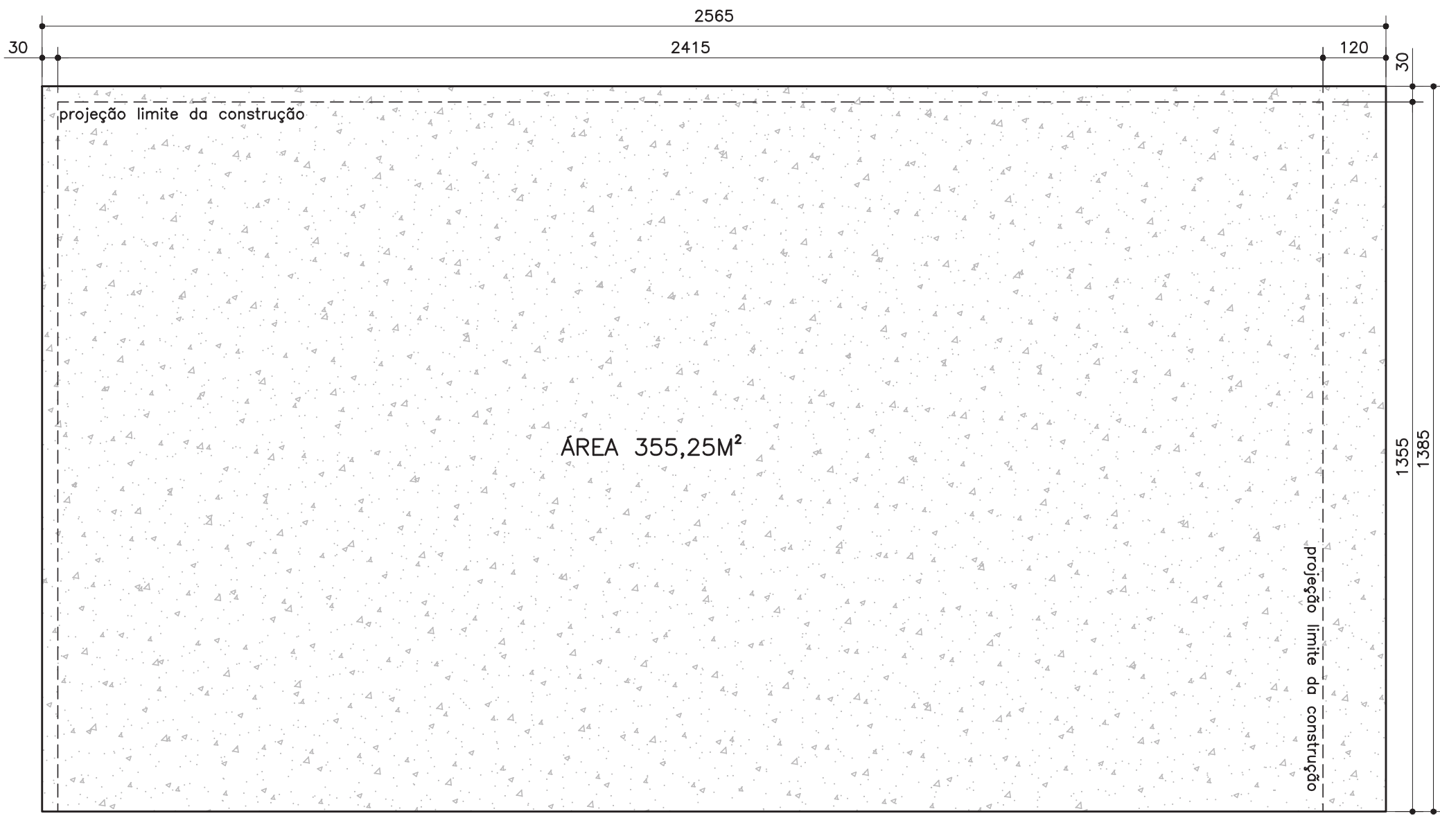
PLANTA DO RADIER ESC 1/100
