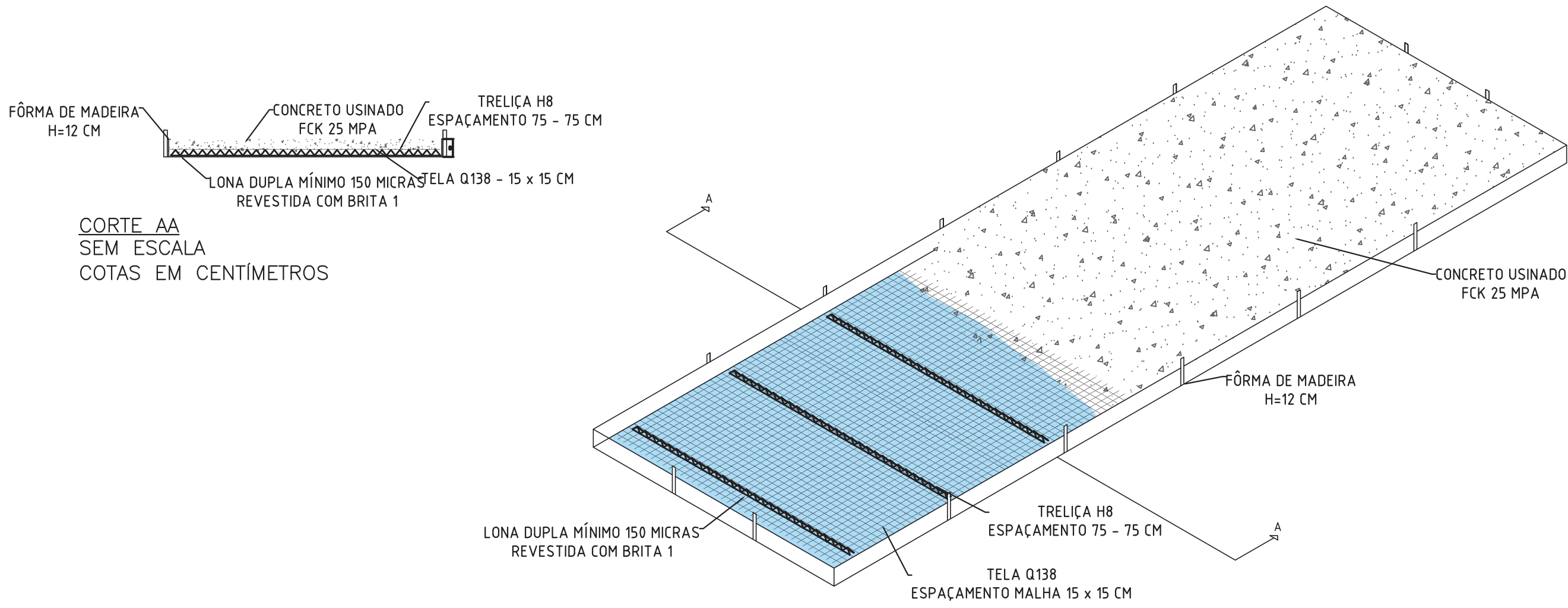
MODELO DE ESPECIFICAÇÕES TÉCNICAS PARA RADIER - VISTA ISOMÉTRICA SEM ESCALA COTAS EM CENTÍMETROS
