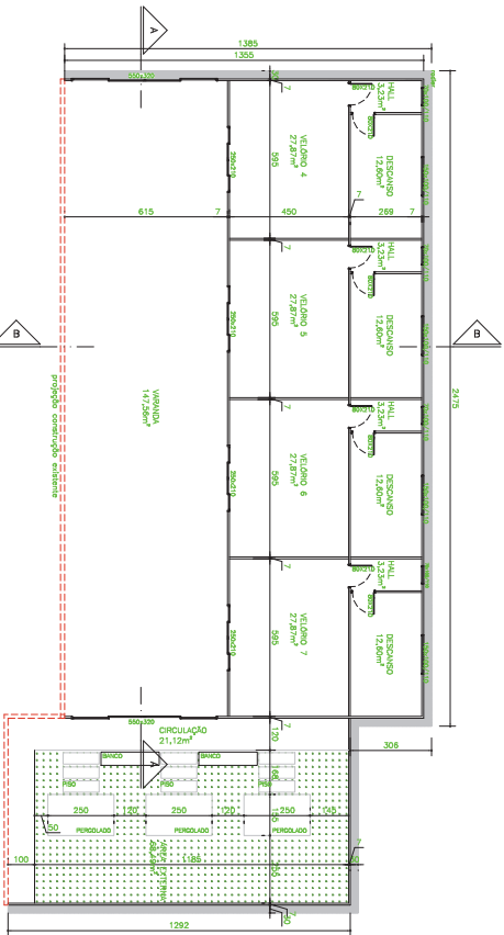
PLANTA BAIXA – AMPLIAÇÃO VELÓRIO ESC 1/100
