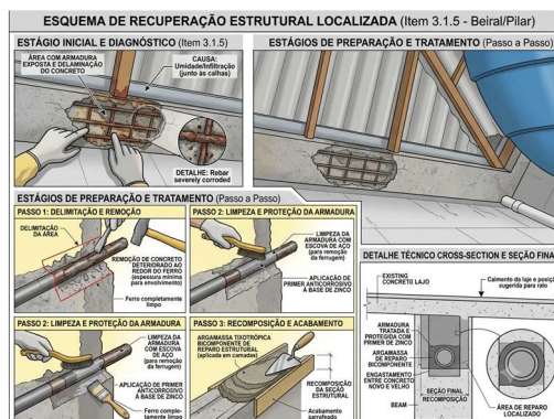
Figura 2 – Esquema sugestivo de intervenção para tratamento recuperação estrutural
