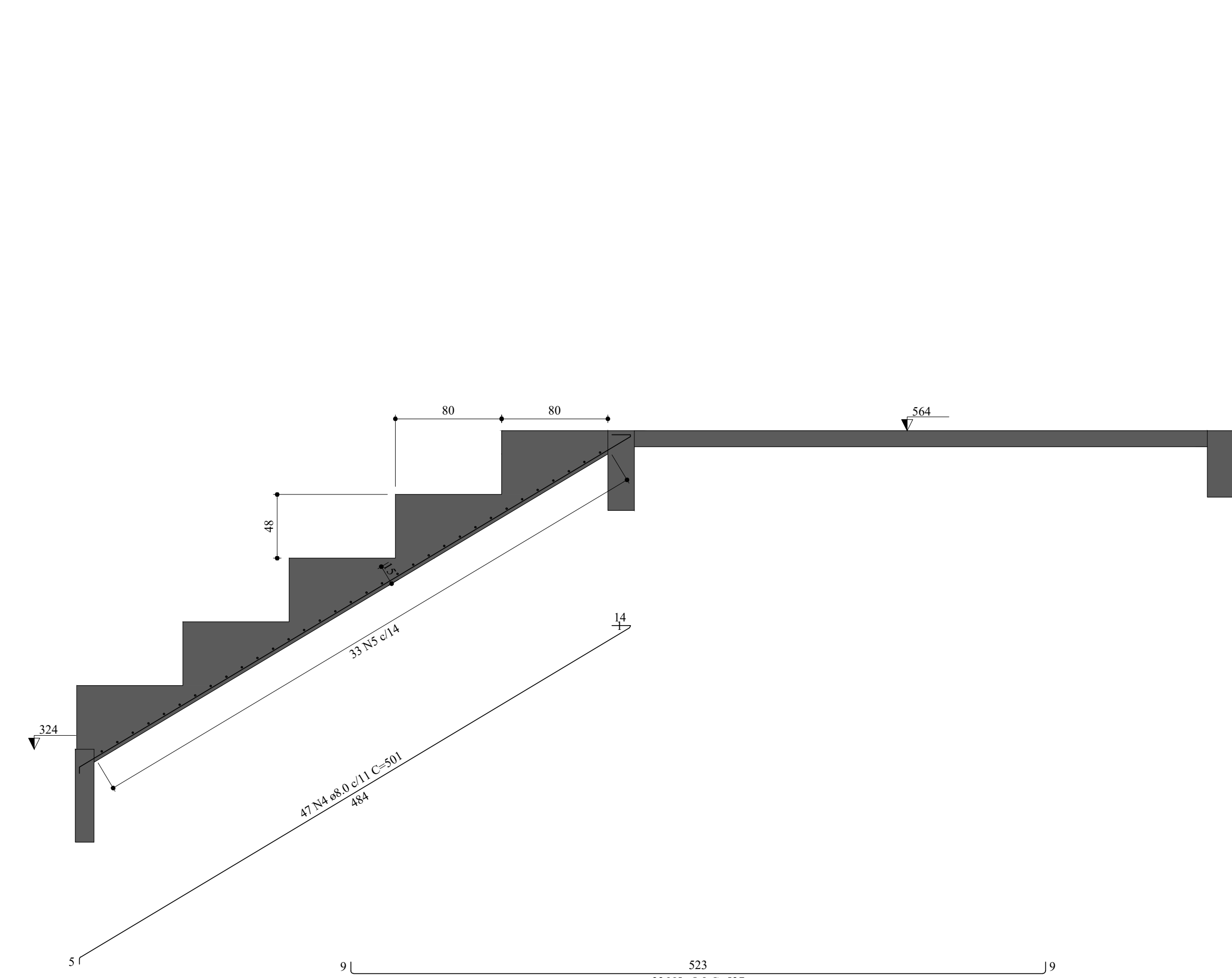
Corte B-B (ARQ7) ESC 1:30
