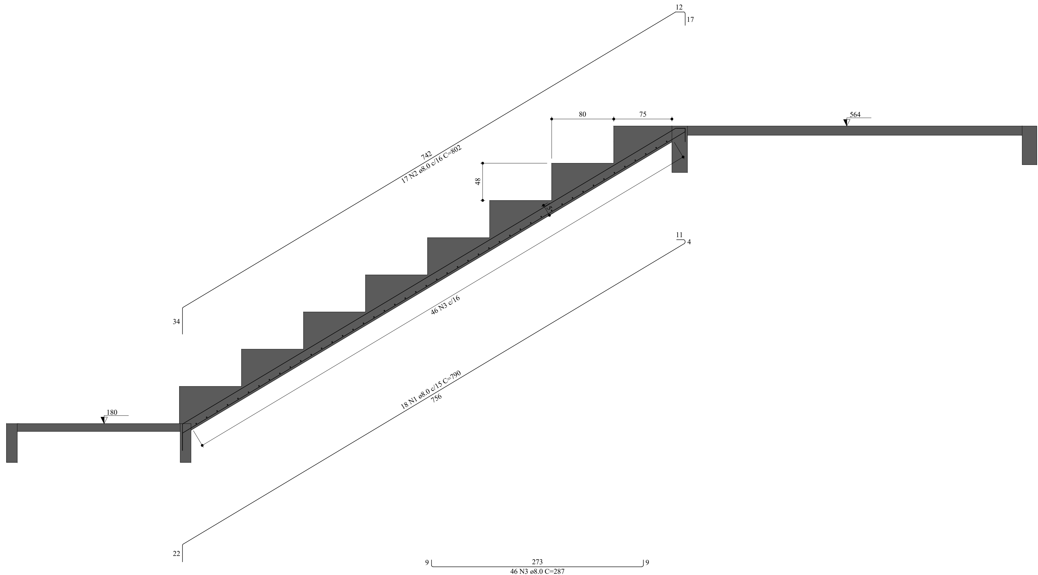
Corte A-A (ARQ6) ESC 1:30
