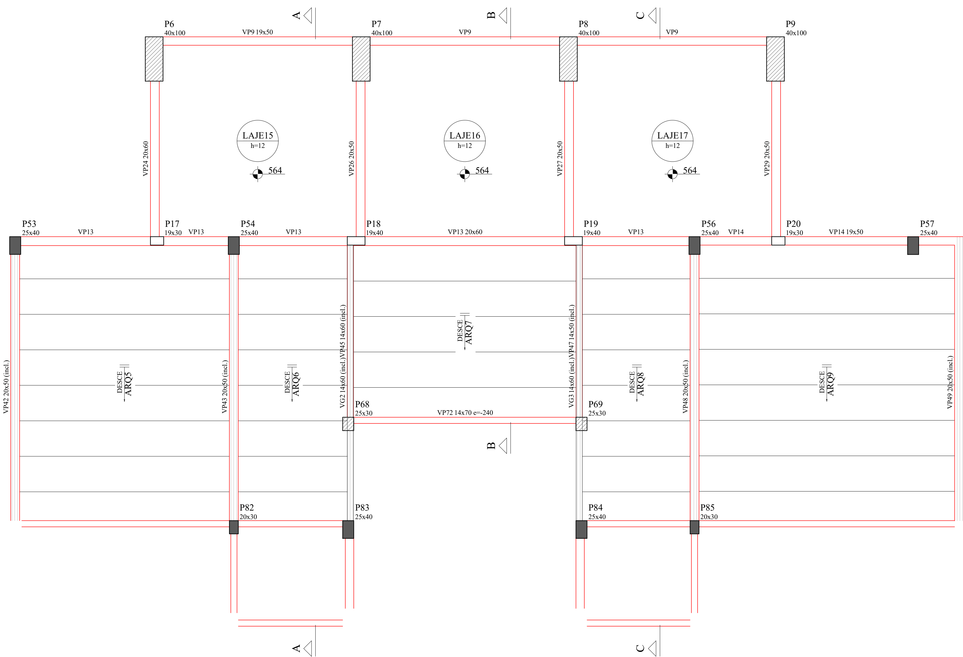
Armação positiva da escada E4 ESC 1:50
