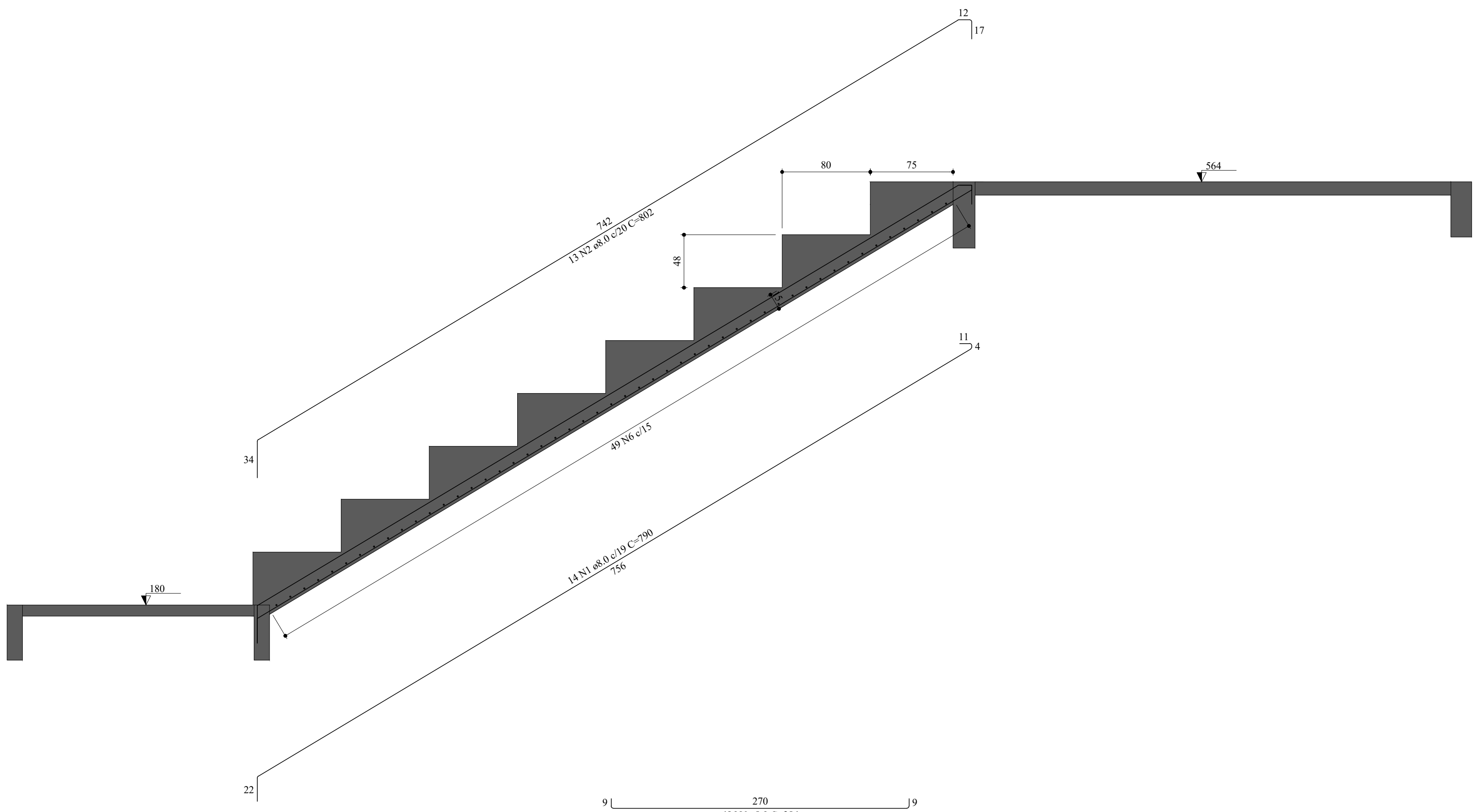
Corte C-C (ARQ8) ESC 1:30
