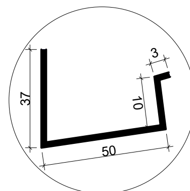
SEÇÃO TRANSVERSAL DA CALHA - 50CM SEM ESCALA
