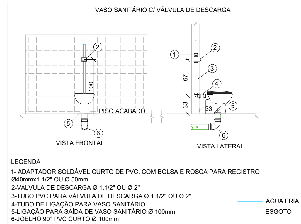
DETALHE INSTALAÇÕES DE APARELHOS SEM ESCALA
