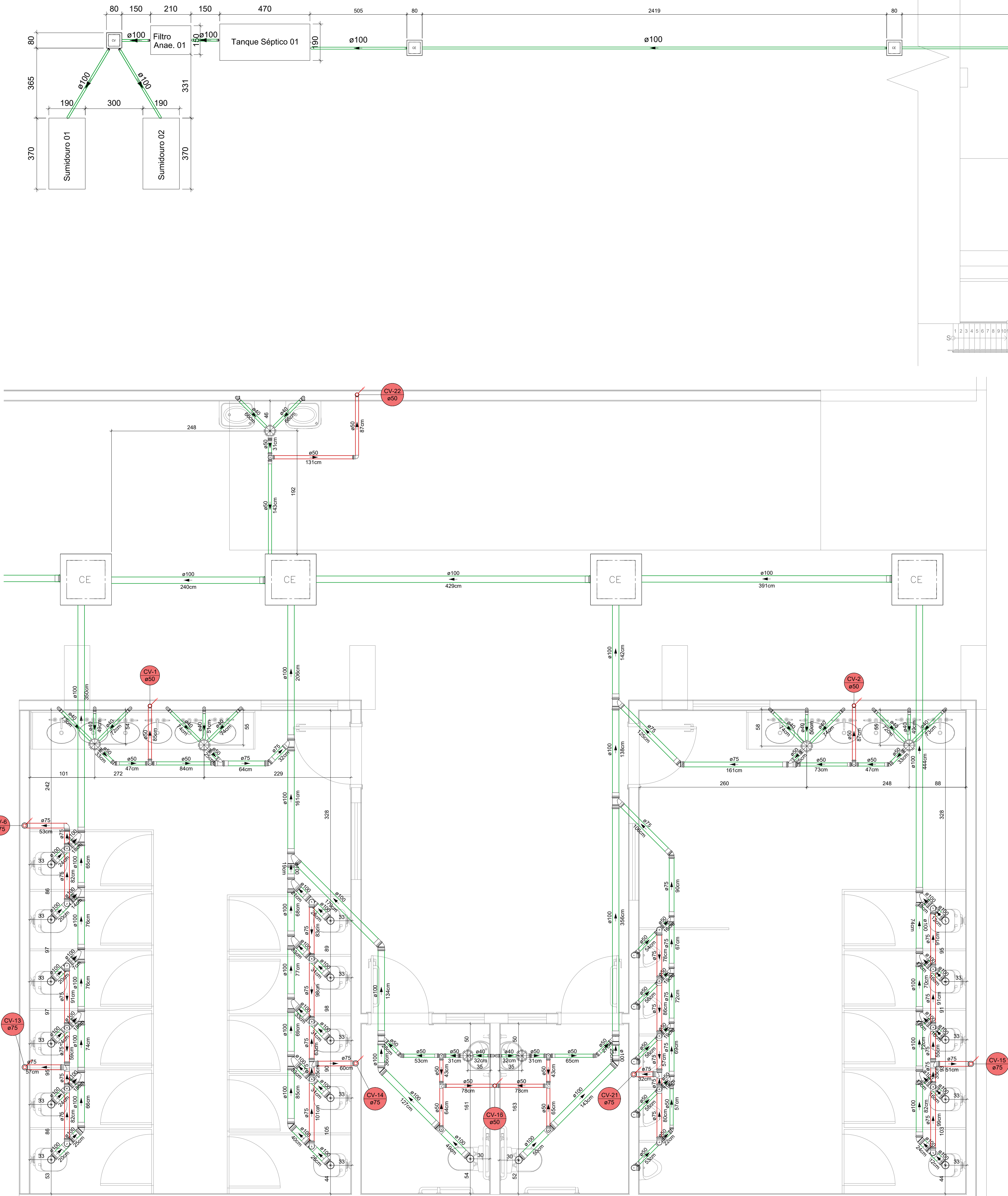
INSTALAÇÕES SANITÁRIAS PLANTA BAIXA ESCALA: 1/100
