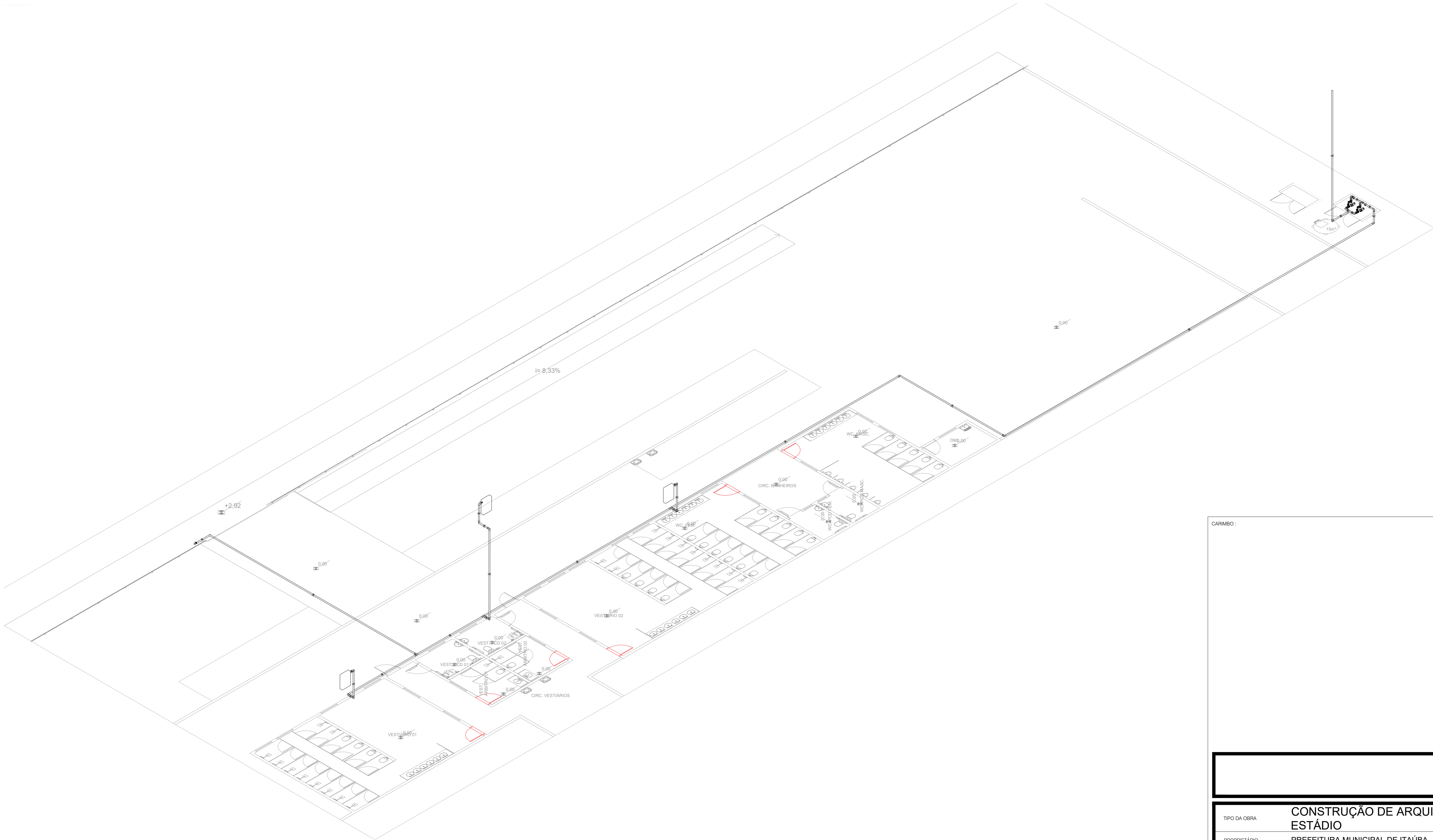
ISOMÉTRICO DOS HIDRANTES SEM ESCALA
