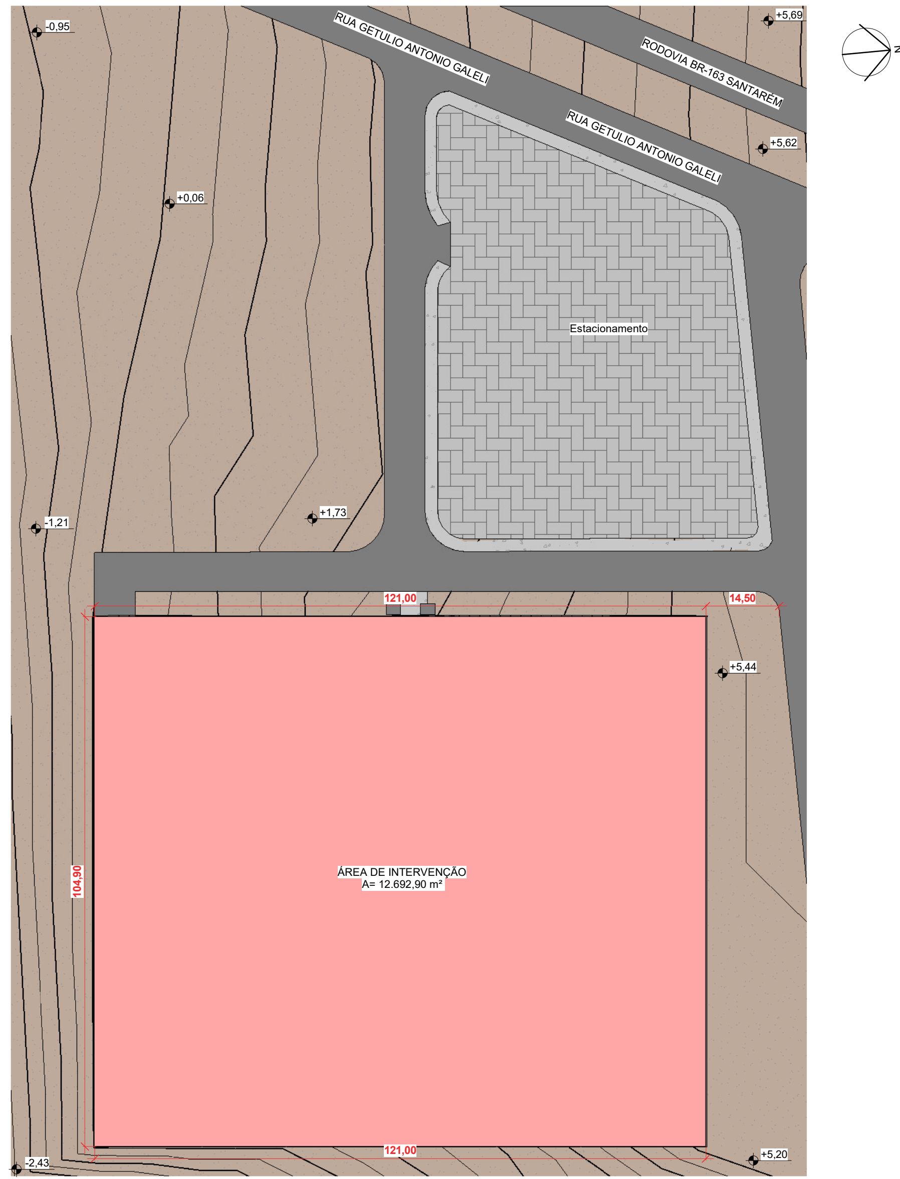
3 Implantação Geral 1 : 750
