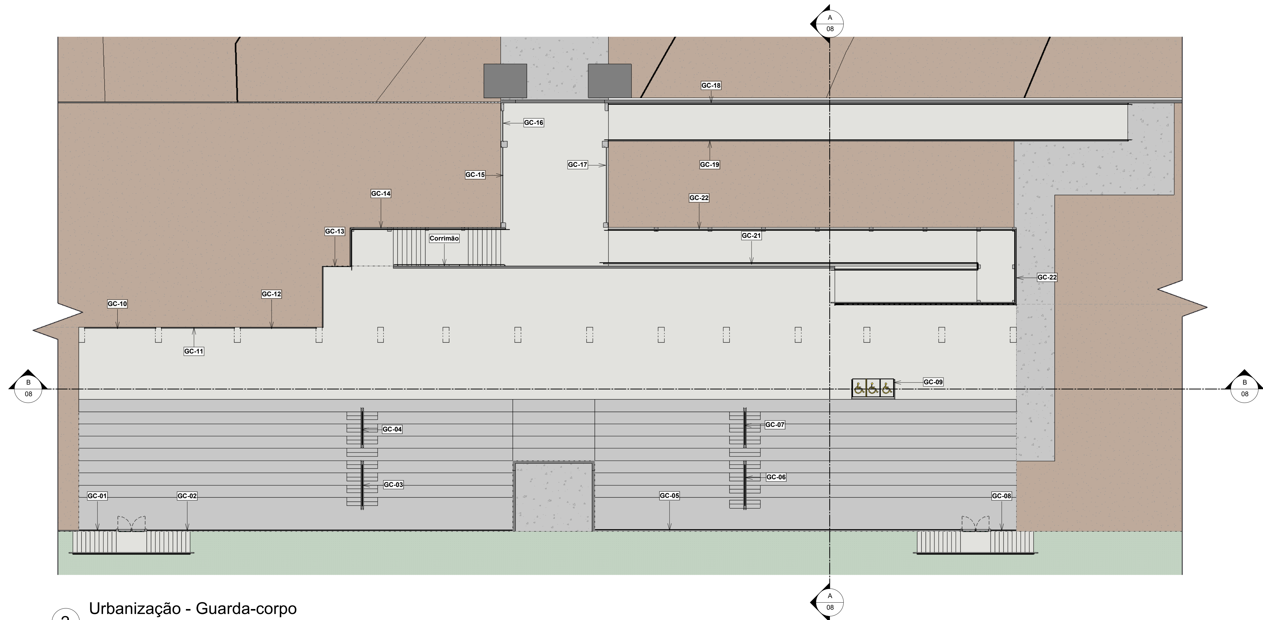
2 Urbanização - Guarda-corpo 1 : 150
